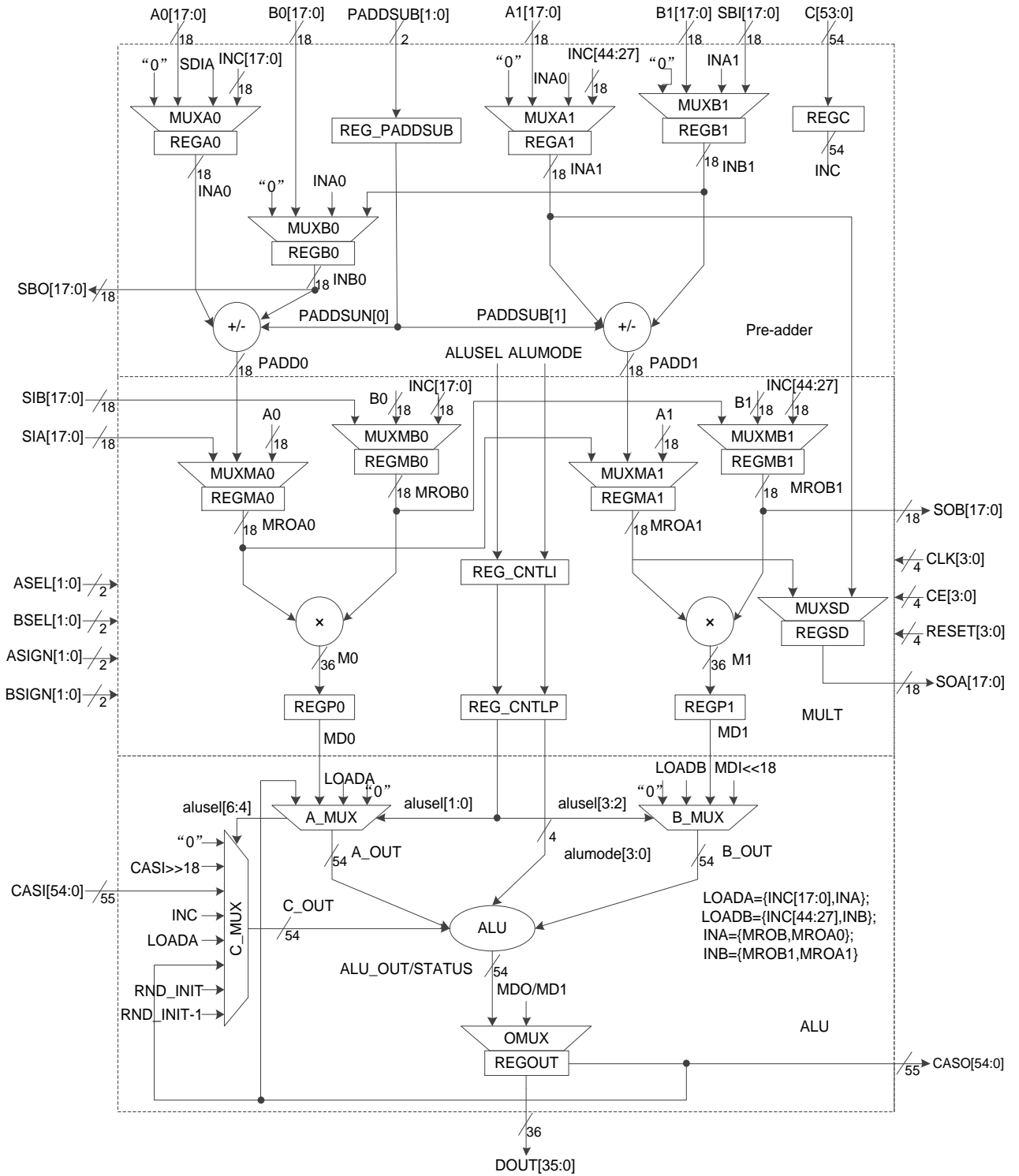
图 3-15 DSP 宏单元
