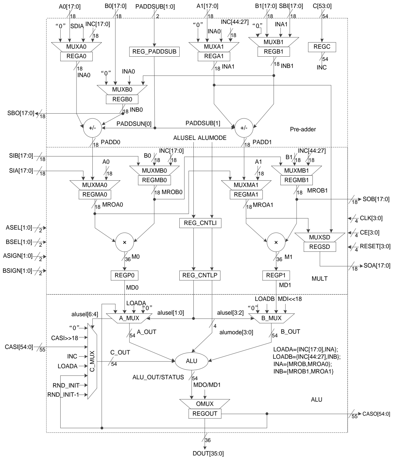
图 3-14 DSP 宏单元
