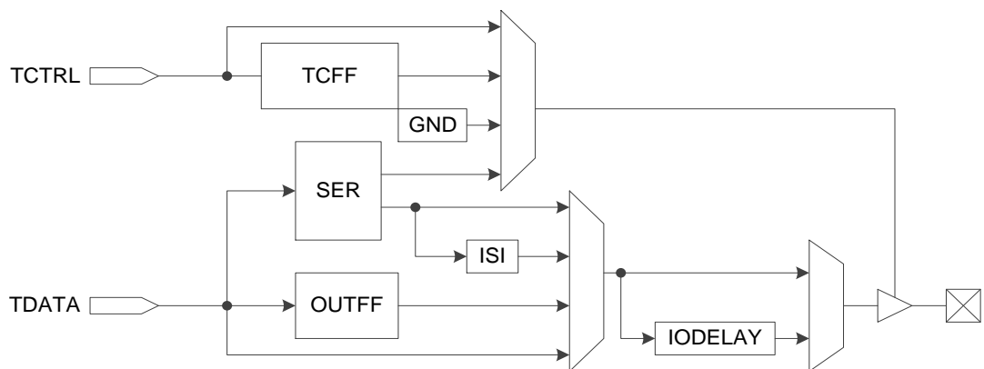
图 3-5 I/O 逻辑输出示意图
