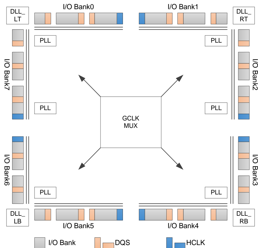
图 3-15 GW2A 时钟资源
