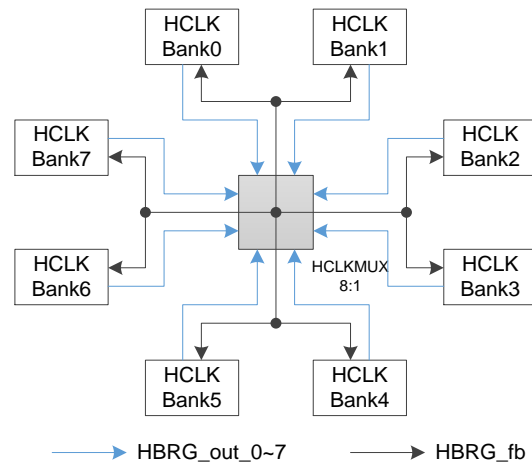
图 3-22 GW2A HCLK 示意图
