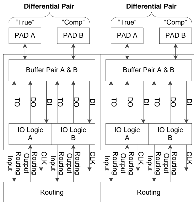
图 3-3 IOB 结构示意图
