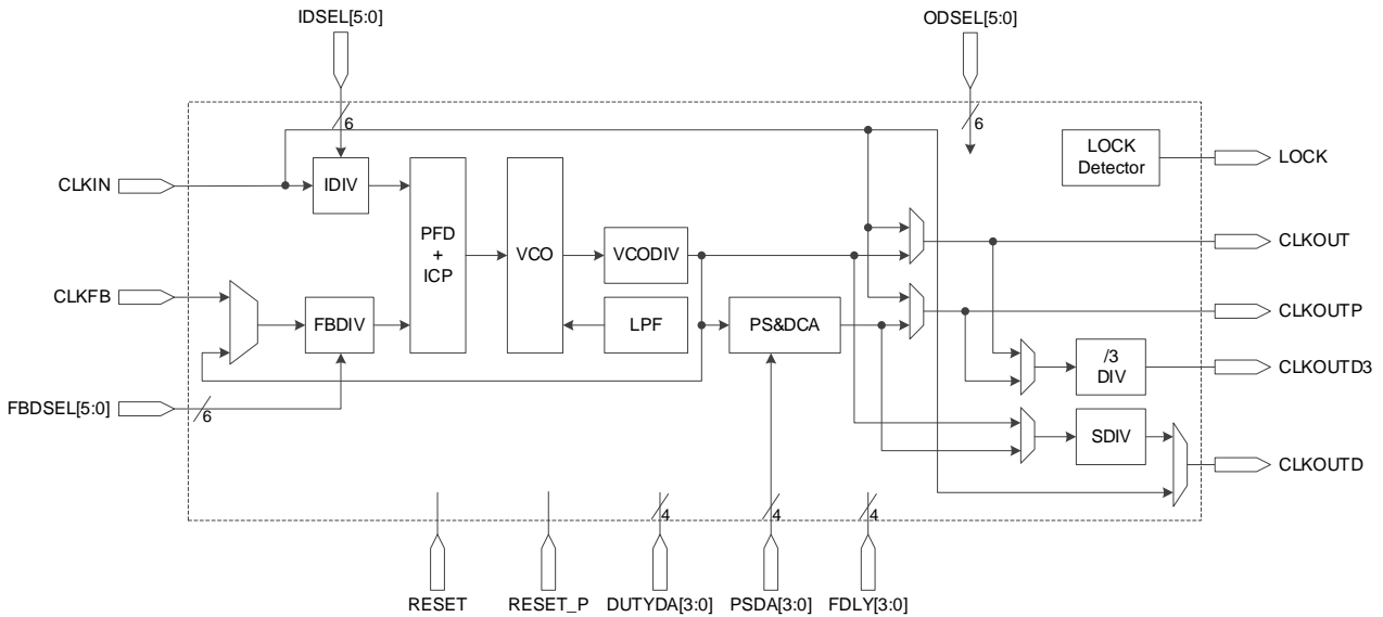
图 3-21 PLL 示意图
