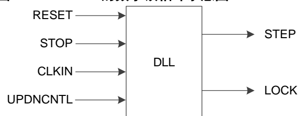
图 3-47 GW2AR 的数字锁相环示意图
