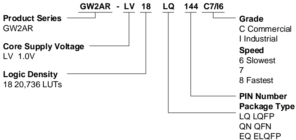
图 5-2 内嵌 SDRAM 器件命名方法 - Production
