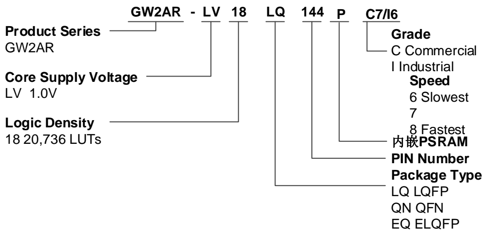
图 5-3 内嵌 PSRAM 器件命名方法 - Production
