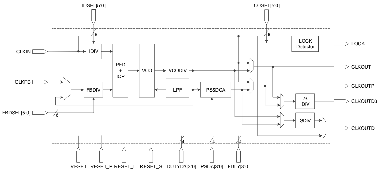
图 3-45 PLL 示意图
