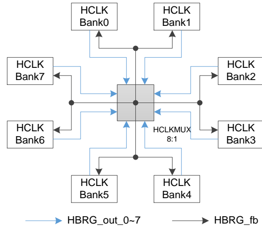
图 3-46 GW2AR HCLK 示意图
