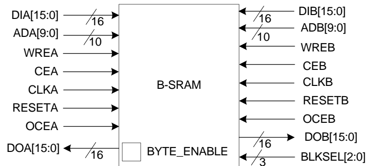
图 3-30 双端口存储模式框图
