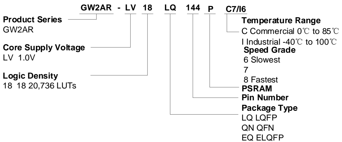
图 5-4 内嵌 PSRAM 器件命名方法 - Production
