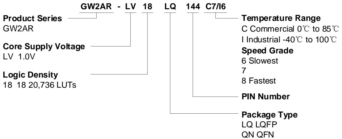
图 5-3 内嵌 SDRAM 器件命名方法 - Production
