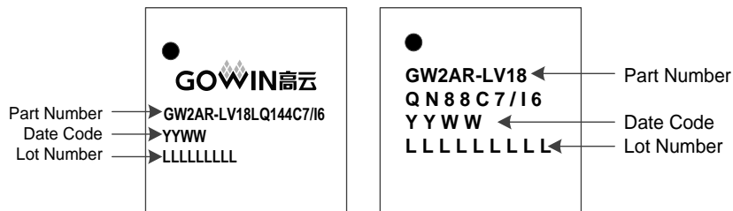
图 5-5 器件封装标识示例
