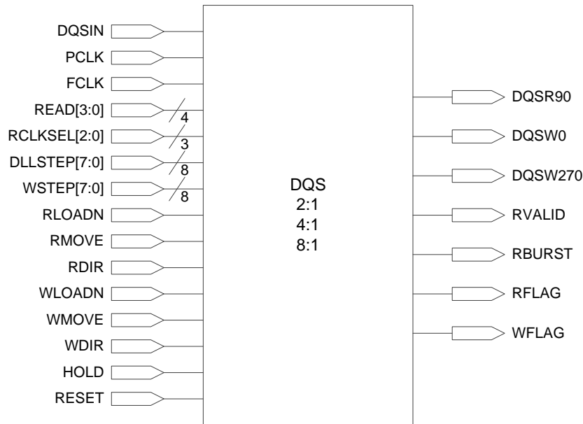
图 3-47 DQS 示意图
