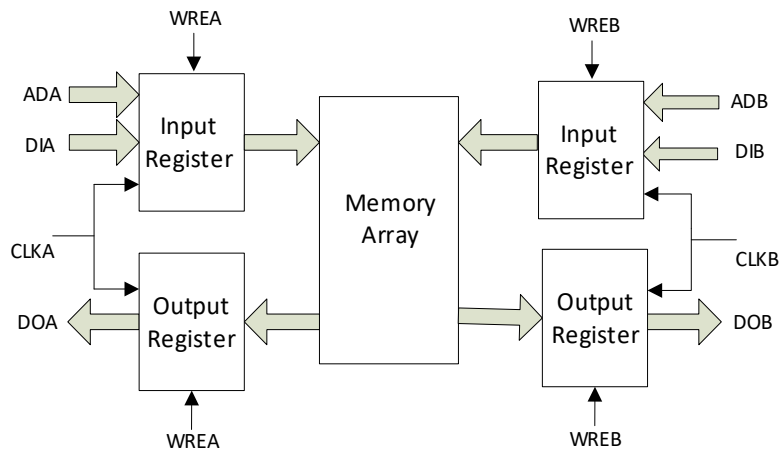
图 3-30 独立时钟模式
