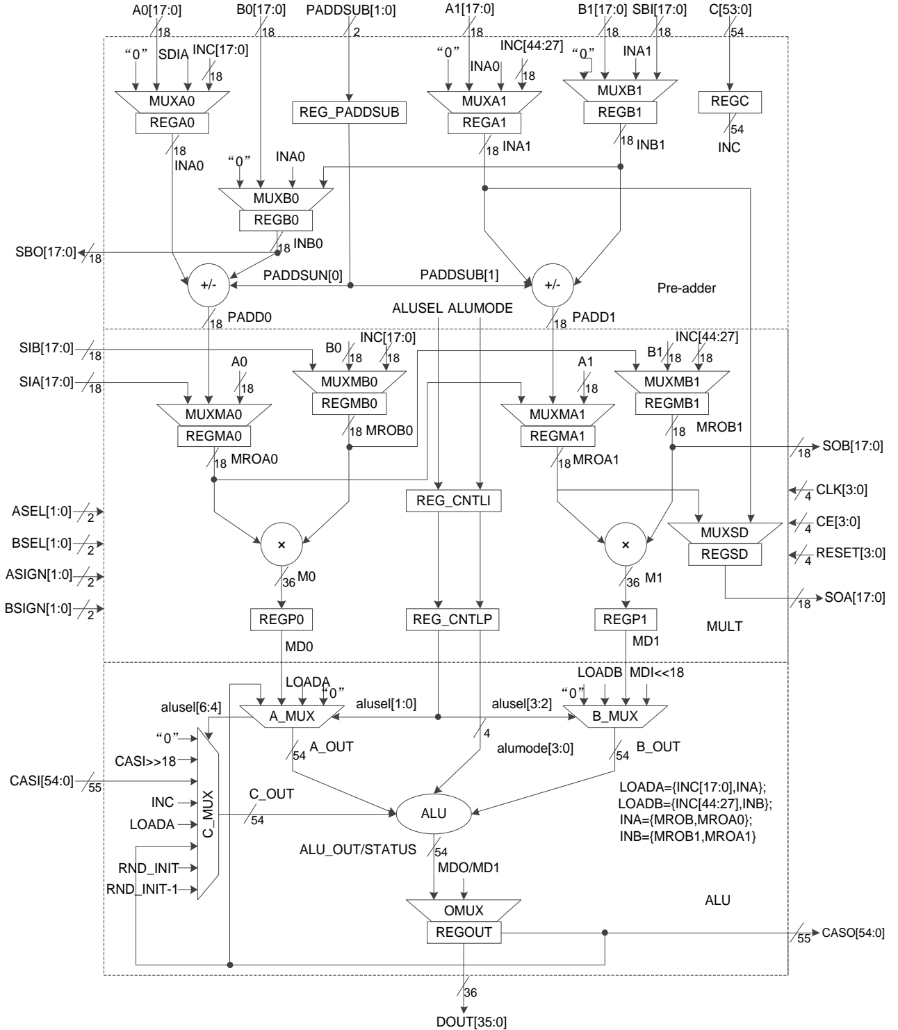
图 3-32 DSP 宏单元
