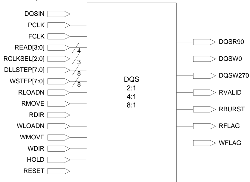
图 3-41 DQS 示意图
