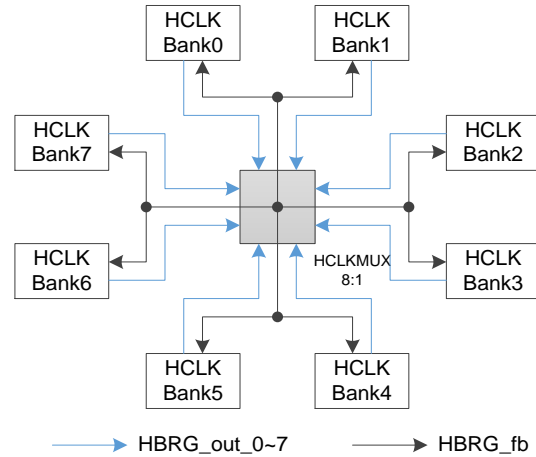
图 3-40 GW2AR HCLK 示意图
