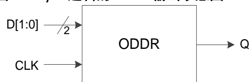
图 3-13 I/O 逻辑的 DDR 输出示意图
