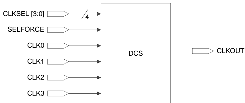
图 3-36 DCS 接口示意图
