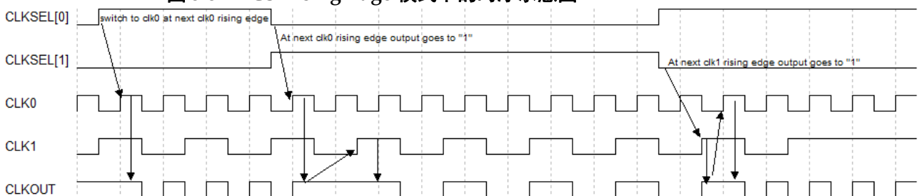
图 3-37 DCS Rising Edge 模式下的时序示意图
