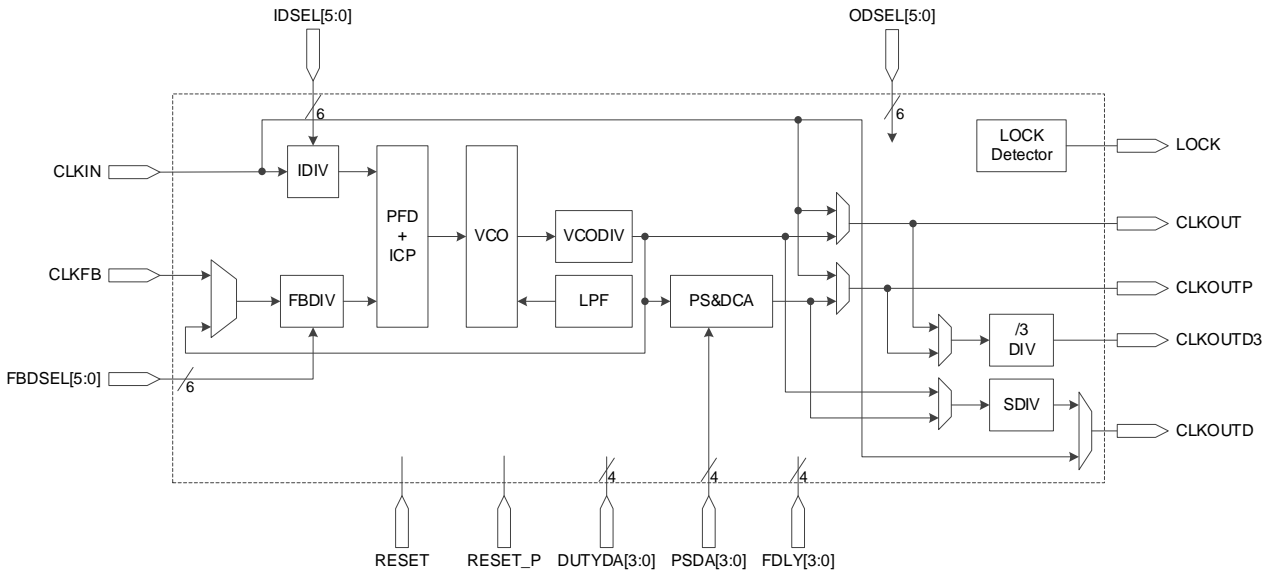
图 3-39 PLL 示意图
