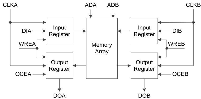
图 3-31 独立时钟模式
