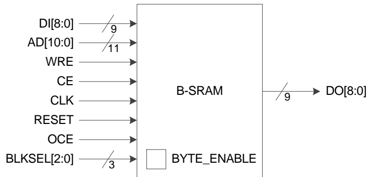
图 3-26 单端口存储模式框图
