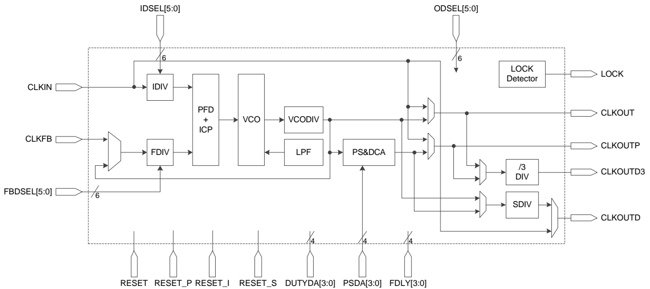
图 3-47 PLL 示意图
