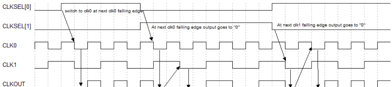
图 3-46 DCS Falling Edge 模式下的时序示意图
