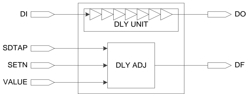
图 3-9 IODELAY 示意图
