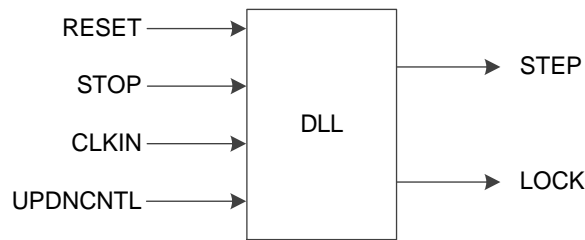
图 3-49 GW1NS-2 的延迟锁相环示意图
