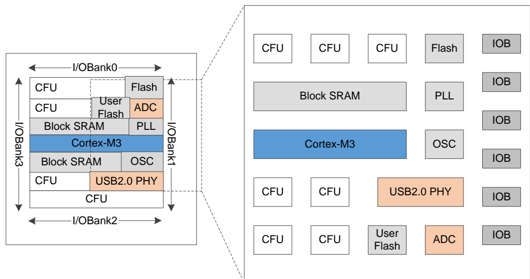
图 3-1 GW1NS-2 器件结构示意图
