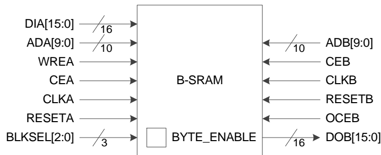
图 3-28 伪双端口存储模式框图 1
