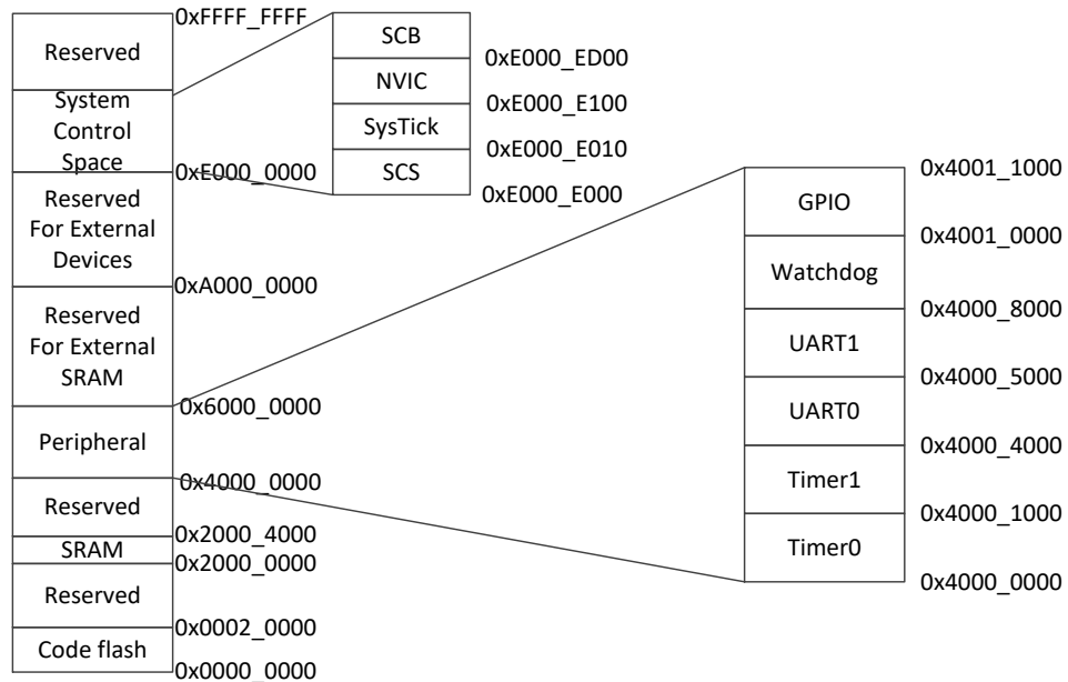
图 3-40 内存映射
