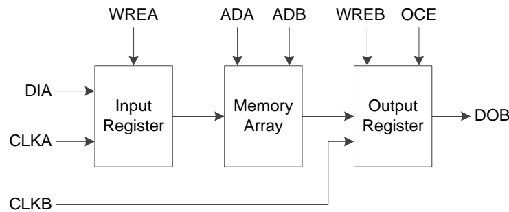
图 3-32 读写时钟模式
