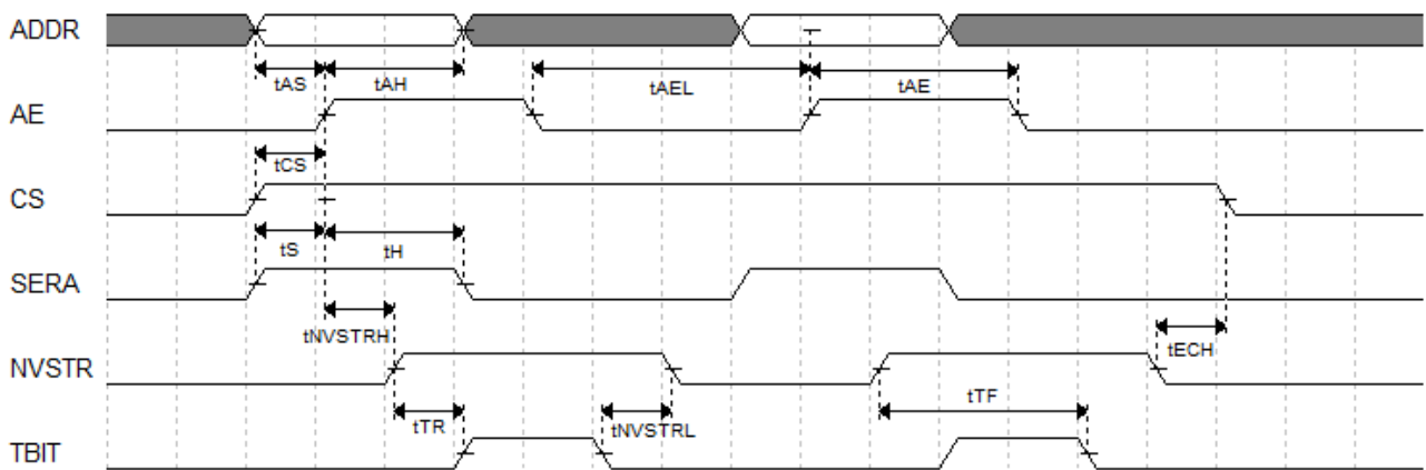
图 4-3 页擦除模式
