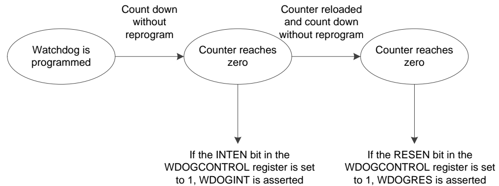
图 3-39 Watchdog 操作方式
