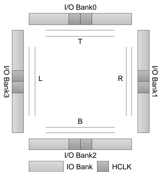
图 3-41 GW1NS-2 时钟资源
