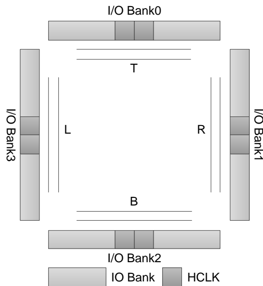
图 3-48 GW1NS-2 HCLK 示意图
