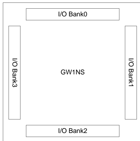
图 3-5 GW1NS 系列 FPGA 产品 I/O Bank 分布示意图
