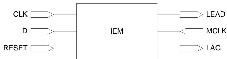
图 3-11 GW1NS 的 IEM 示意图
