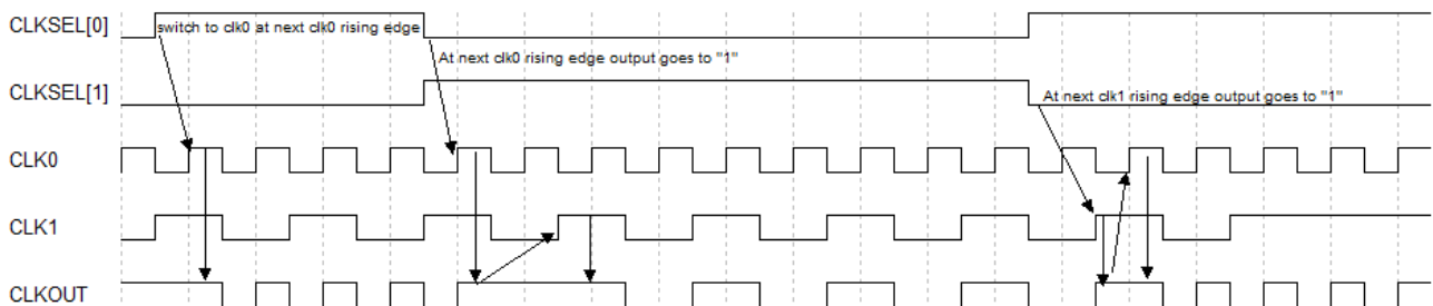
图 3-45 DCS Rising Edge 模式下的时序示意图
