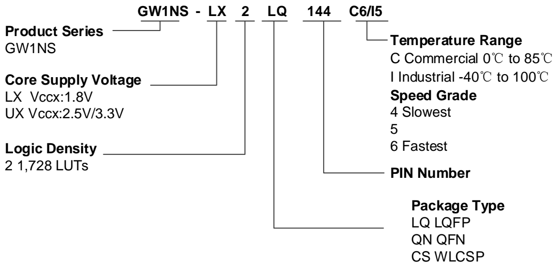
图 5-4 GW1NS-2C 器件命名方法 - Production
