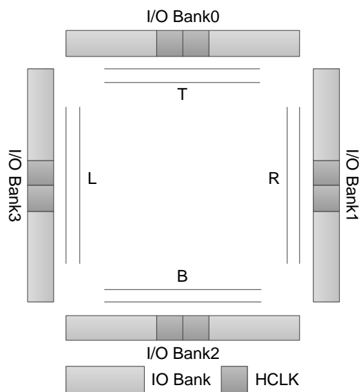
图 3-40 GW1NS-2 时钟资源
