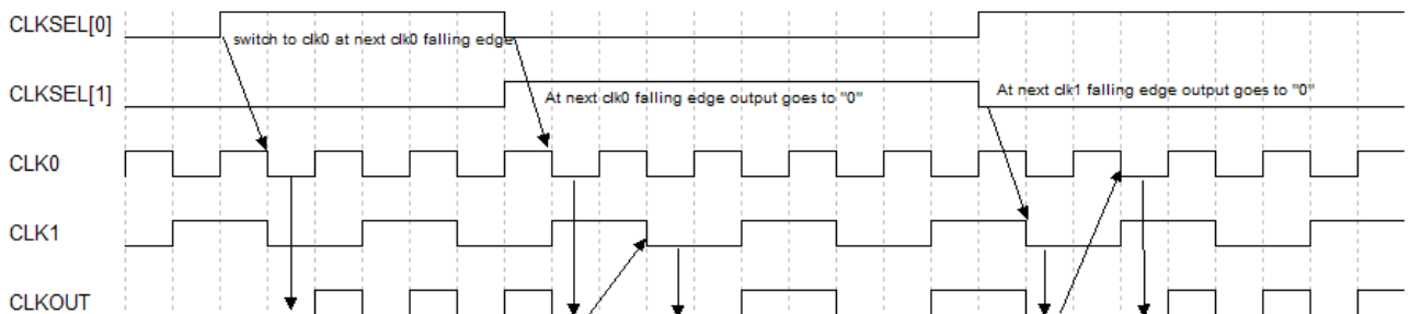
图 3-45 DCS Falling Edge 模式下的时序示意图
