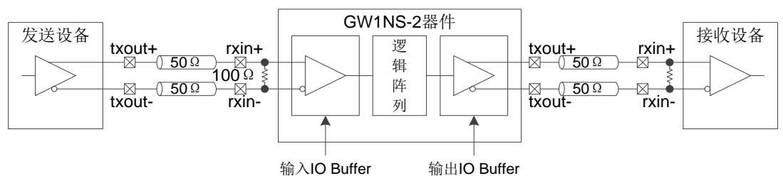
图 3-5 真 LVDS 设计参考框图
