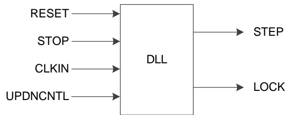
图 3-48 GW1NS-2 的延迟锁相环示意图
