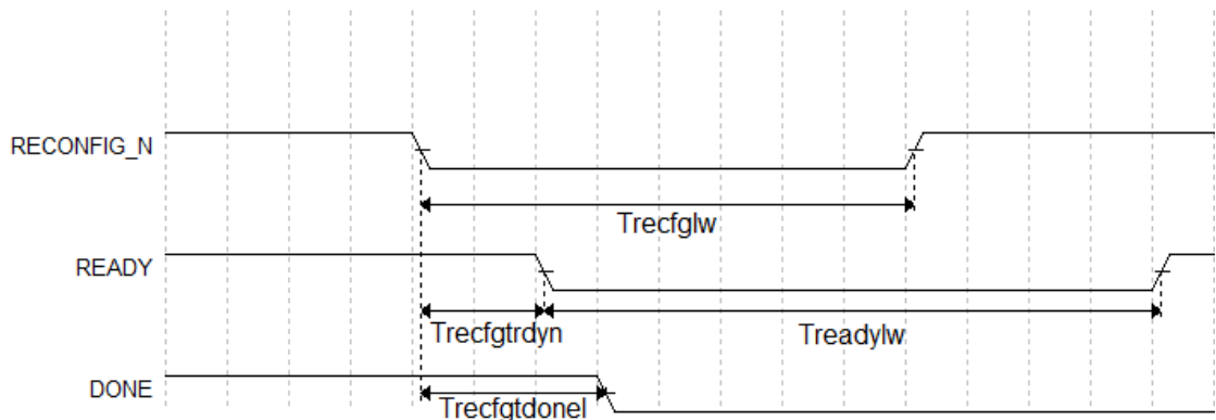
图 4-8 RECONFIG_N 触发时序图
