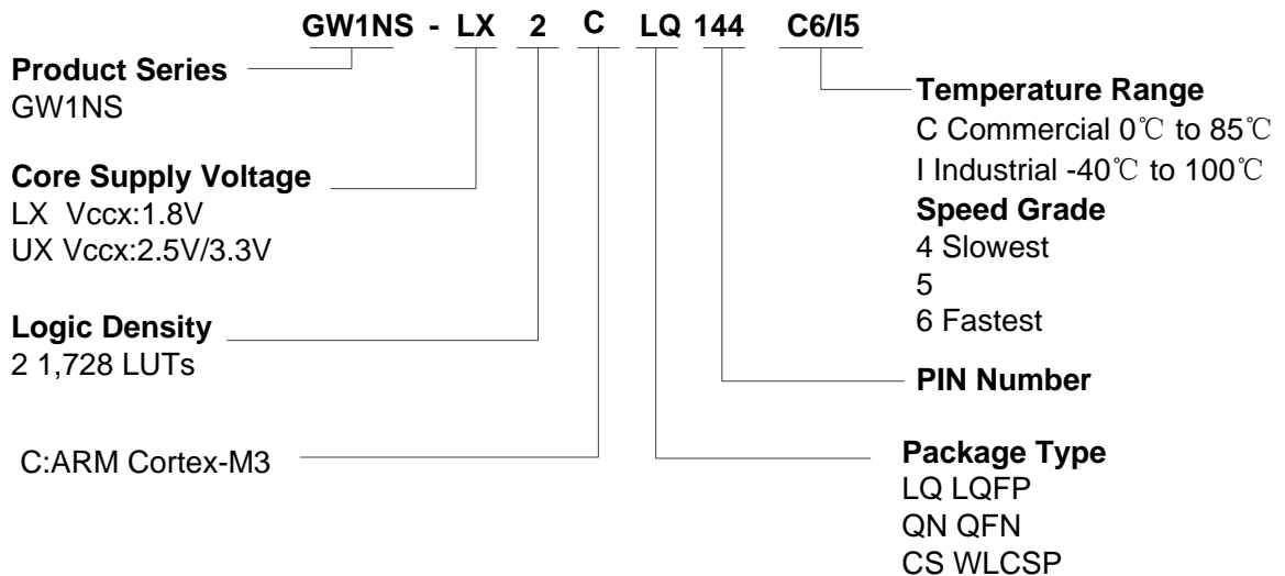
图 5-4 GW1NS-2C 器件命名方法 - Production
