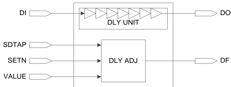
图 3-8 IODELAY 示意图
