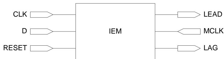
图 3-10 GW1NS 的 IEM 示意图
