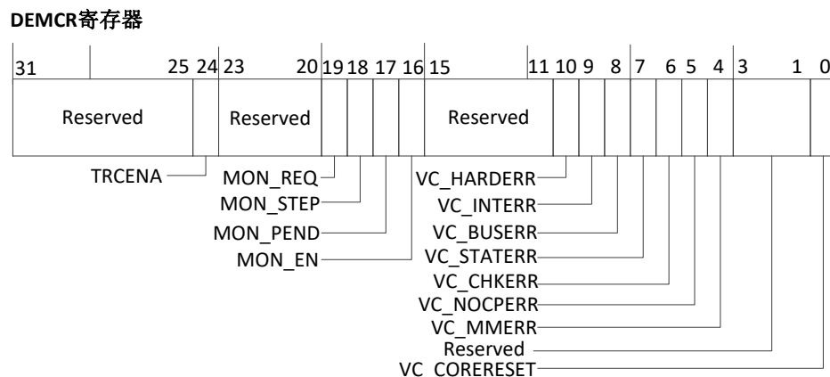
图 3-35 DEMCR 寄存器
