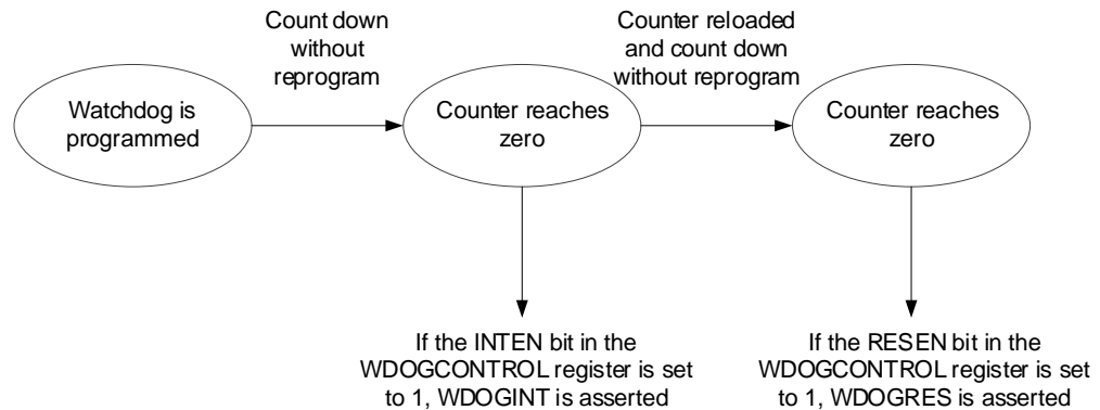
图 3-38 Watchdog 操作方式
