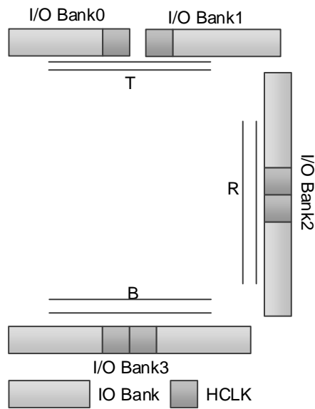
图 3-42 GW1NS-4C/4 HCLK 示意图
