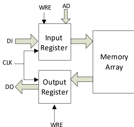
图 3-33 单端口时钟模式
