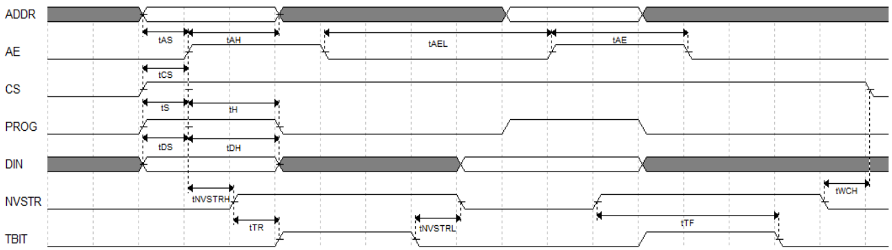
图 4-2 写操作模式
