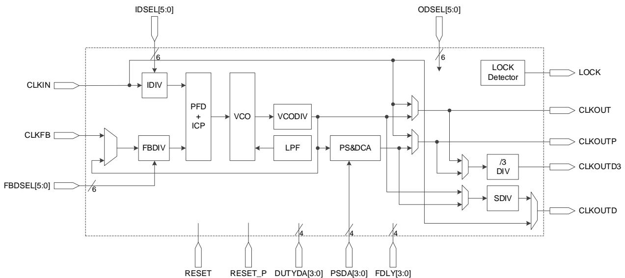
图 3-40 PLL 示意图
