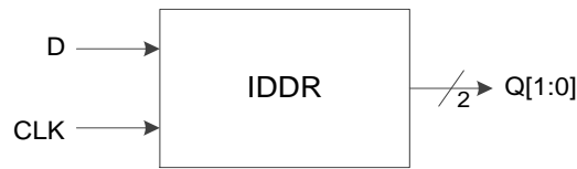
图 3-18 I/O 逻辑的 DDR 输入示意图
