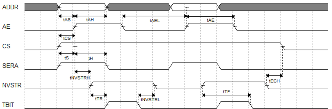
图 4-3 页擦除模式
