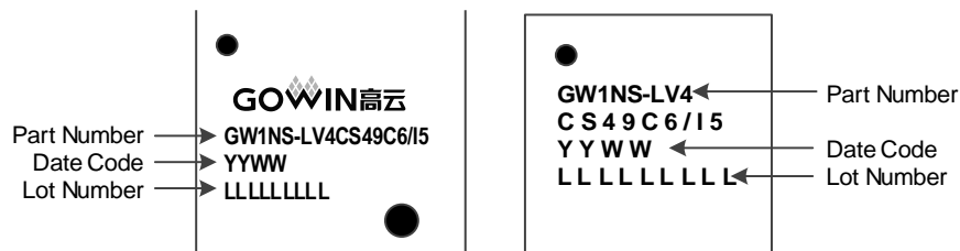
图 5-7 GW1NS-4 器件封装标识示例
