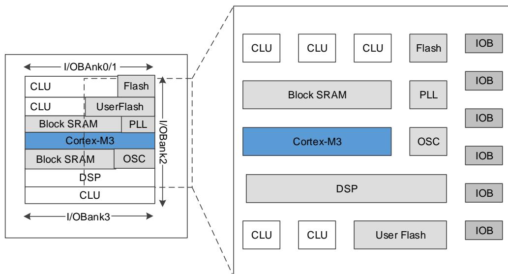
图 3-2 GW1NS-4C 器件结构示意图
