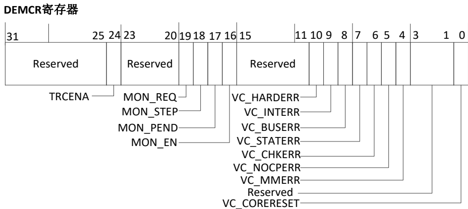
图 3-30 DEMCR 寄存器
