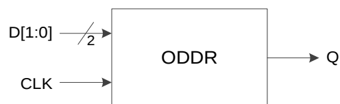
图 3-14 I/O 逻辑的 DDR 输出示意图
