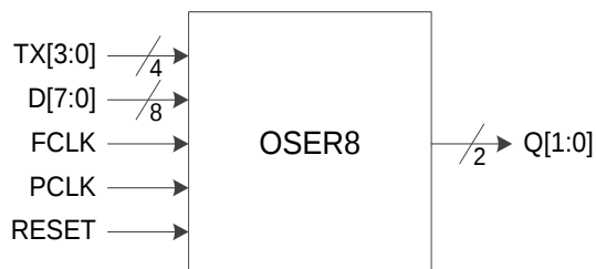
图 3-20 I/O 逻辑的 OSER8 输出示意图
