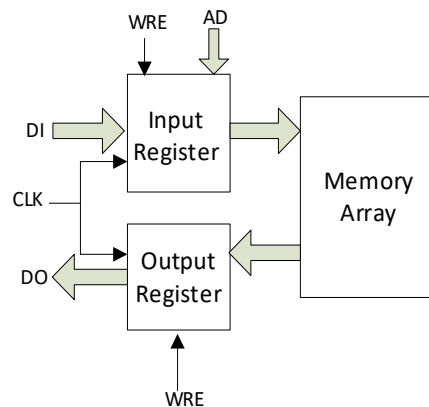
图 3-28 单端口时钟模式
