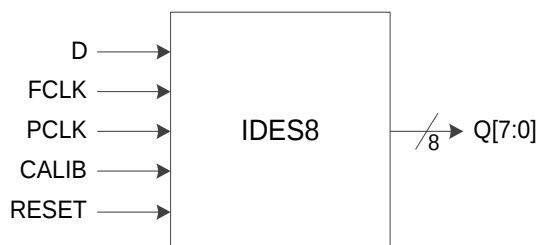
图 3-19 I/O 逻辑的 IDES8 输入示意图
