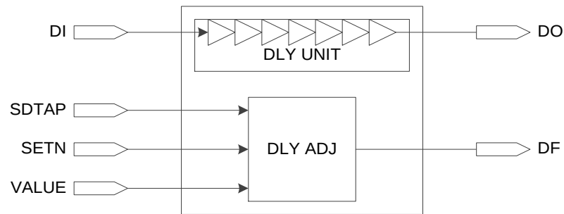
图 3-8 IODELAY 示意图
