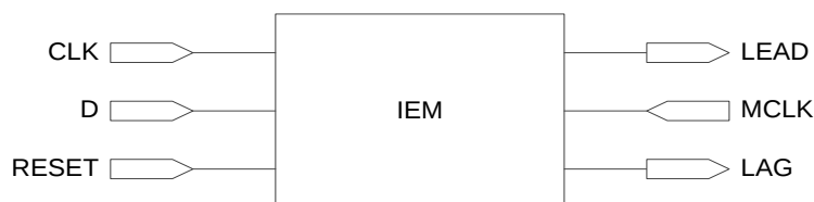
图 3-10 GW1NS 的 IEM 示意图
