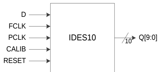
图 3-21 I/O 逻辑的 IDES10 输入示意图
