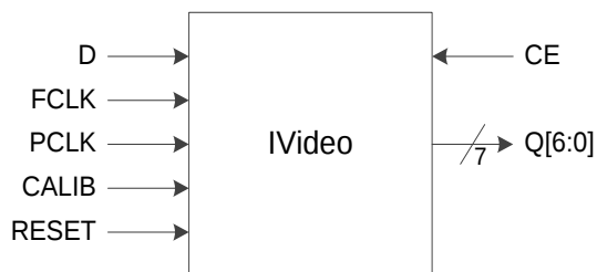
图 3-17 I/O 逻辑的 IVideo 输入示意图
