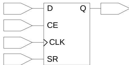
图 3-9 GW1NS 的 I/O 寄存器示意图
