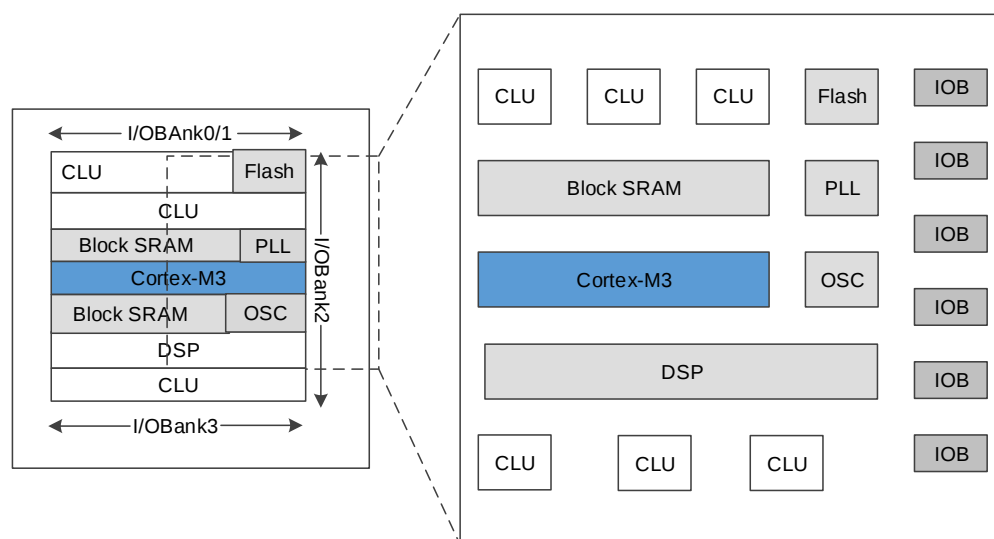
图 3-2 GW1NS-4C 器件结构示意图
