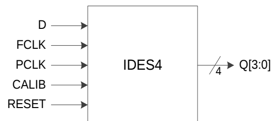
图 3-15 I/O 逻辑的 IDES4 输入示意图
