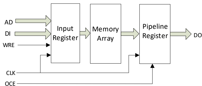
图 3-25 单端口、伪双端口及双端口模式下的流水线模式
