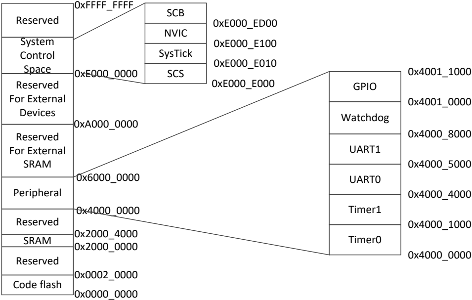
图 3-34 内存映射
