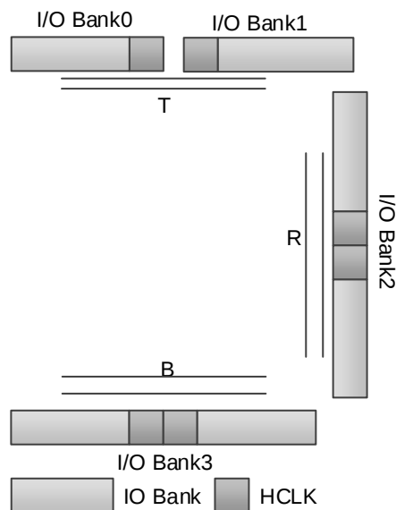
图 3-36 GW1NS-4C/4 HCLK 示意图
