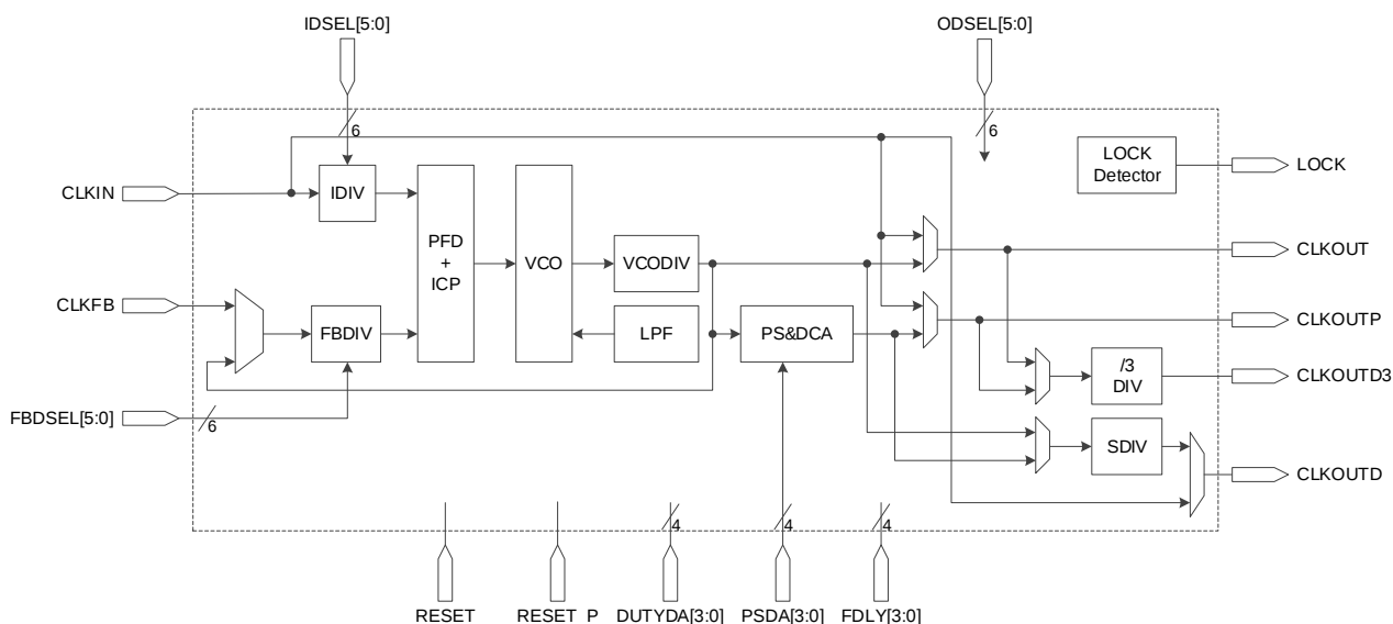
图 3-35 PLL 示意图
