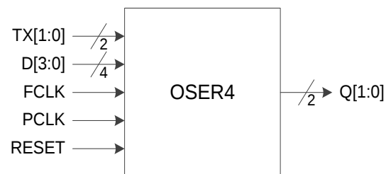
图 3-16 I/O 逻辑的 OSER4 输出示意图
