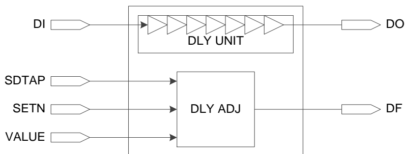
图 2-8 IODELAY 示意图
