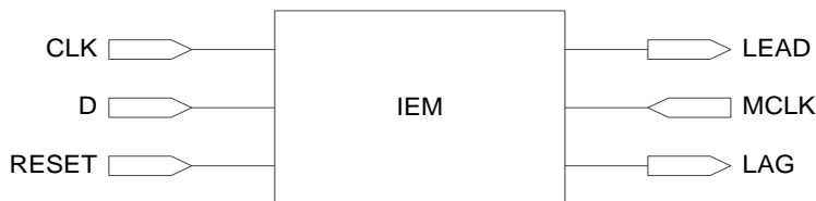
图 2-10 GW1NS 的 IEM 示意图
