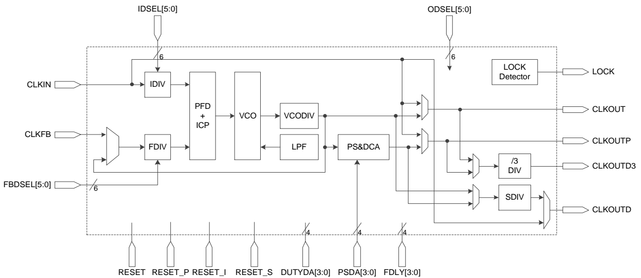
图 3-38 PLL 示意图
