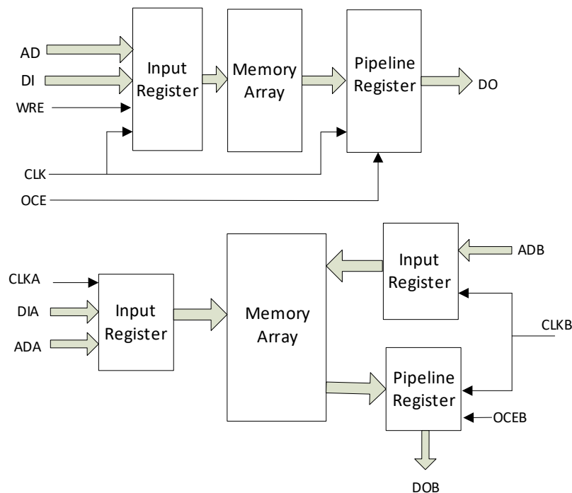
图 3-24 单端口、伪双端口及双端口模式下的流水线模式
