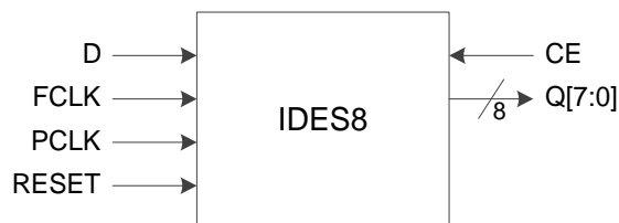
图 3-20 I/O 逻辑的 IDES8 输入示意图
