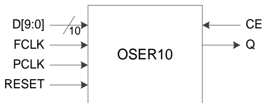
图 3-23 I/O 逻辑的 OSER10 输出示意图
