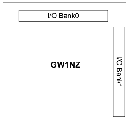
图 3-6 GW1NZ-2 的 I/O Bank 分布示意图
