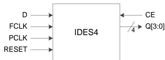
图 3-16 I/O 逻辑的 IDES4 输入示意图
