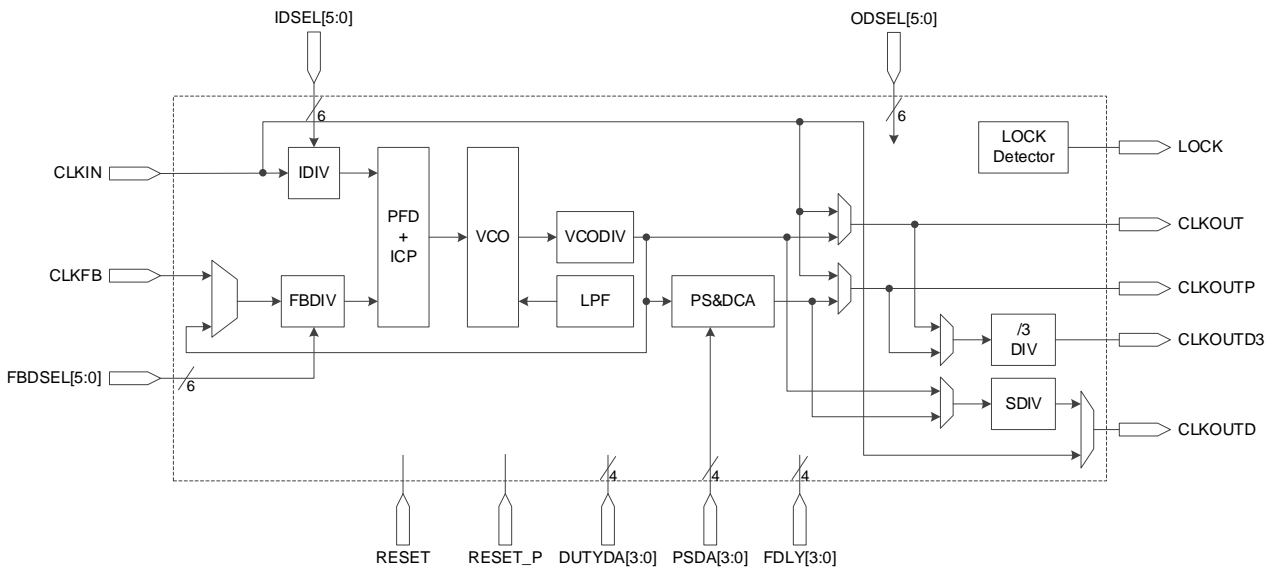
图 3-36 PLL 示意图
