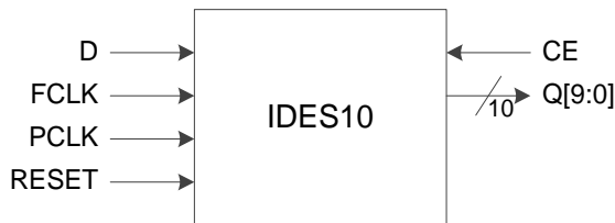
图 3-22 I/O 逻辑的 IDES10 输入示意图
