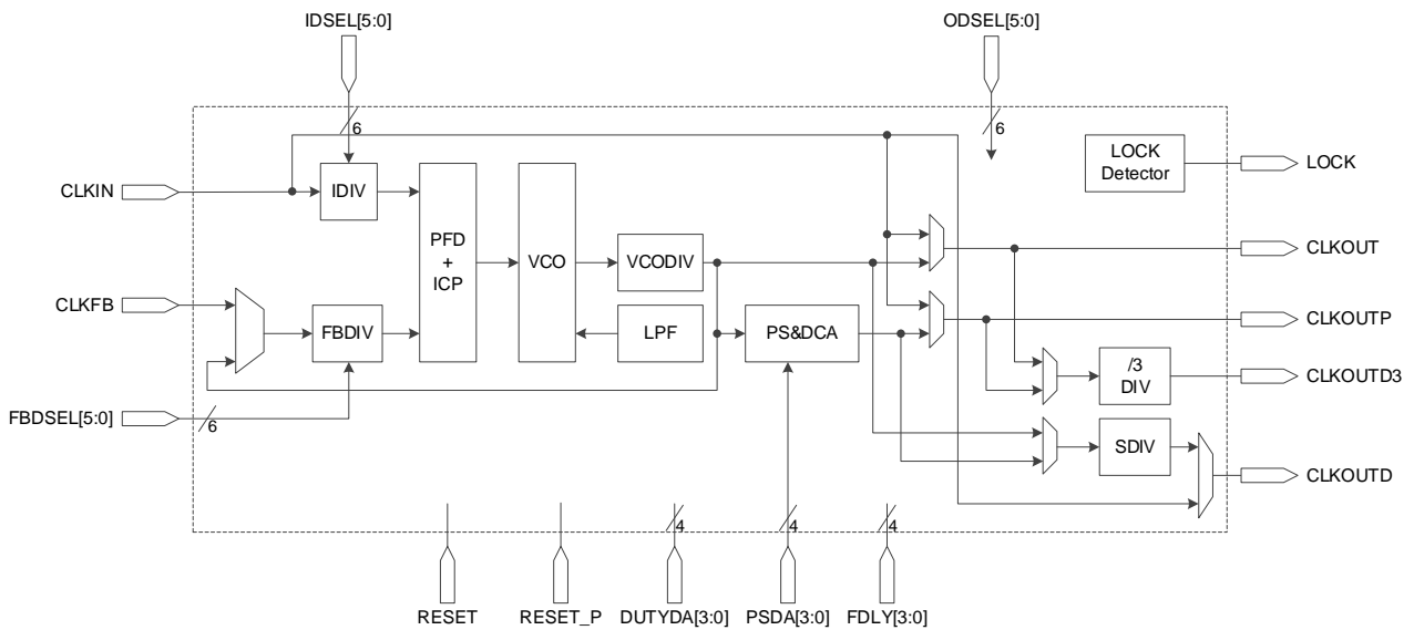
图 3-15 PLL 示意图
