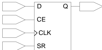
图 3-9 GW1NZ 的 I/O 寄存器示意图
