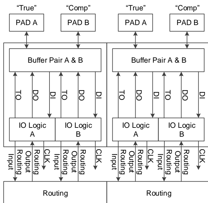
图 3-4 IOB 结构示意图
