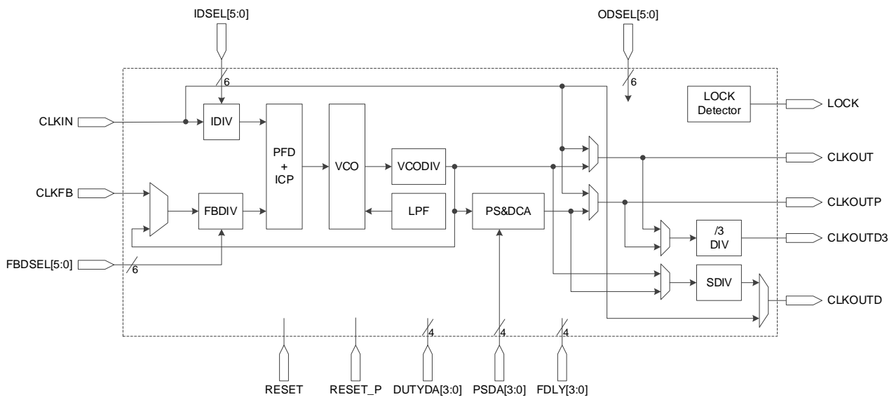
图 3-22 PLL 示意图
