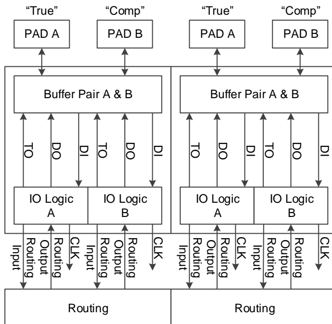
图 3-3 IOB 结构示意图
