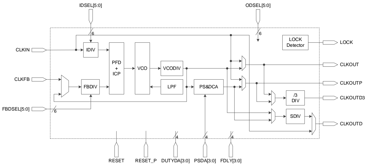
图 3-14 PLL 示意图
