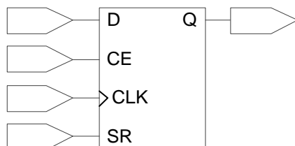
图 3-8 GW1NZ 的 I/O 寄存器示意图
