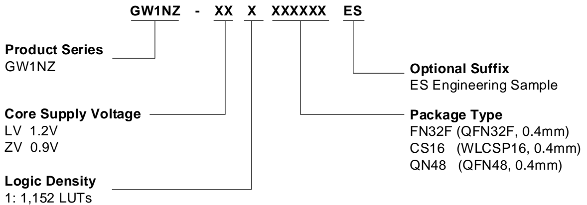
图 5-2 器件命名方法示例 - Production
