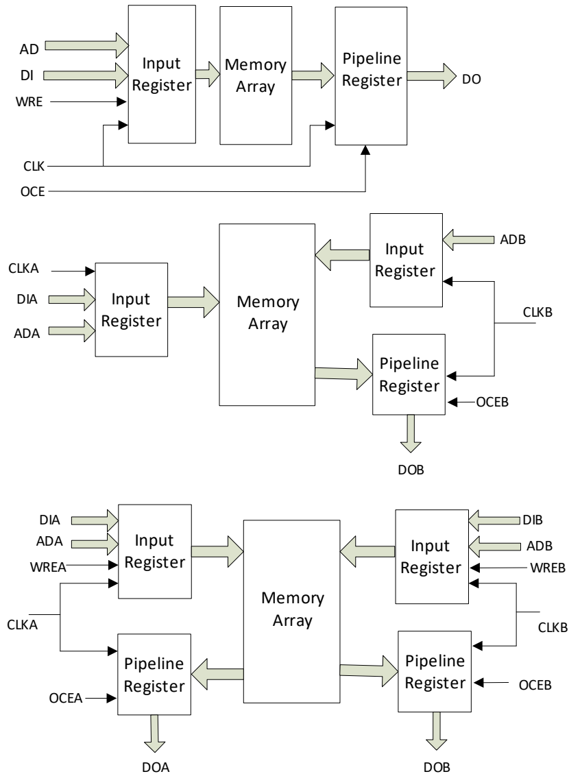
图 3-10 单端口、伪双端口及双端口模式下的流水线模式
