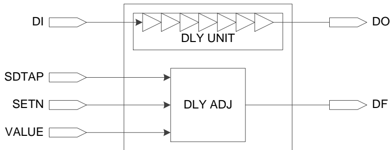
图 3-7 IODELAY 示意图
