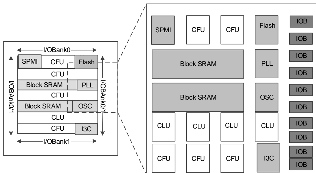
图 3-1 GW1NZ-1 器件结构概念示意图
