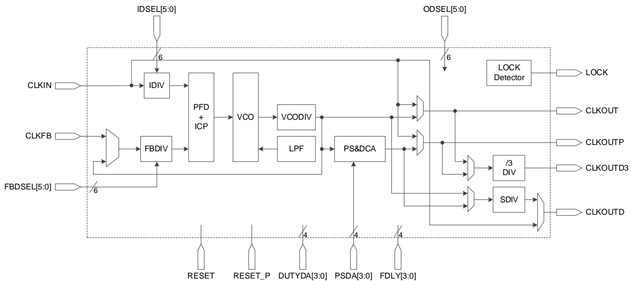
图 3-14 PLL 示意图
