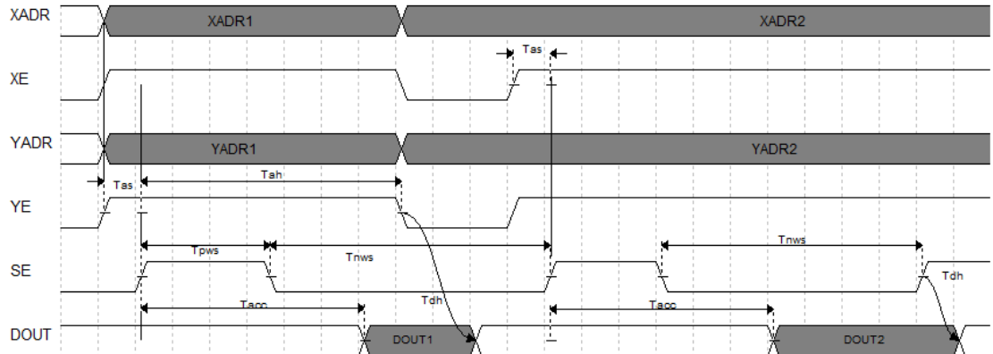
图 4-1 读操作模式
