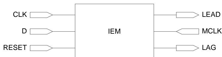
图 3-10 GW1NZ 的 IEM 示意图
