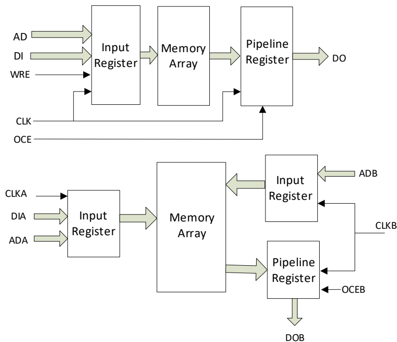
图 3-11 单端口、伪双端口及双端口模式下的流水线模式
