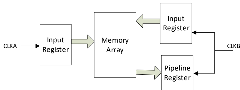
图 3-13 读写时钟模式
