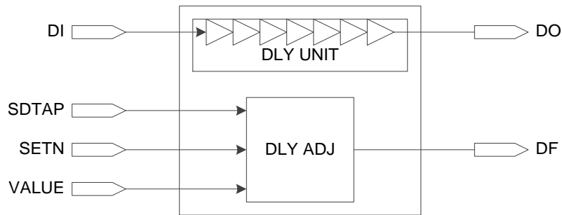
图 3-8 IODELAY 示意图
