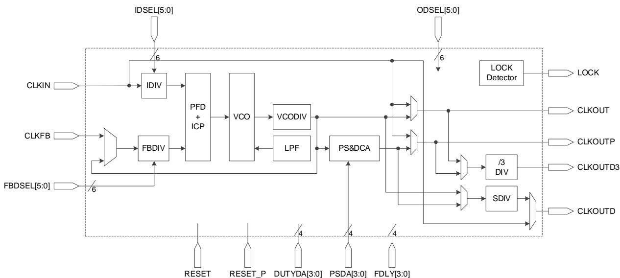
图 3-15 PLL 示意图
