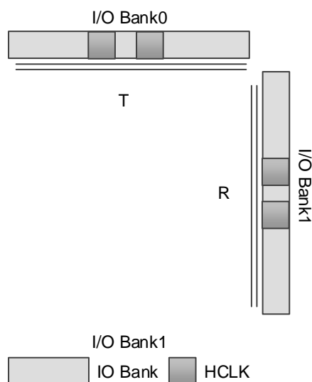
图 3-16 GW1NZ-1 HCLK 示意图
