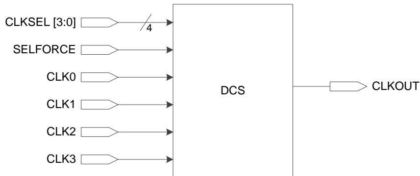
图 3-19 DCS 接口示意图
