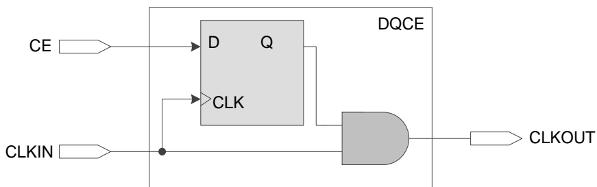
图 3-18 DQCE 结构示意图
