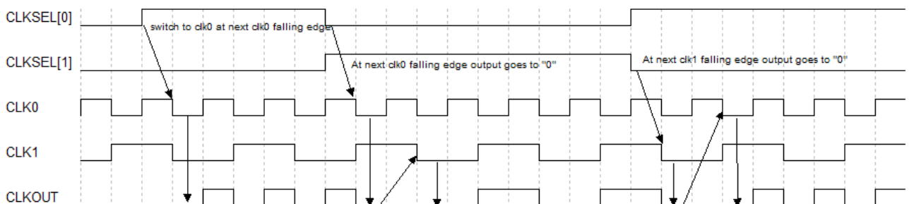
图 3-21 DCS Falling Edge 模式下的时序示意图
