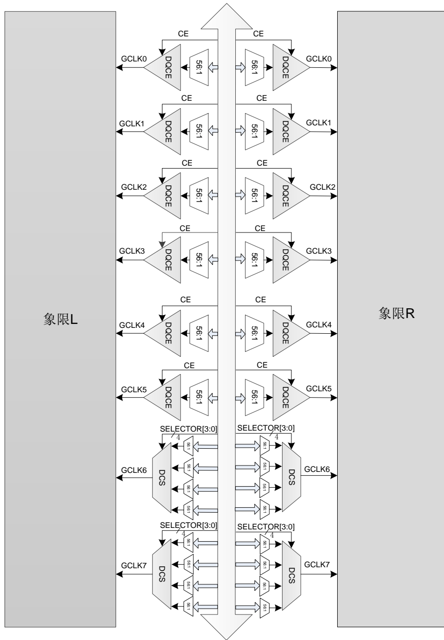
图 3-17 GCLK 象限分布示意
