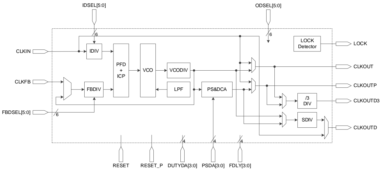
图 3-22 PLL 示意图
