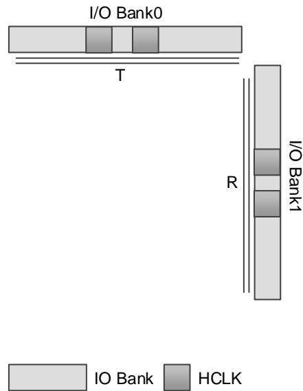
图 3-16 GW1NZ-1 器件时钟资源
