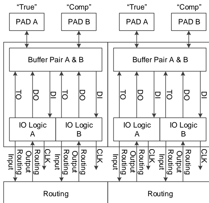
图 3-4 IOB 结构示意图
