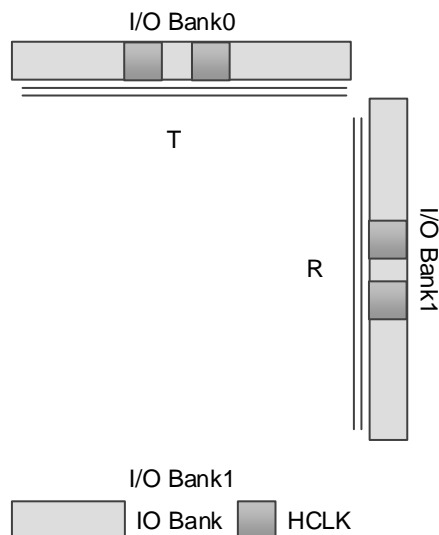
图 3-23 GW1NZ-1 HCLK 示意图
