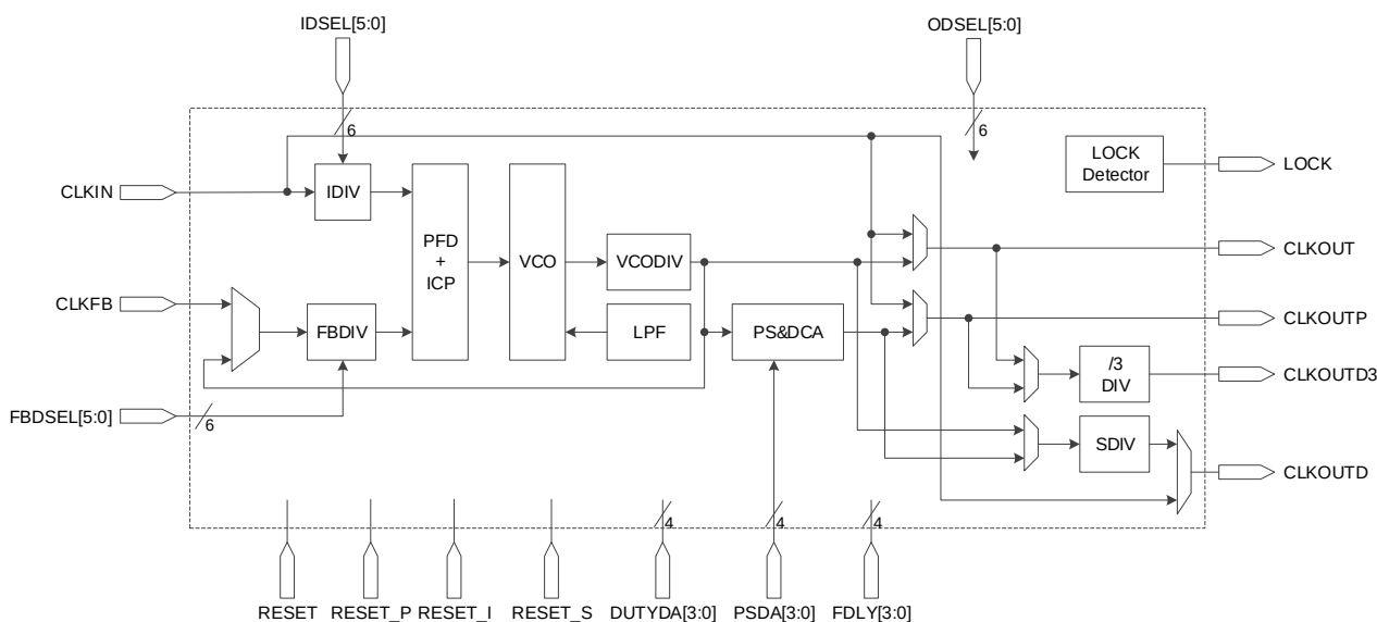
图 3-54 PLL 示意图
