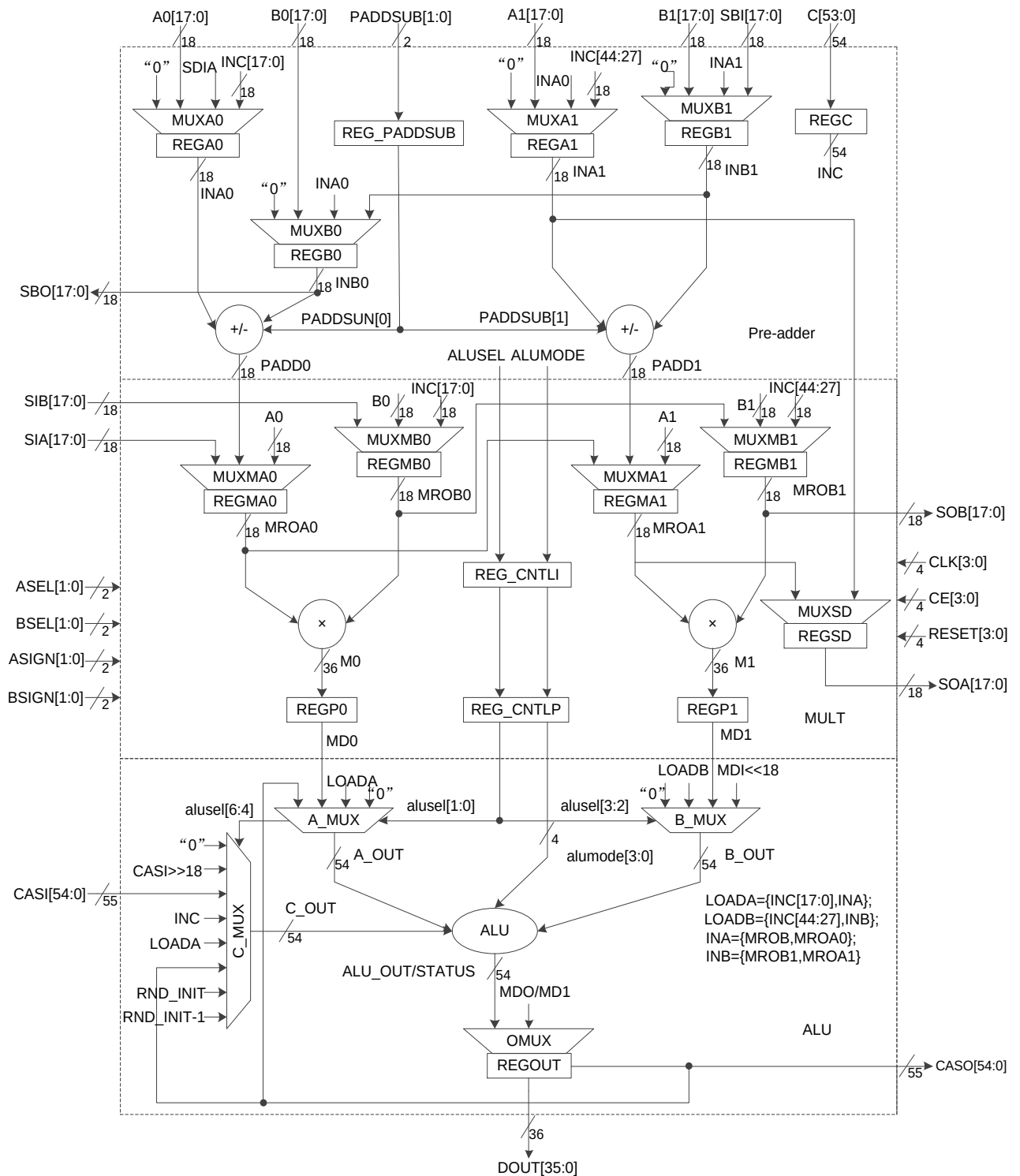
图 3-40 DSP 宏单元
