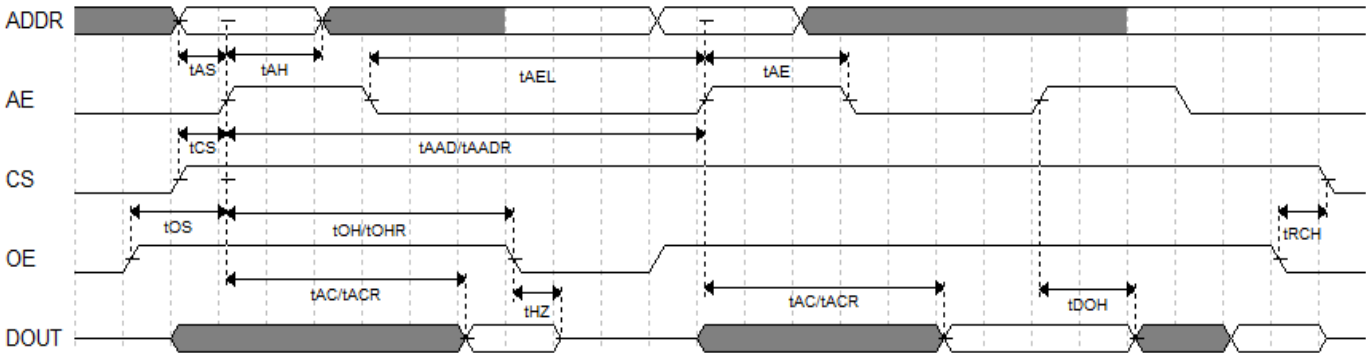
图 4-1 读操作模式
