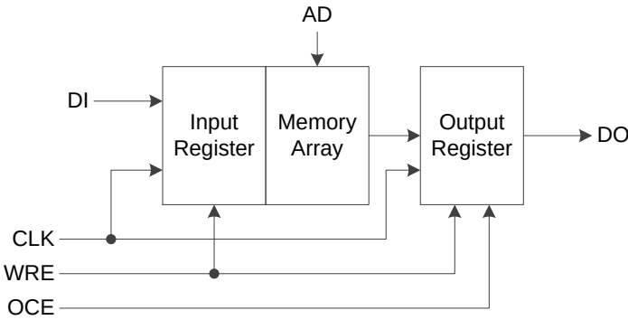
图 3-34 单端口、伪双端口及双端口模式下的流水线模式
