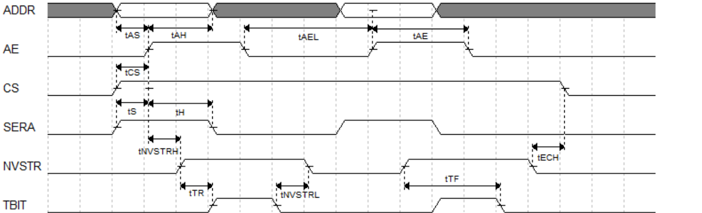
图 4-3 页擦除模式
