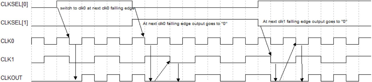
图 3-53 DCS Falling Edge 模式下的时序示意图
