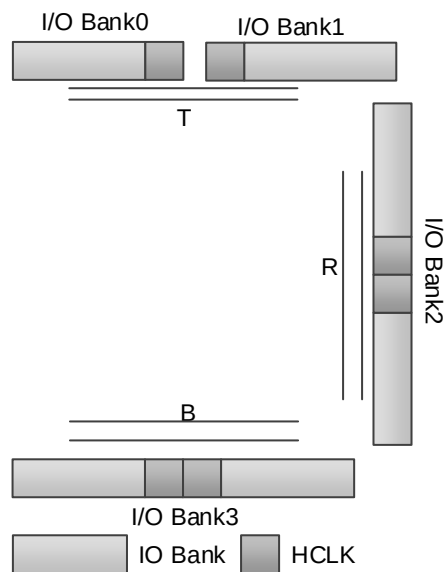
图 3-56 GW1NSR-4/4C HCLK 示意图
