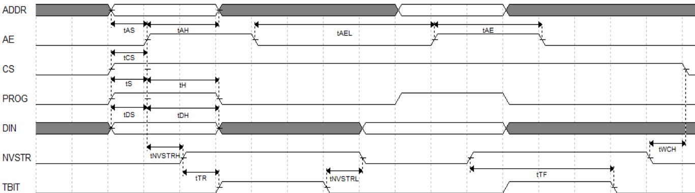
图 4-2 写操作模式
