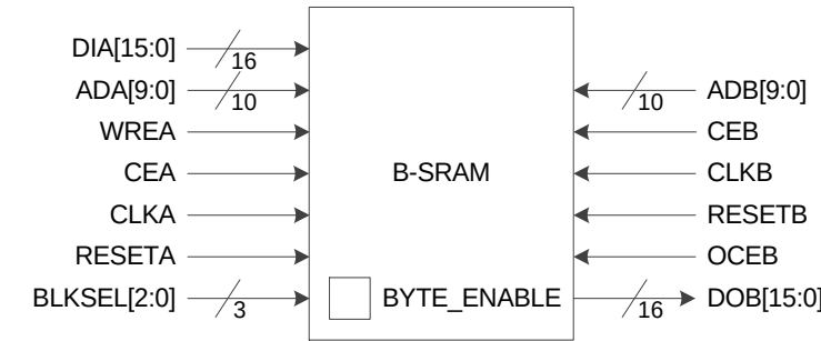
图 3-32 伪双端口存储模式框图
