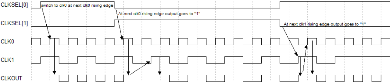
图 3-52 DCS Rising Edge 模式下的时序示意图
