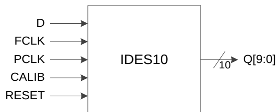
图 3-26 I/O 逻辑的 IDES10 输入示意图
