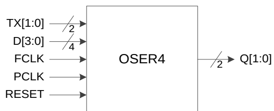
图 3-21 I/O 逻辑的 OSER4 输出示意图
