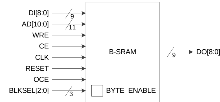
图 3-30 单端口存储模式框图
