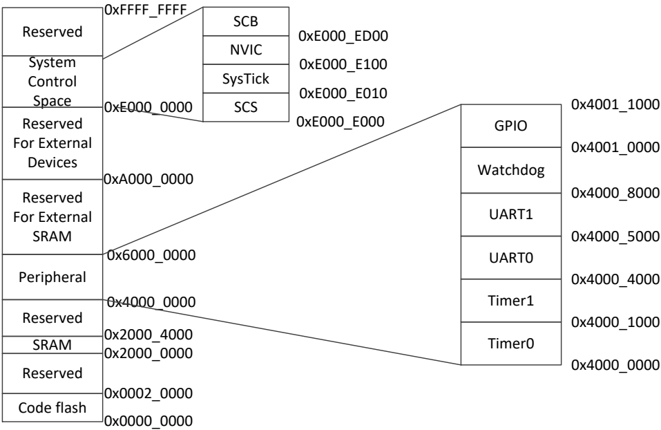
图 3-46 内存映射
