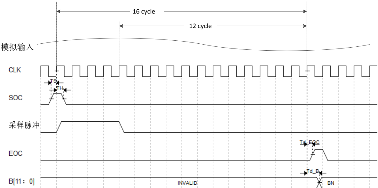
图 4-8ADC 转换时序
