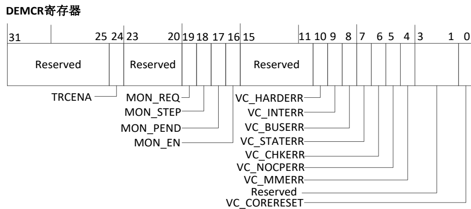
图 3-35 DEMCR 寄存器
