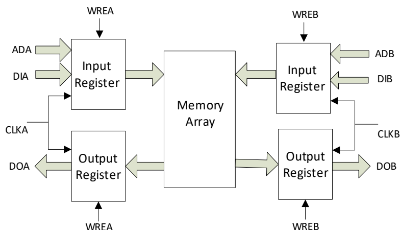
读写时钟模式
