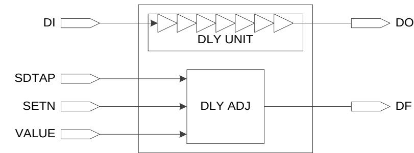
图 2-8 IODELAY 示意图
