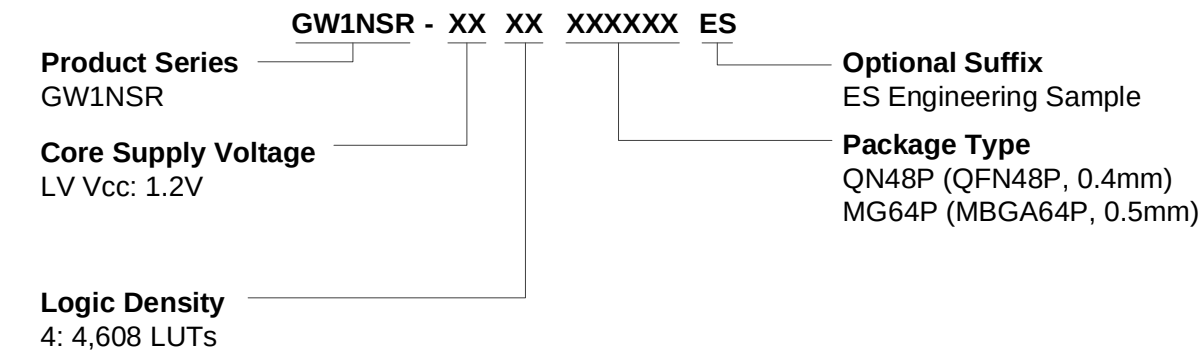
图 4-1 GW1NSR-4 器件命名方法示例 - ES
