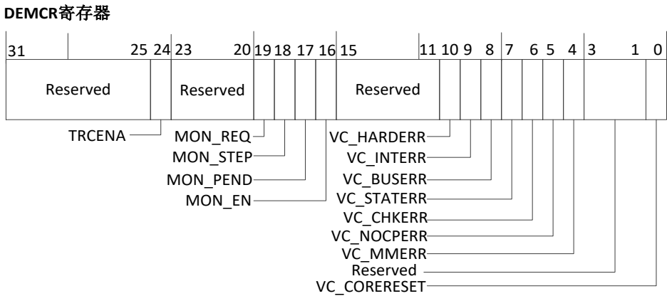
图 2-16 DEMCR 寄存器
