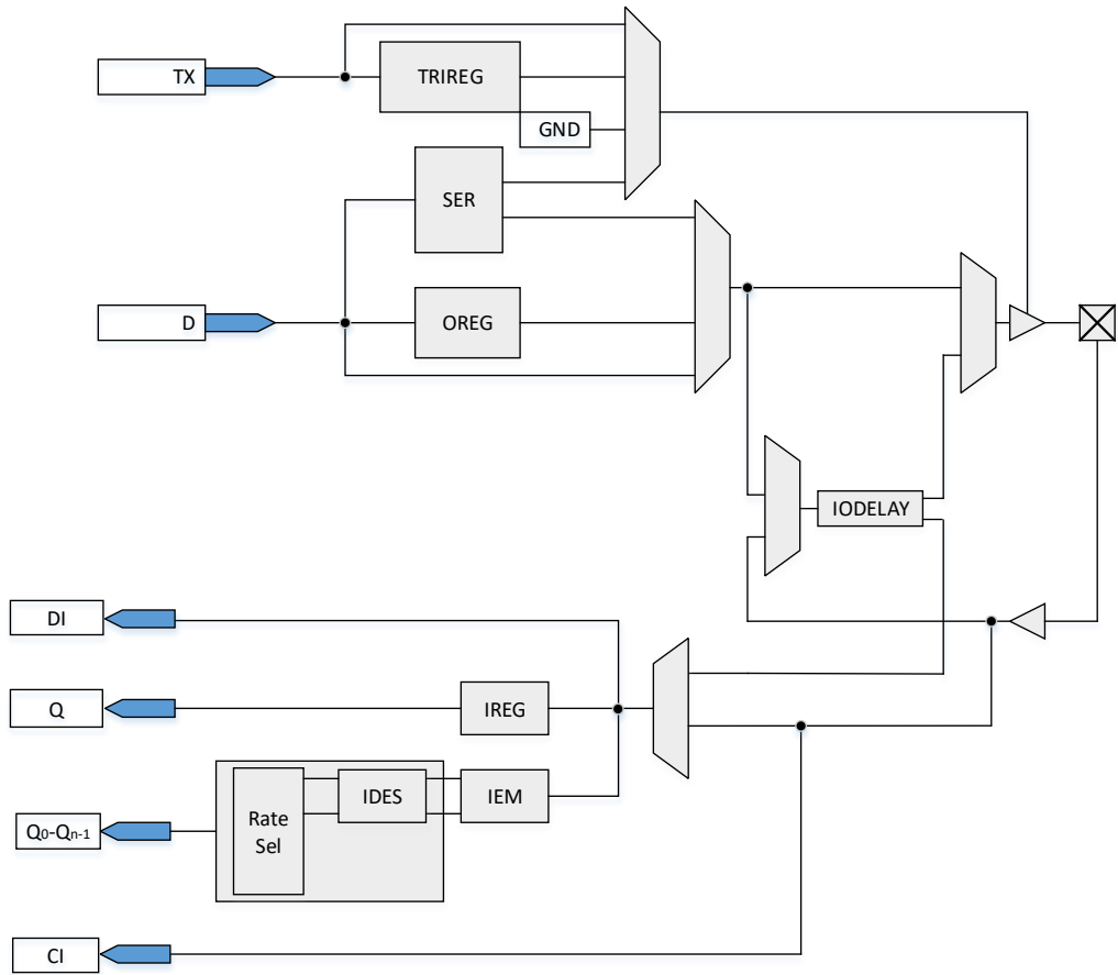
图 2-7 I/O 逻辑输入输出示意图
