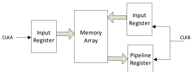
单端口时钟模式
