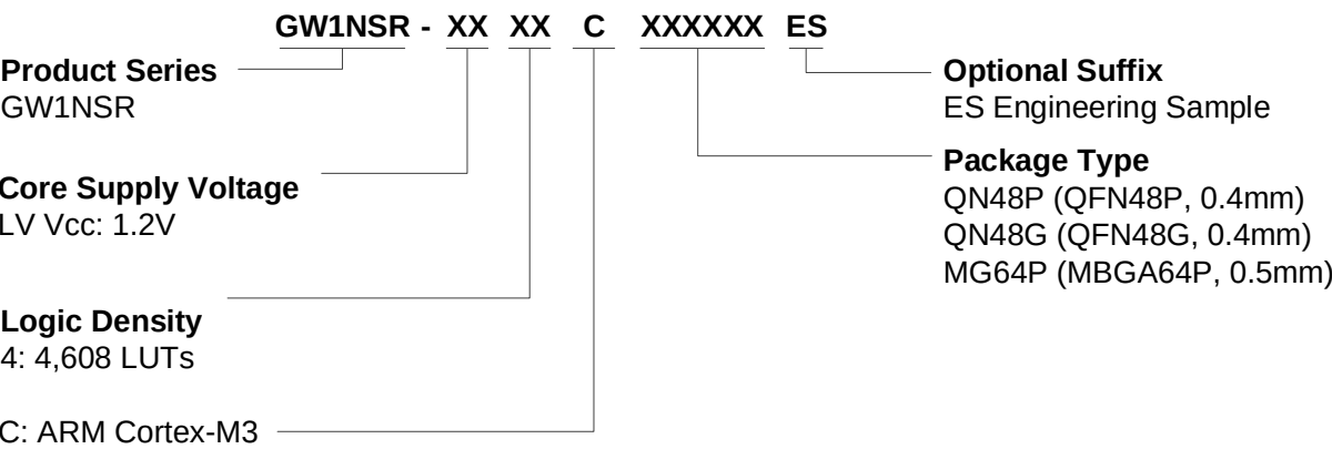
图 4-2 GW1NSR-4C 器件命名方法示例 - ES
