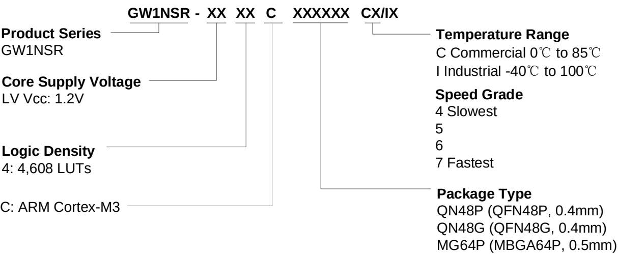
图 4-4 GW1NSR-4C 器件命名方法示例 - Production
