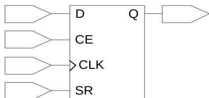
图 2-9 I/O 寄存器示意图
