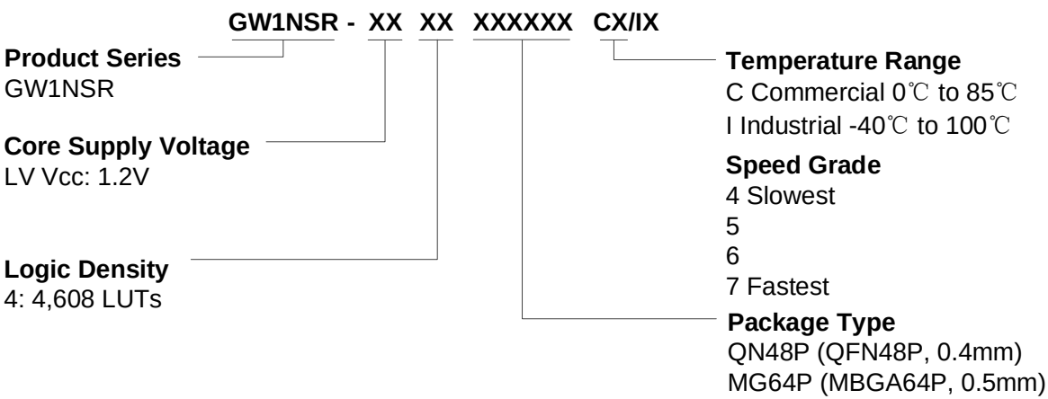
图 4-3 GW1NSR-4 器件命名方法示例 - Production
