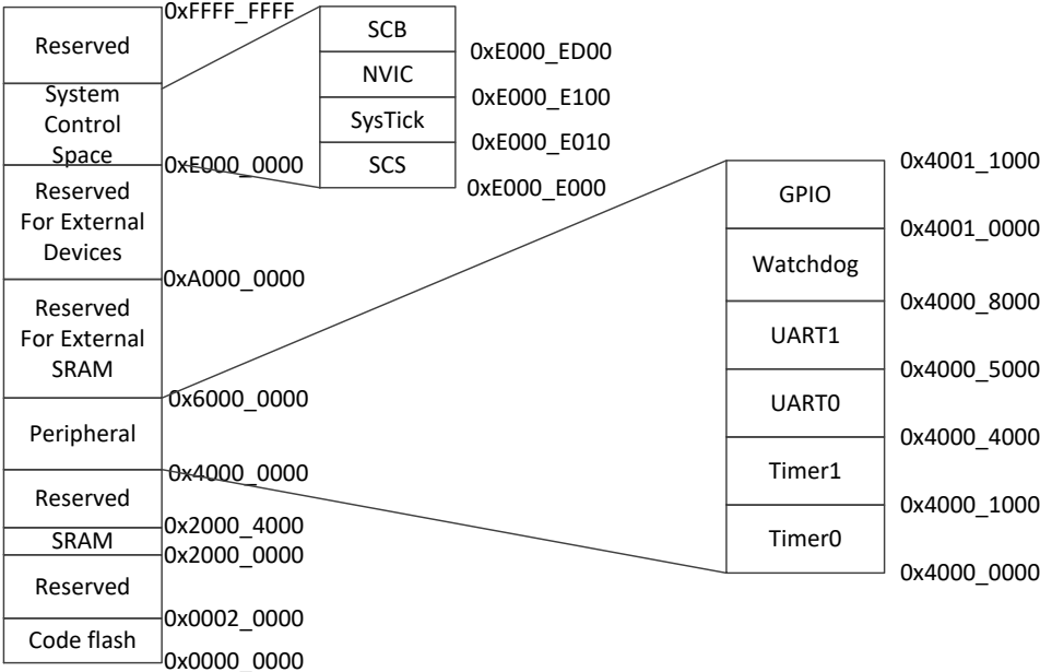
图 2-20 内存映射
