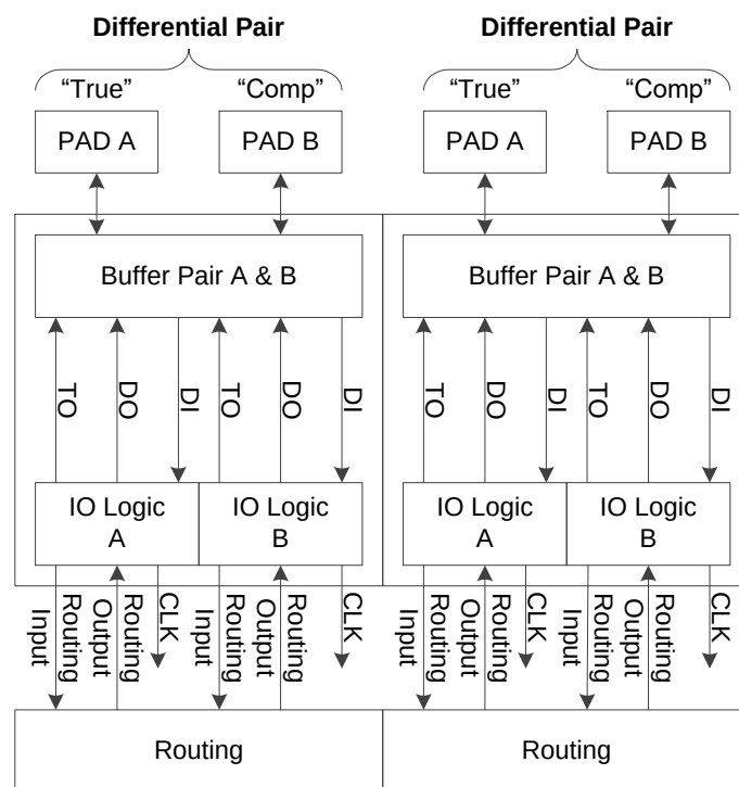
图 2-4 IOB 结构示意图
