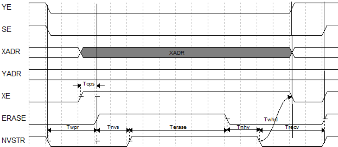
图 3-3 擦除操作时序
