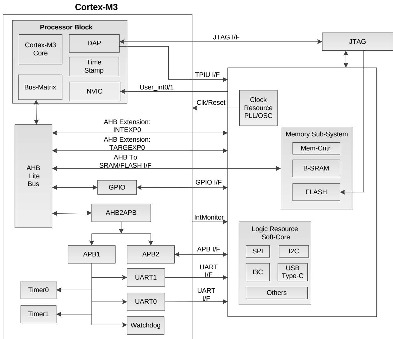
图 3-35 Cortex-M3 结构框图
