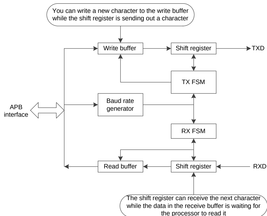
图 3-38 APB UART Buffering
