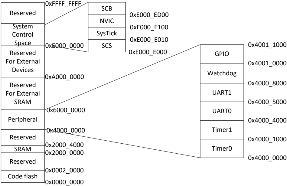
图 3-40 内存映射
