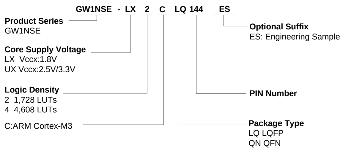
图 5-2 GW1NSE-2C/GW1NSE-4C 器件命名方法 - Production
