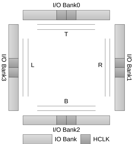
图 3-48 GW1NSE-2C HCLK 示意图
