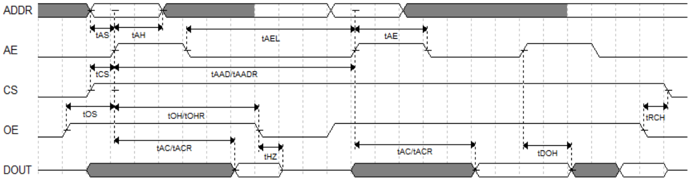
图 4-1 读操作模式
