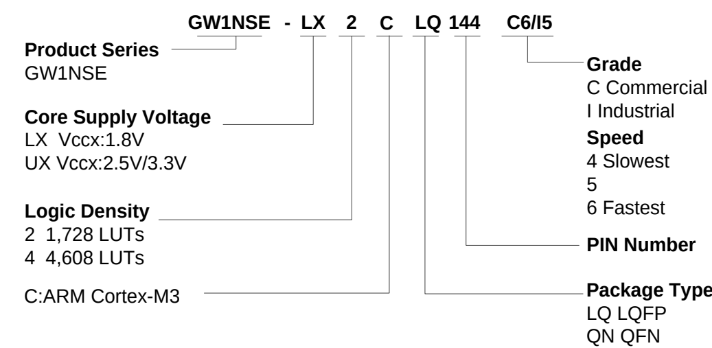
图 5-2 GW1NSE-2C/GW1NSE-4C 器件命名方法 - Production
