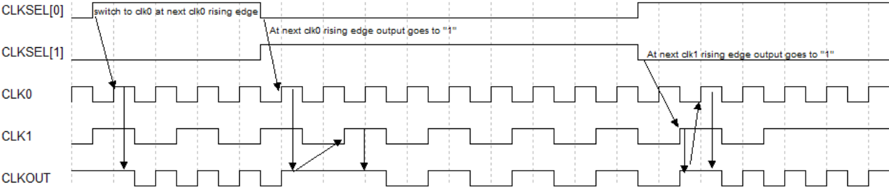
图 3-45 DCS Rising Edge 模式下的时序示意图
