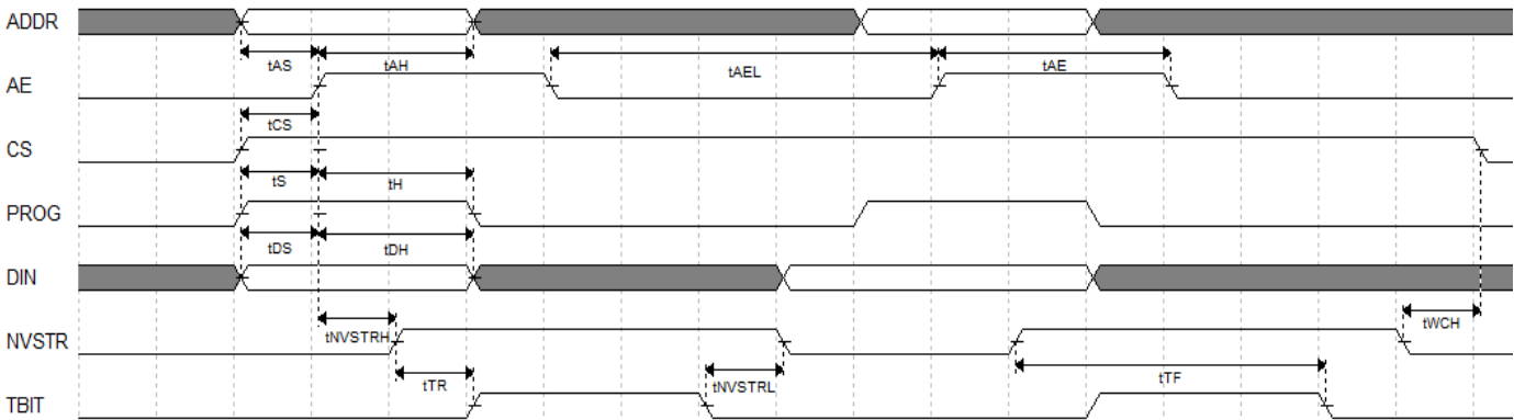
图 4-2 写操作模式
