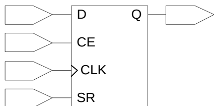
图 3-9 GW1NS 的 I/O 寄存器示意图
