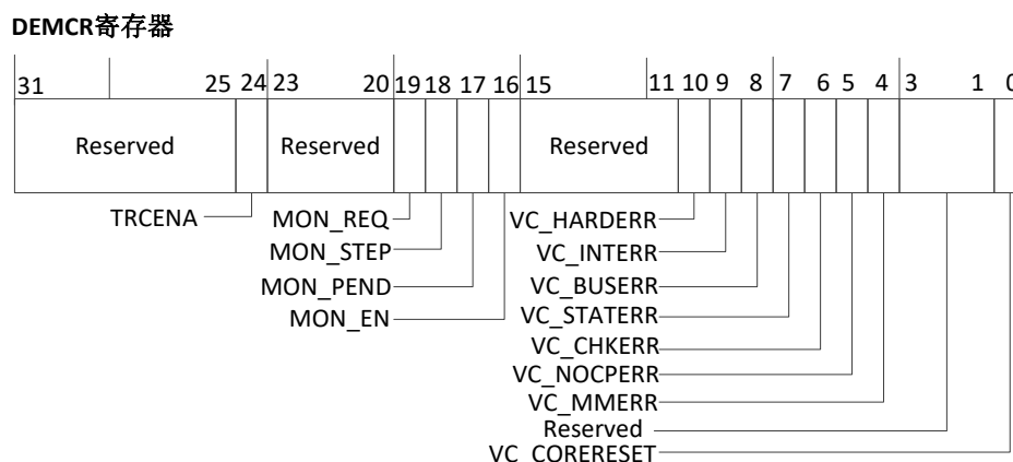
图 3-36 DEMCR 寄存器
