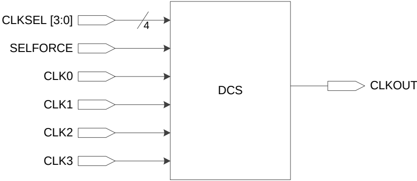
图 3-44 DCS 接口示意图
