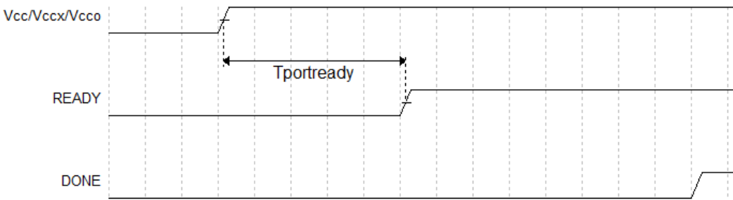
图 4-7 重新上电时序图
