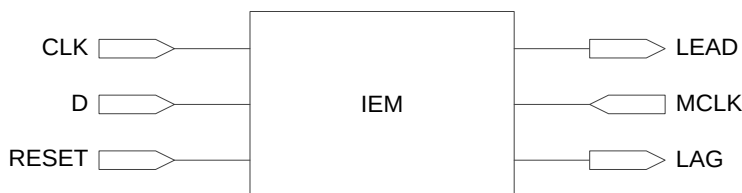
图 3-10 GW1NS 的 IEM 示意图
