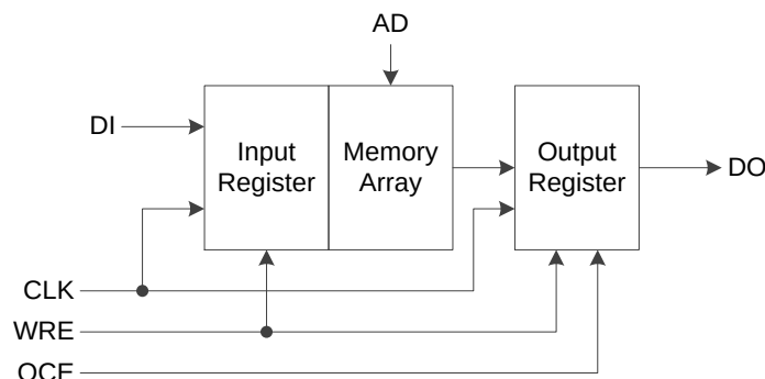
图 3-32 单端口时钟模式
