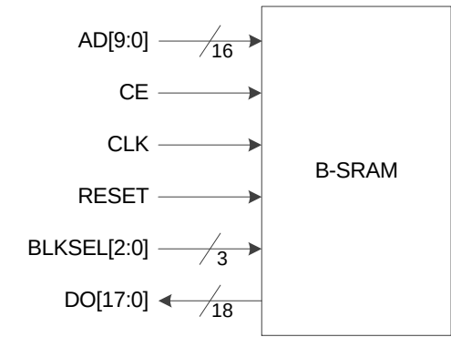
图 3-28 只读模式存储框图
