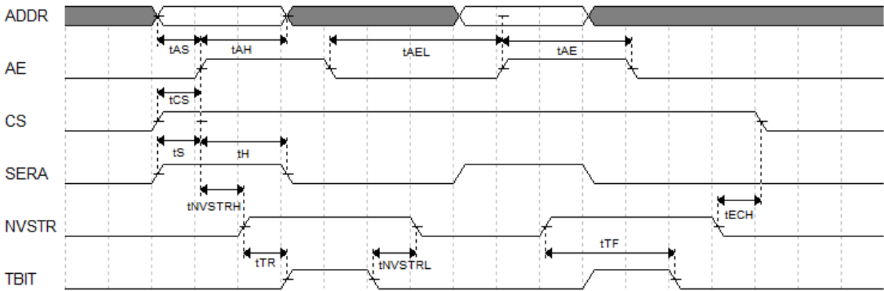
图 4-3 页擦除模式
