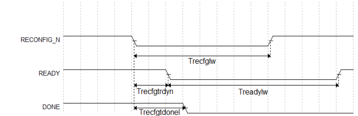
图 4-8 RECONFIG_N 触发时序图
