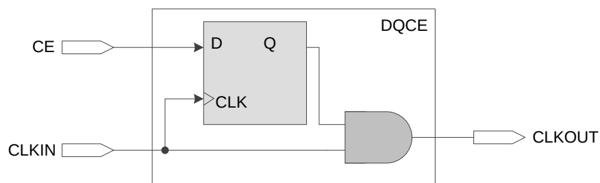
图 3-43 DQCE 结构示意图
