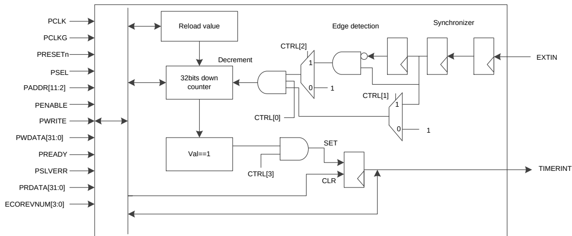
图 3-37 Timer0/ Timer1 结构框图
