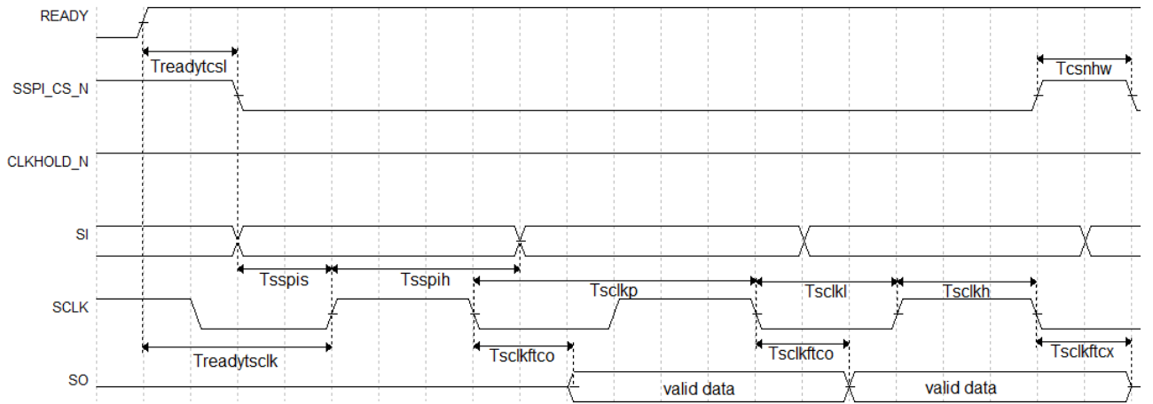
图 4-9 SSPI 编程模式时序图
