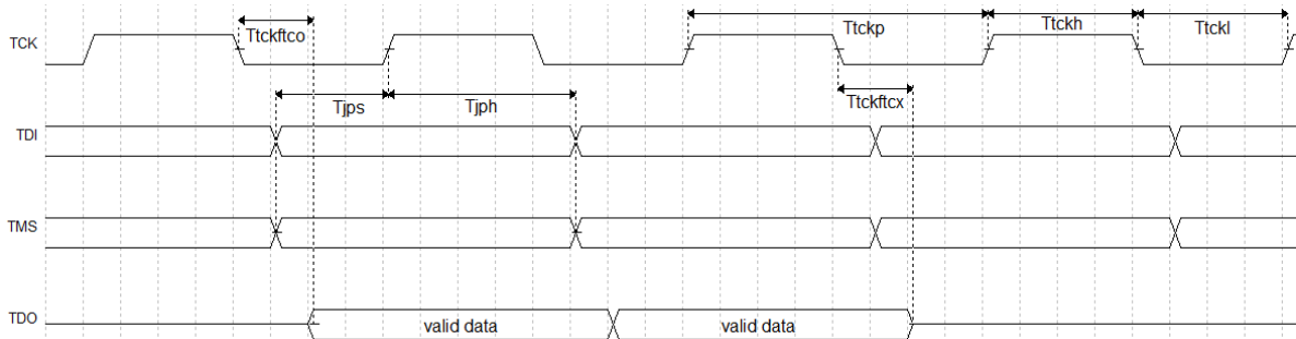
图 4-6 JTAG 编程模式时序示意图
