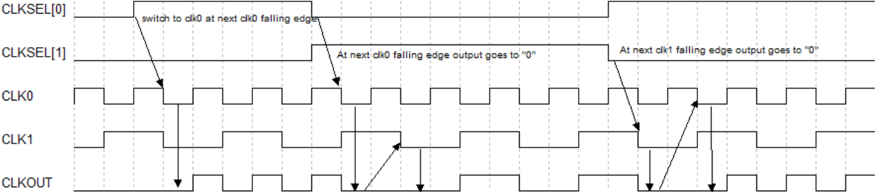
图 3-46 DCS Falling Edge 模式下的时序示意图
