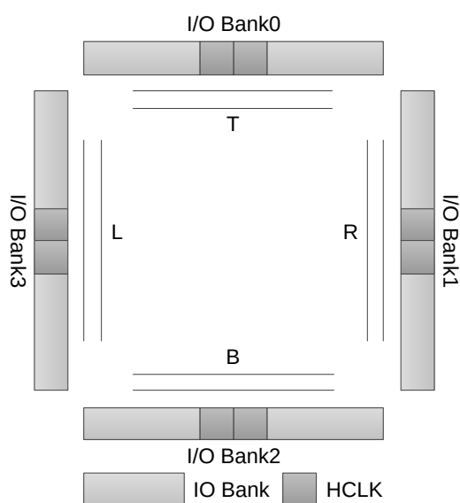
图 3-41 GW1NSE-2C 时钟资源
