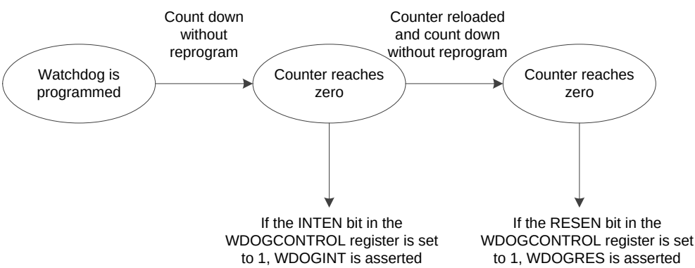
图 3-39 Watchdog 操作方式
