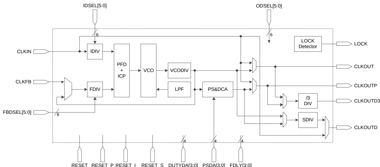
图 3-47 PLL 示意图
