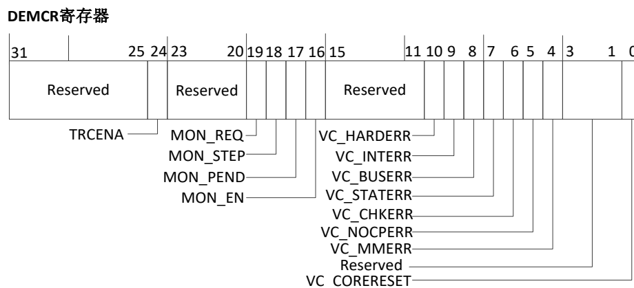
图 3-30 DEMCR 寄存器
