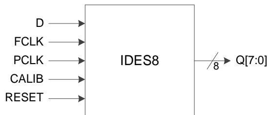
图 3-19 I/O 逻辑的 IDE8 输入示意图
