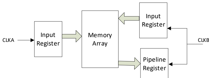
图 3-28 读写时钟模式
