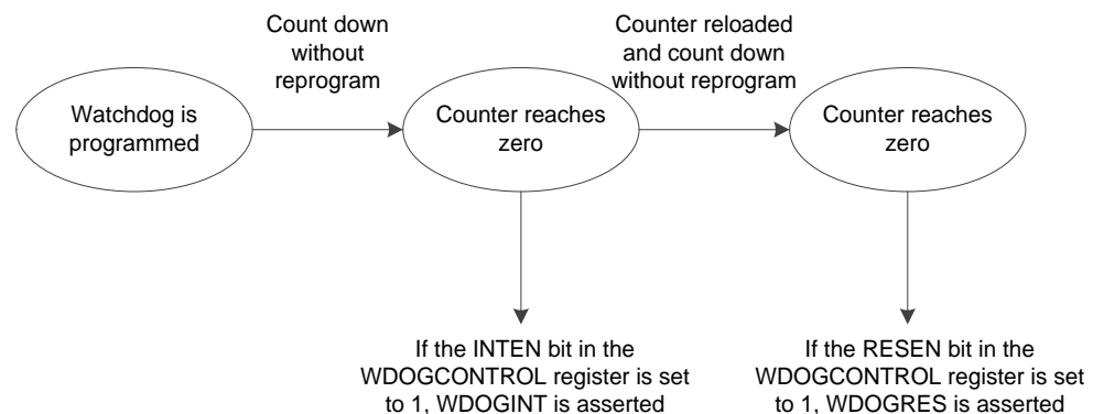
图 3-34 Watchdog 操作方式
