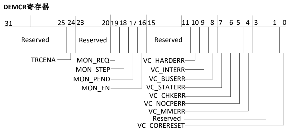
图 3-31 DEMCR 寄存器
