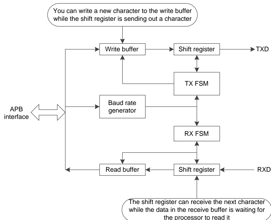
图 3-33 APB UART Buffering
