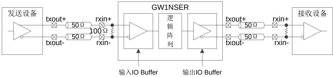
图 2-5 真 LVDS 设计参考框图
