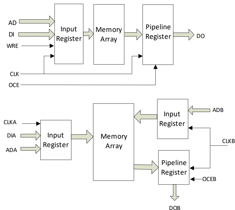
图 2-10 单端口、伪双端口及双端口模式下的流水线模式
