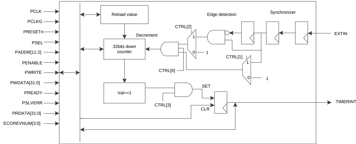
图 2-16 Timer0/Timer1 结构框图
