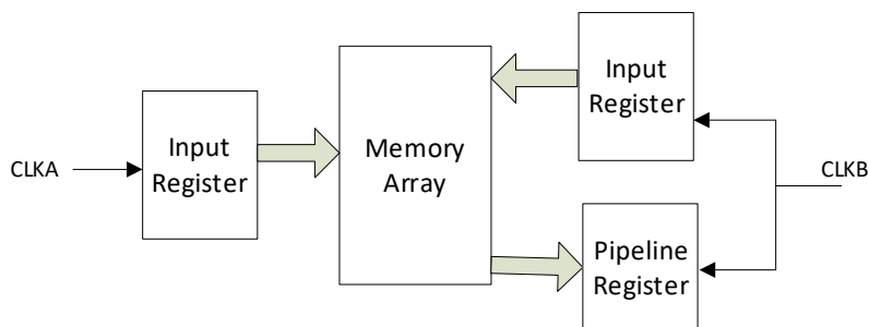
图 2-12 读写时钟模式
