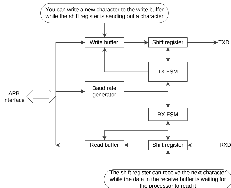
图 2-17 APB UART Buffering
