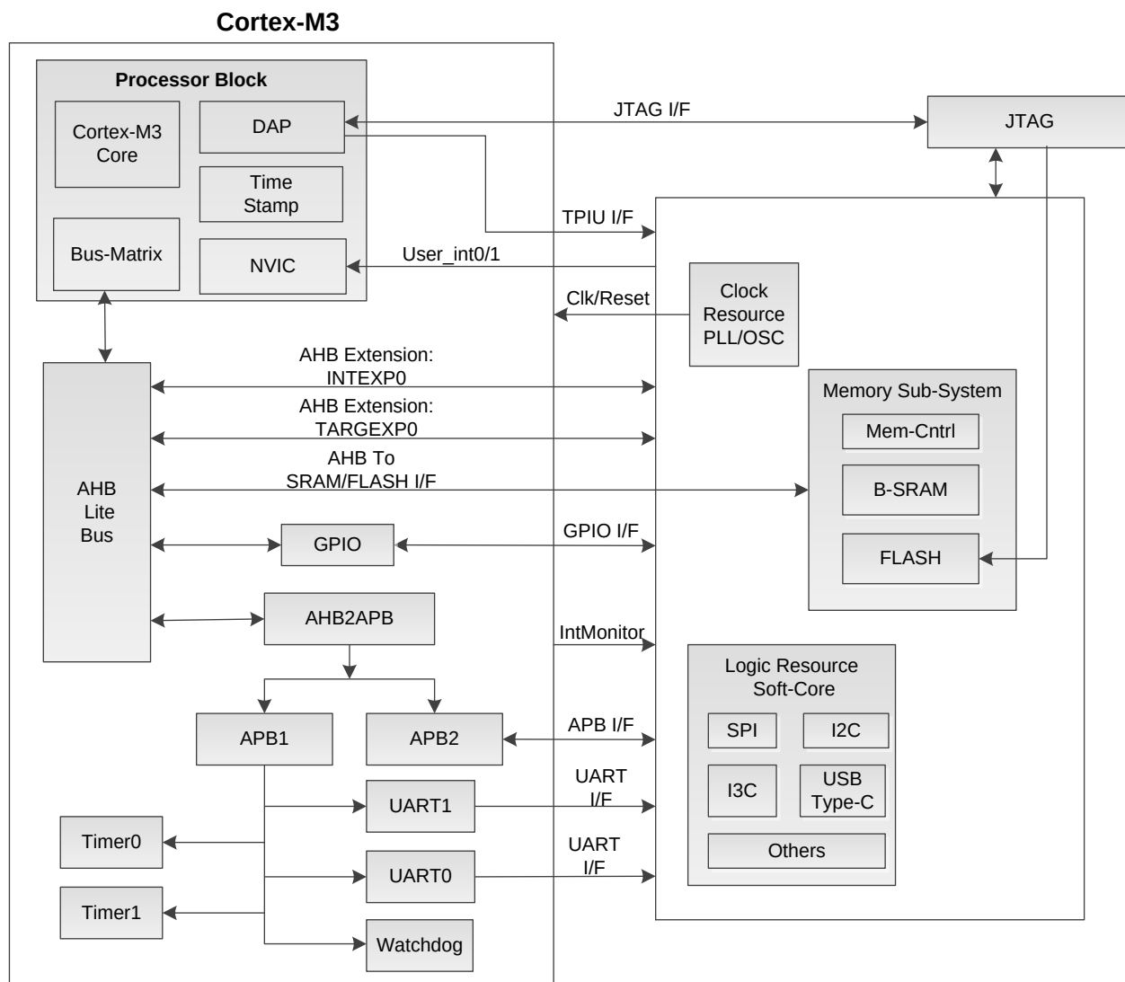
图 2-14 Cortex-M3 结构框图
