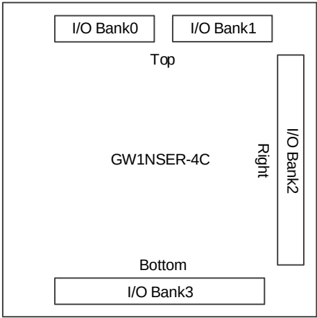
图 2-4 GW1NSER-4C 器件 I/O Bank 分布示意图
