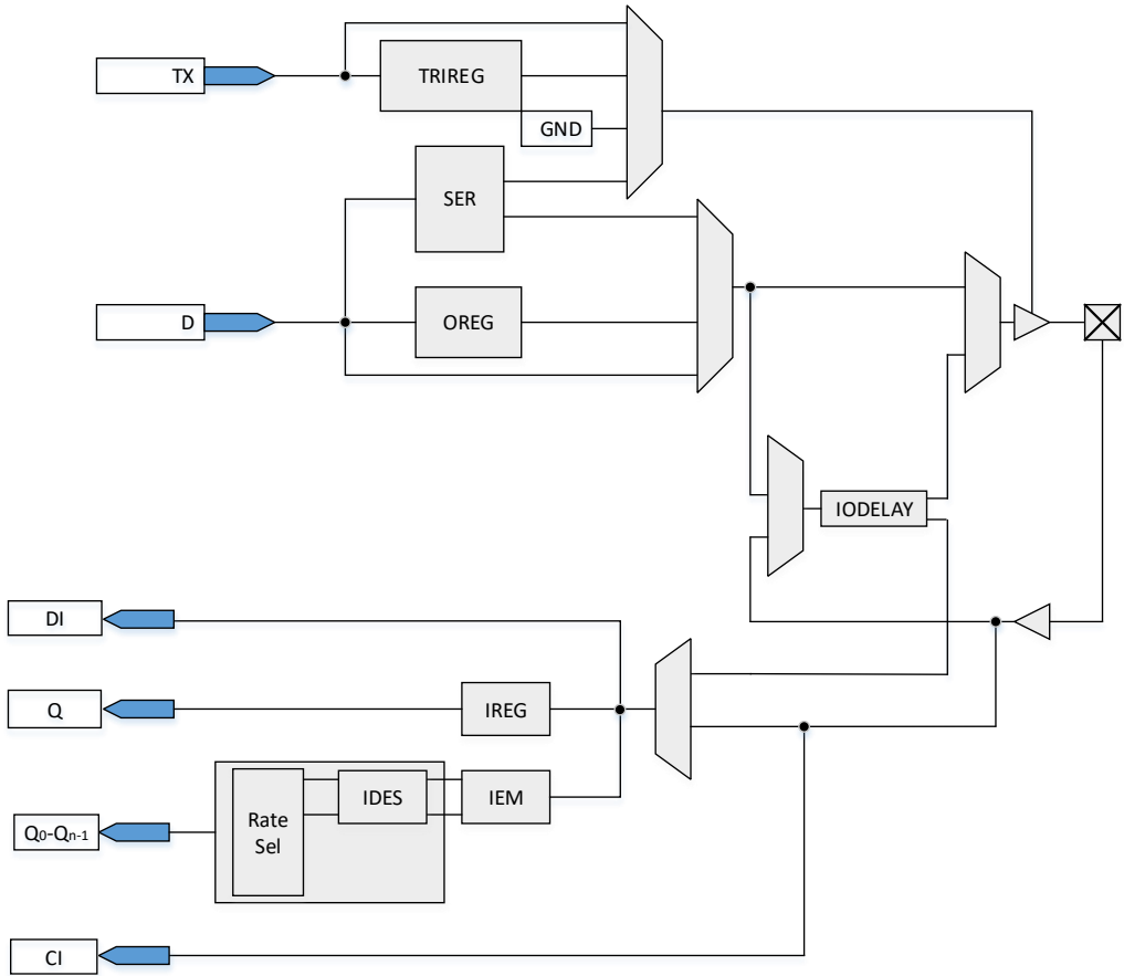
图 2-6 I/O 逻辑输入输出示意图
