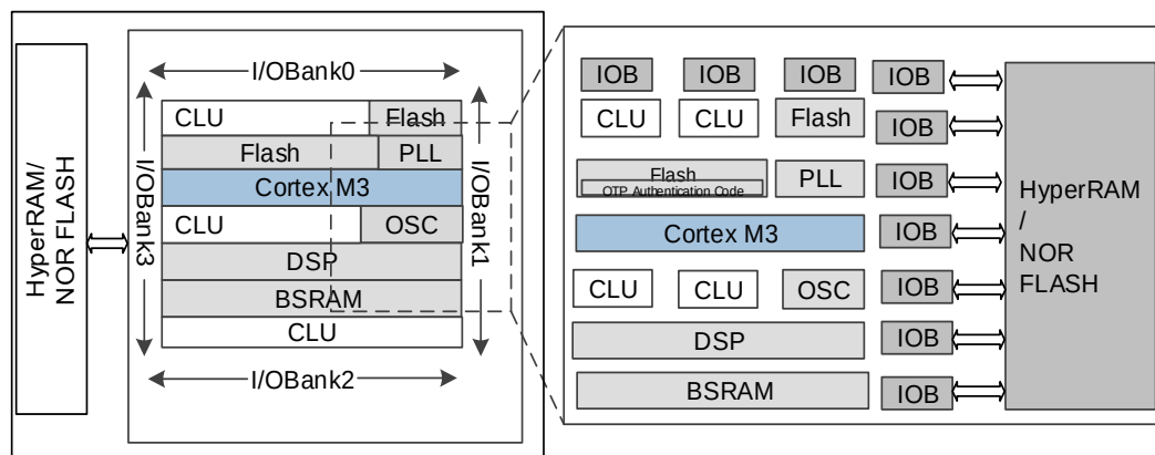
图 2-1 GW1NSER-4C 器件结构示意图
