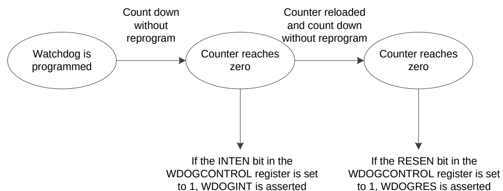
图 2-18 Watchdog 操作方式
