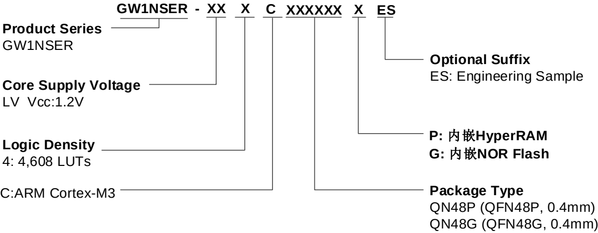
图 4-1 GW1NSER-4C 器件命名方法示例 - ES
