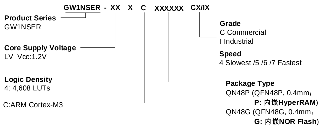
图 4-2 GW1NSER-4C 器件命名方法示例 - Production
