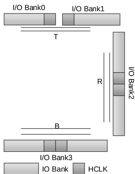
图 2-20 GW1NSER-4C HCLK 示意图
