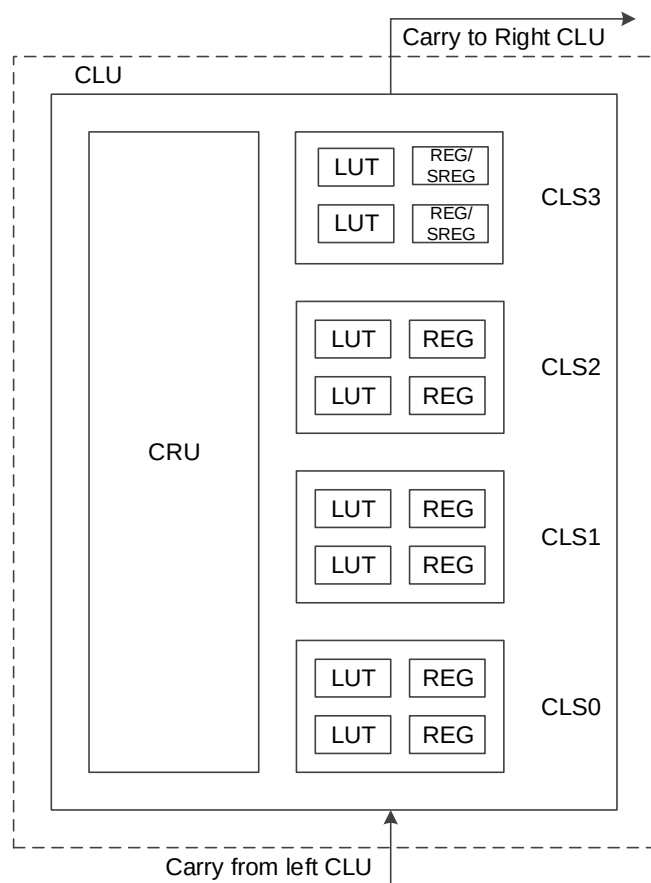
图 2-2 CLU 结构示意图
