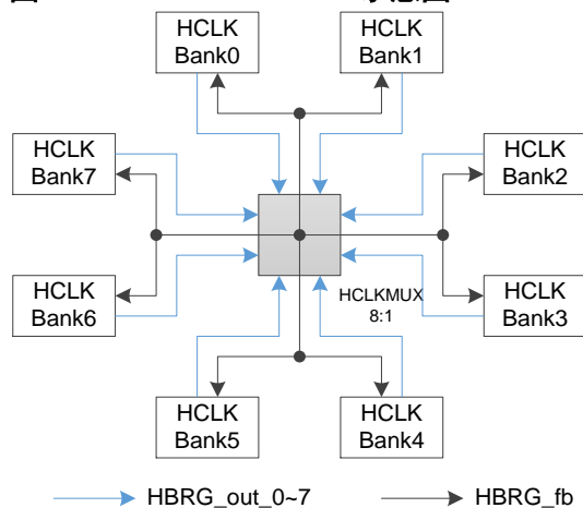
图 3-41 GW2ANR HCLK 示意图
