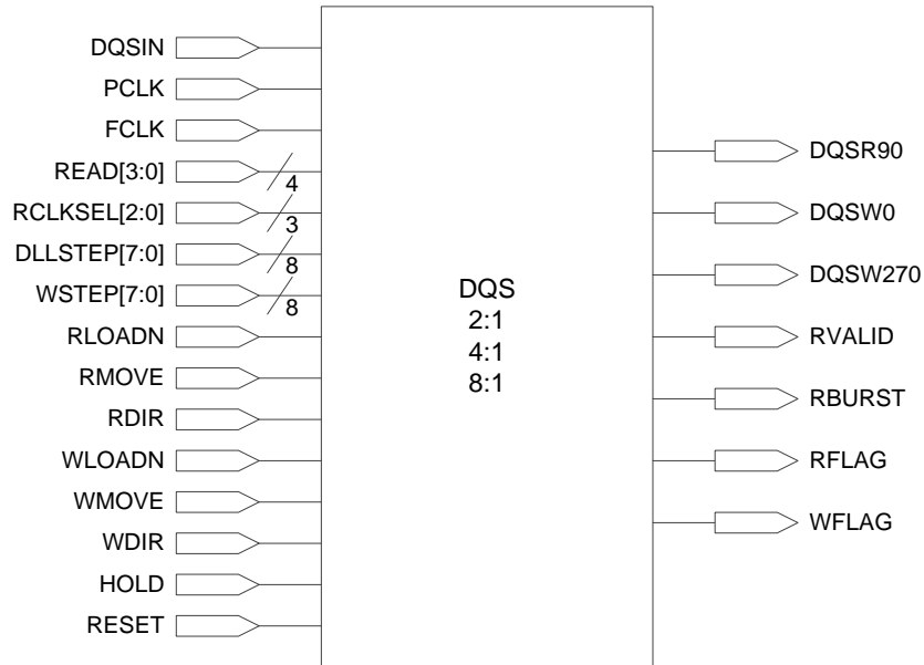
图 3-42 DQS 示意图
