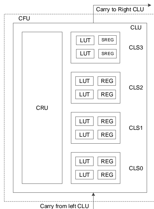
图 3-2 CFU 结构示意图
