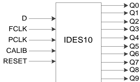
图 3-21 I/O 逻辑的 IDES10 输入示意图
