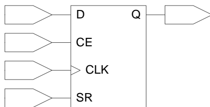
图 3-9 GW2ANR 的 I/O 寄存器示意图
