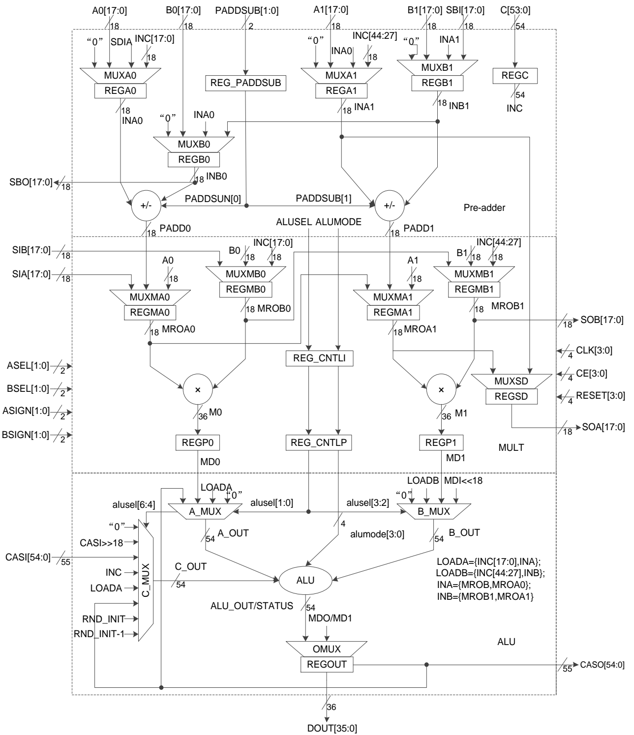
图 3-33 DSP 宏单元
