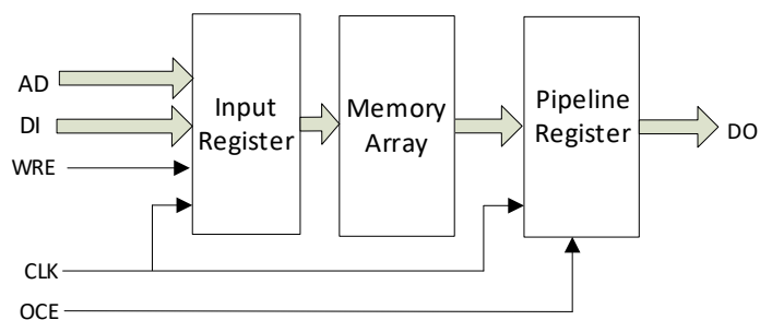
图 3-11 单端口、伪双端口及双端口模式下的流水线模式
