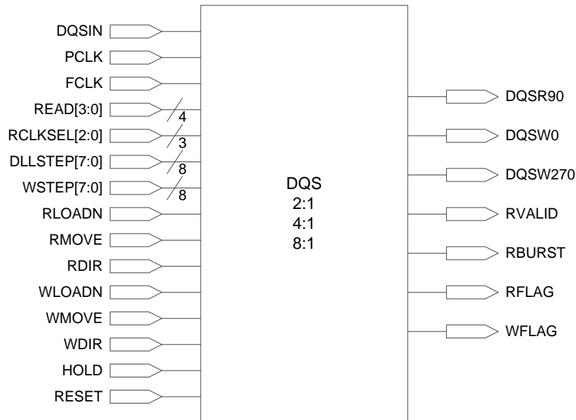
图 3-23 DQS 示意图
