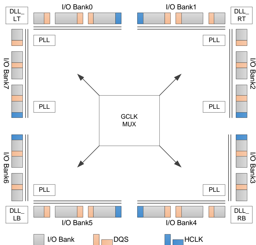
图 3-34 GW2AN-55 时钟资源
