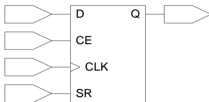
图 3-9 GW2AN-55 的 I/O 寄存器示意图
