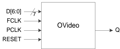
图 3-18 I/O 逻辑的 OVideo 输出示意图
