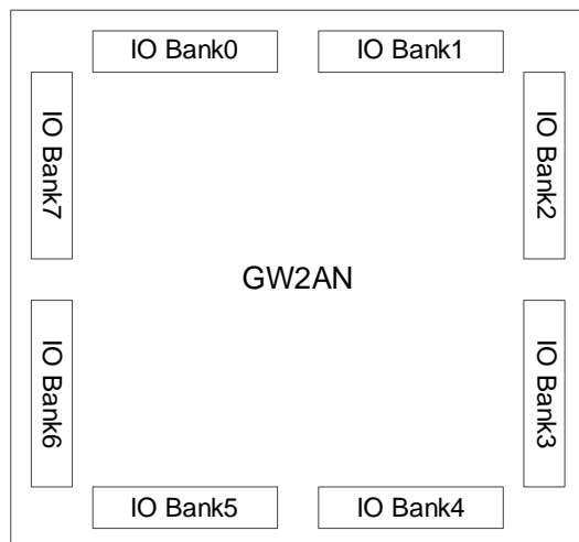
图 3-5 GW2AN-55 的 I/O Bank 分布示意图
