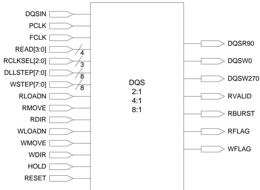
图 3-42 DQS 示意图
