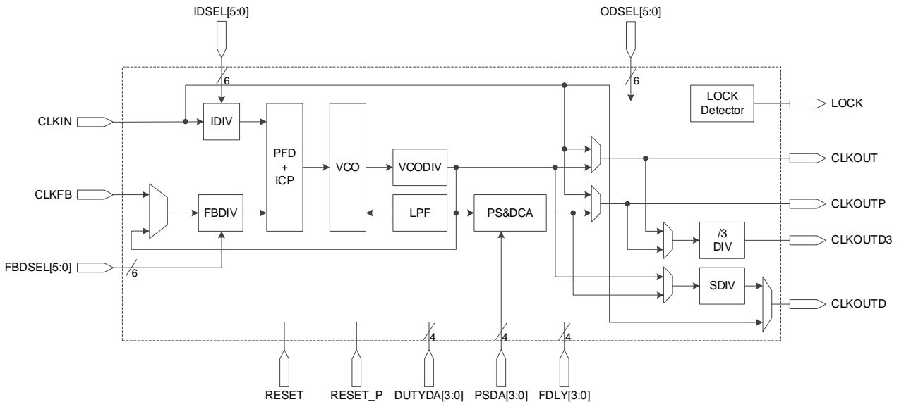
图 3-40 PLL 示意图
