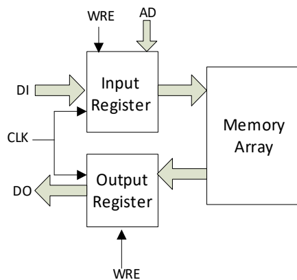
图 3-32 单端口时钟模式
