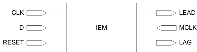
图 3-10 GW2AN-55 的 IEM 示意图
