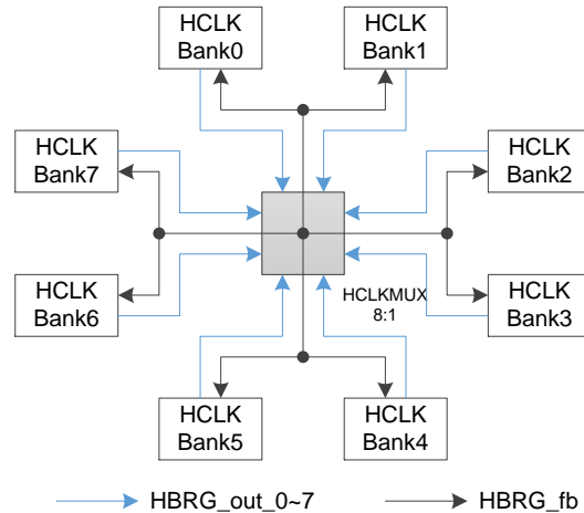
图 3-41 GW2AN-55 HCLK 示意图
