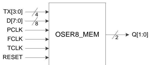
图 3-28 IO 逻辑的 OSER8_MEM 输出示意图
