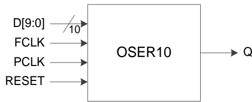
图 3-22 I/O 逻辑的 OSER10 输出示意图
