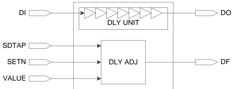
图 3-8 IODELAY 示意图
