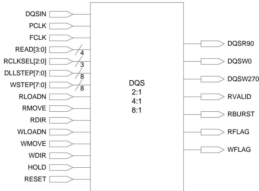
图 3-42 DQS 示意图
