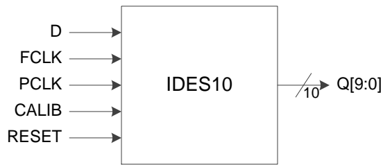
图 3-21 I/O 逻辑的 IDER10 输入示意图
