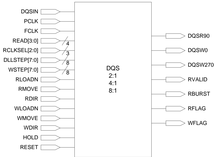
图 3-42 DQS 示意图
