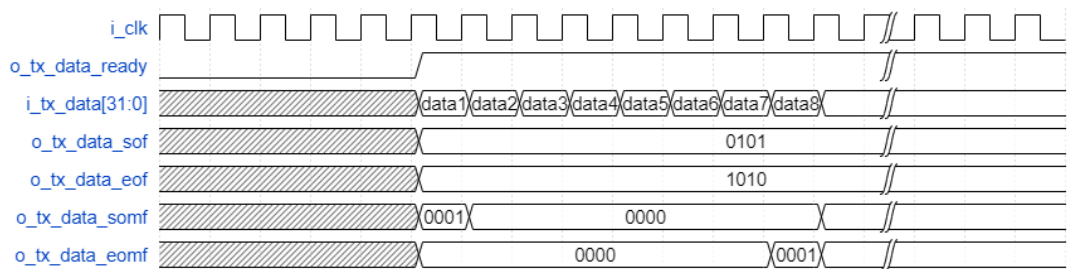
图 3-7 F=2 K=32 时，发射数据接口时序
