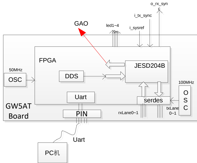
图 6-3 平台框图
