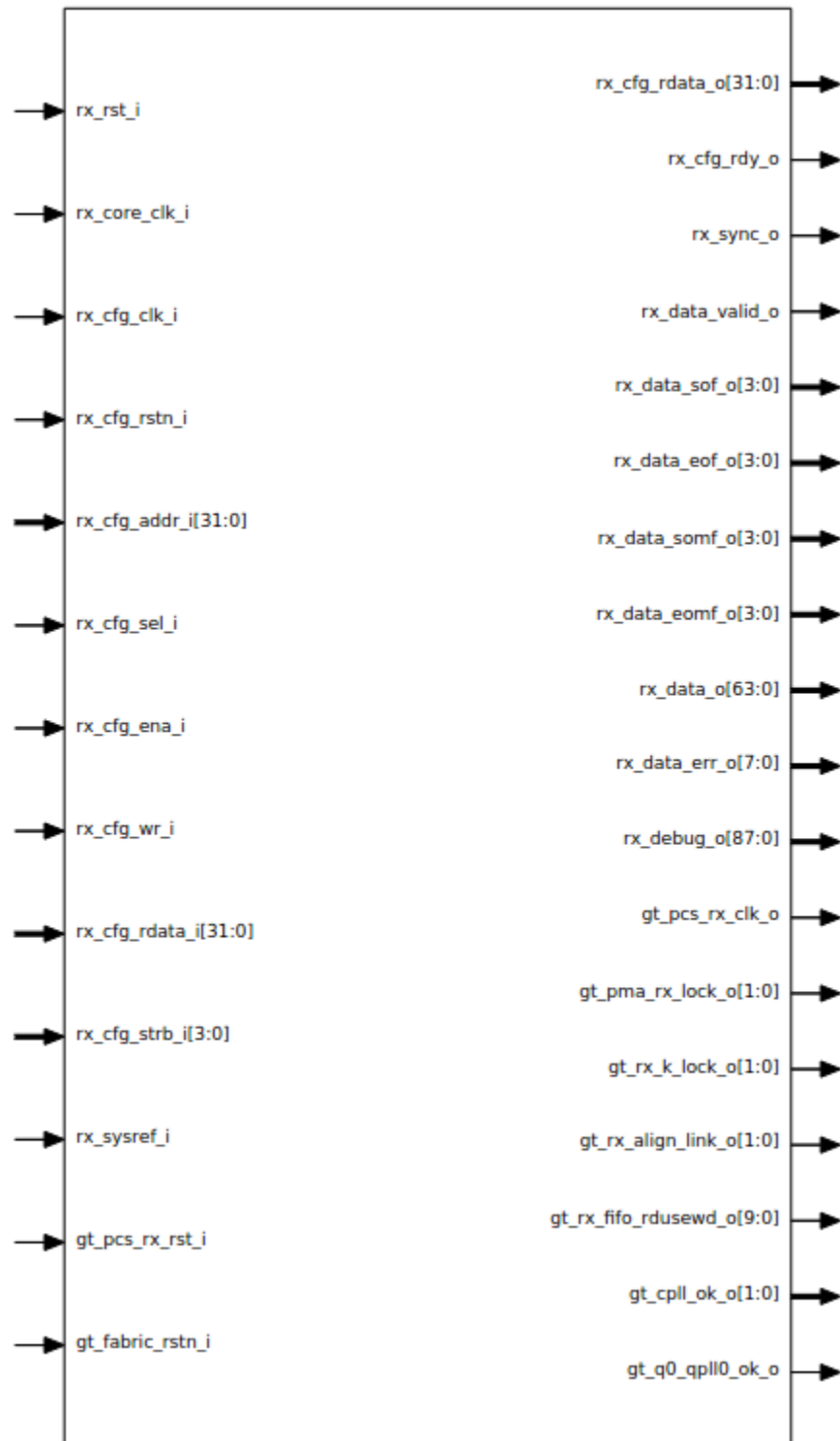
图 3-4 Gowin JESD204B IP RX 端口示意图
