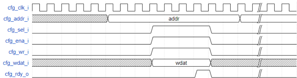
图 3-5 配置接口写时序图
