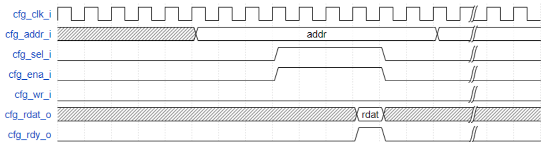
图 3-6 配置接口读时序图
