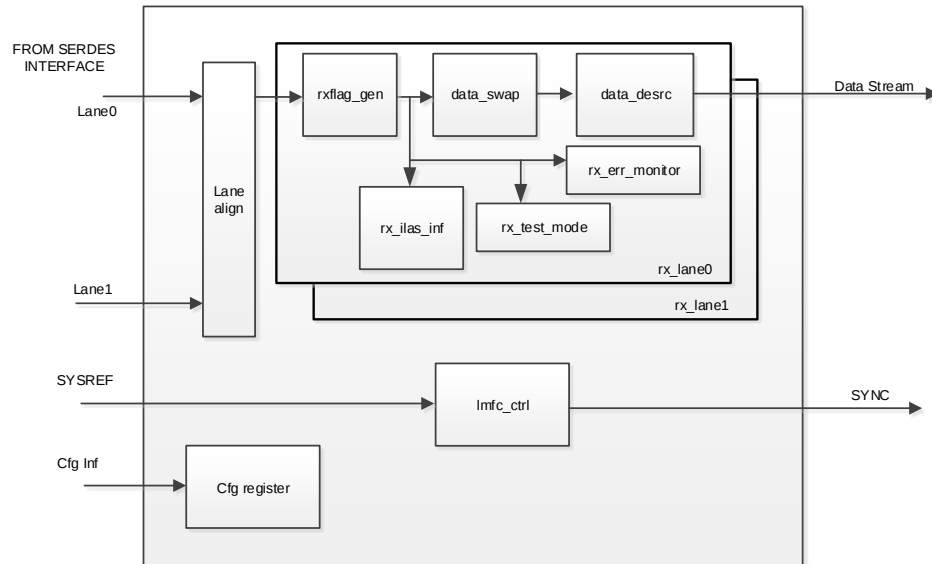
图 3-2 接收器结构图
