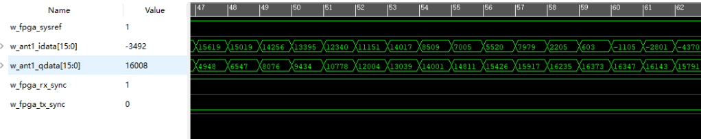
图 6-8 抓取 DDS 数据
