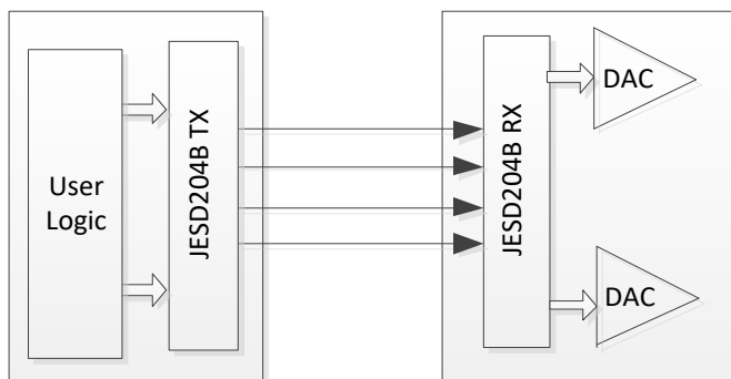
图 6-2 FPGA 与 DAC 的连接
