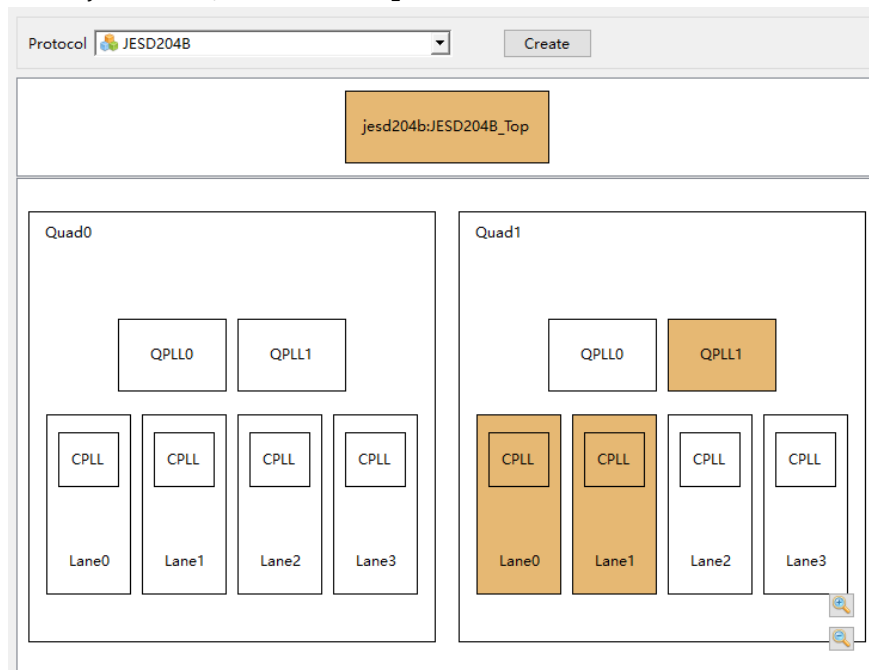
图 5-4 jesd204b: JESD204B_Top
