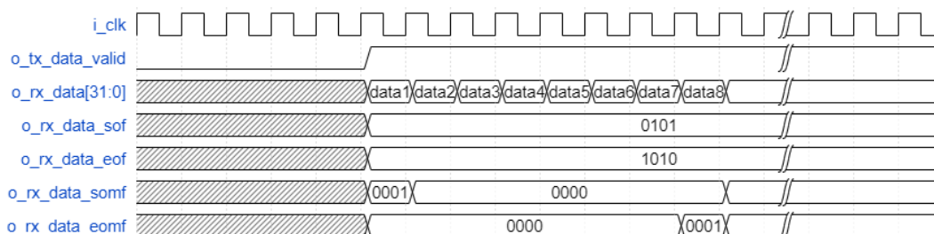
图 3-8 F=2 K=32 时，接收数据接口时序
