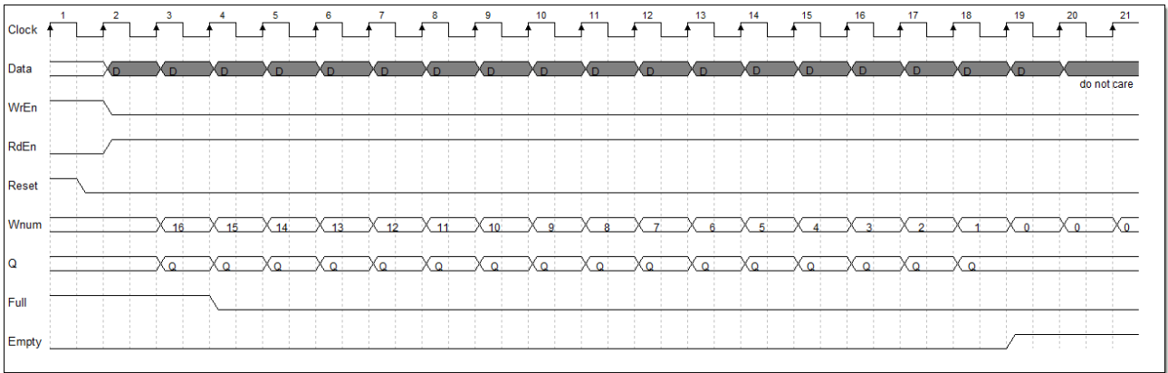
图 4-6 读操作示例
