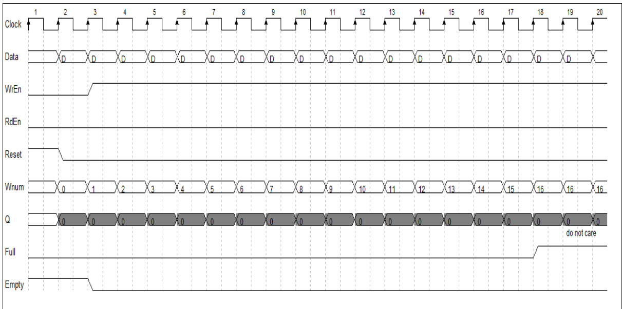
图 4-5 写操作示例
