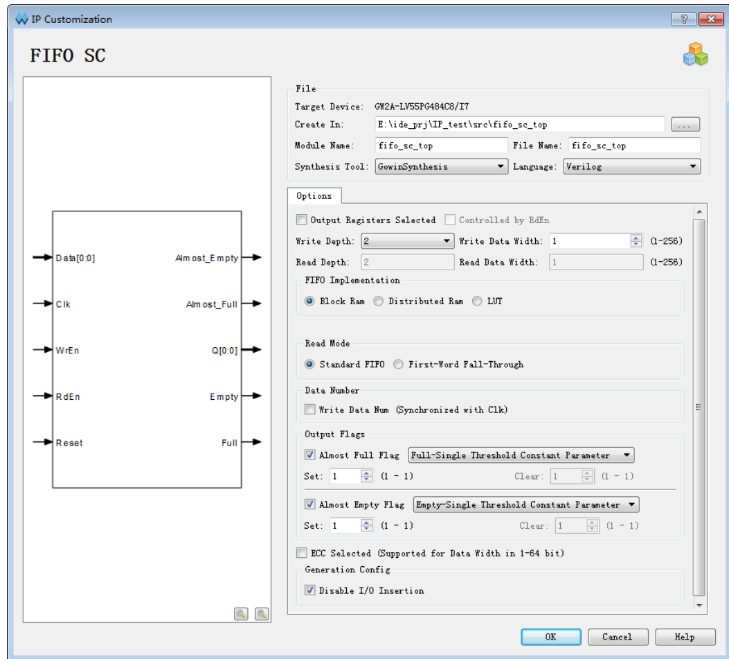
图 5-2 FIFO_SC IP 配置页面
