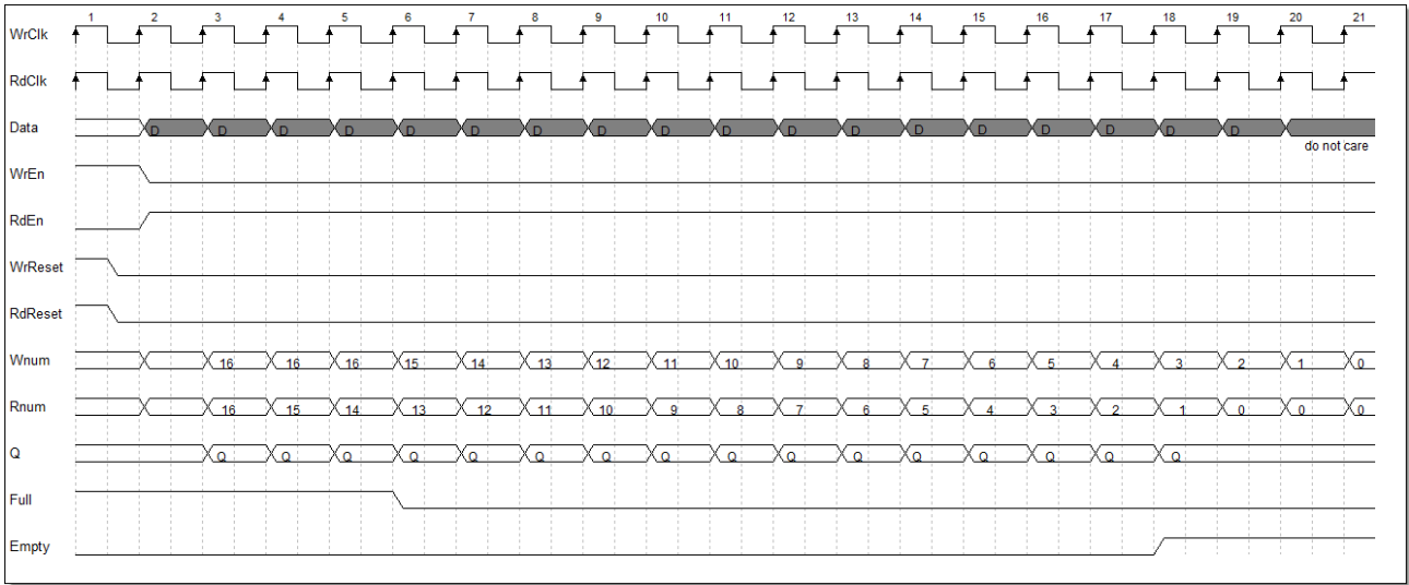
图 4-2 读操作示例
