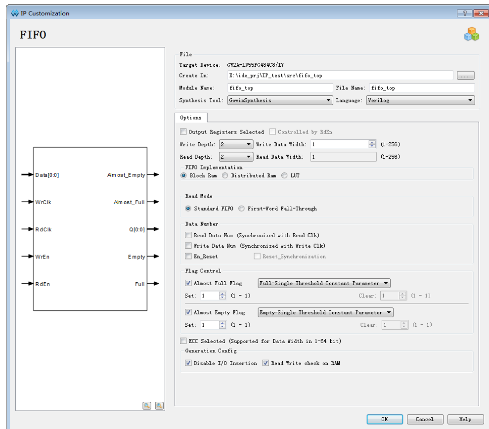
图 5-1 FIFO IP 配置界面
