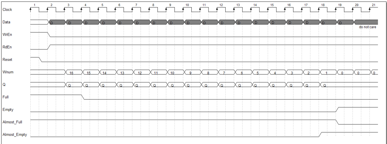
图 4-8 FIFO 空标志和将空标志时序图
