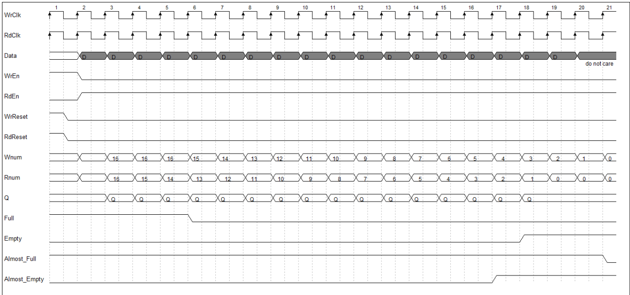
图 4-4 FIFO 空标志和将空标志时序图
