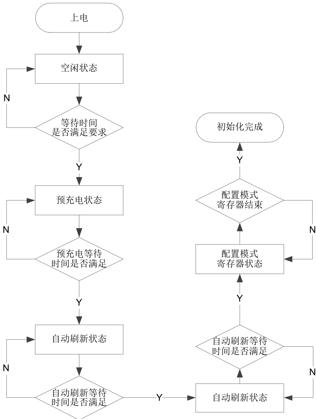
图 5-3 初始化流程图
