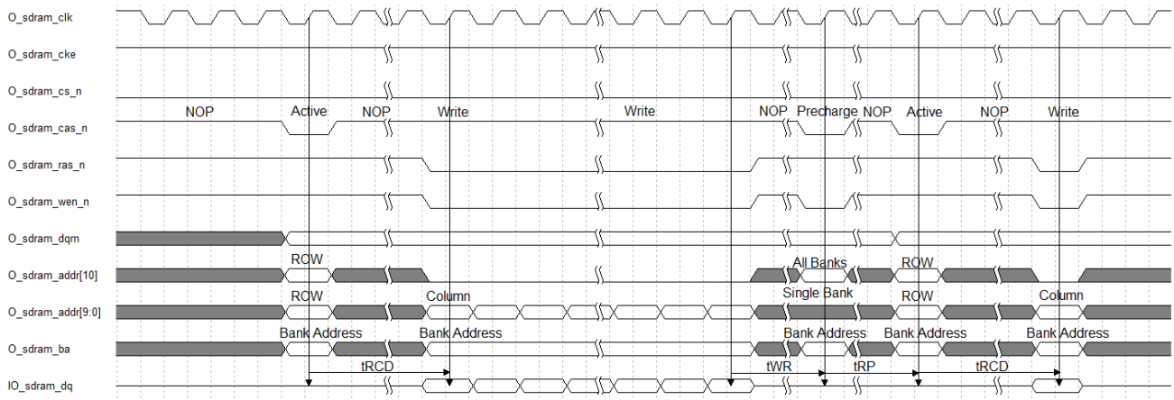
图 7-5 SDRAM 写操作
