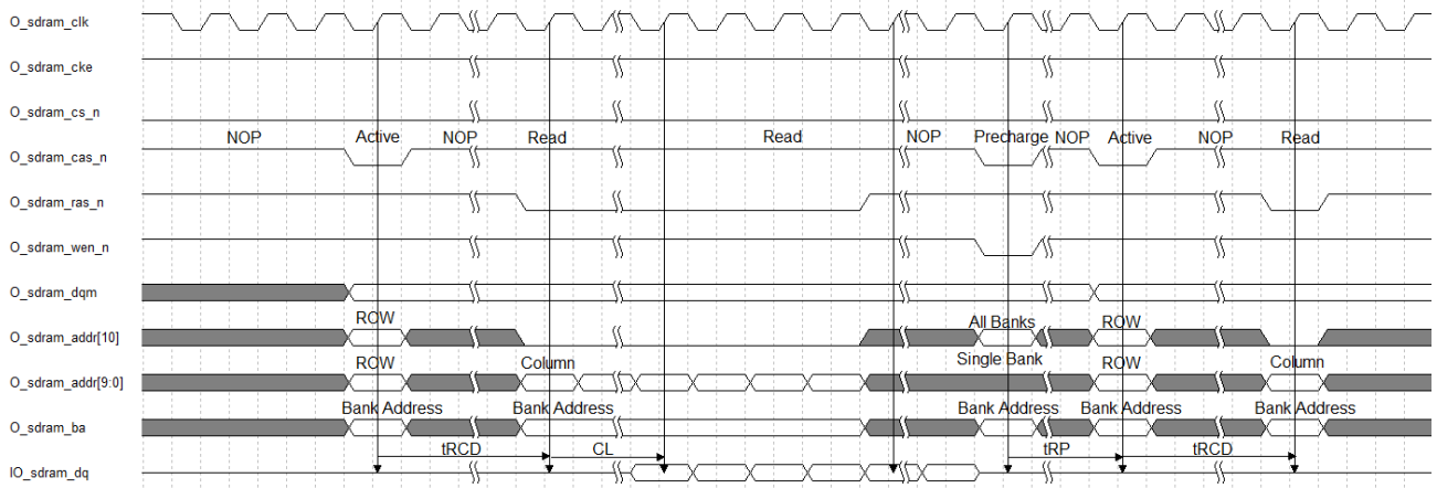
图 7-4 SDRAM 读操作
