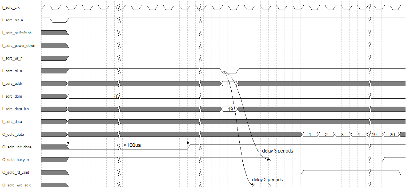
图 7-1 用户侧接口读操作
