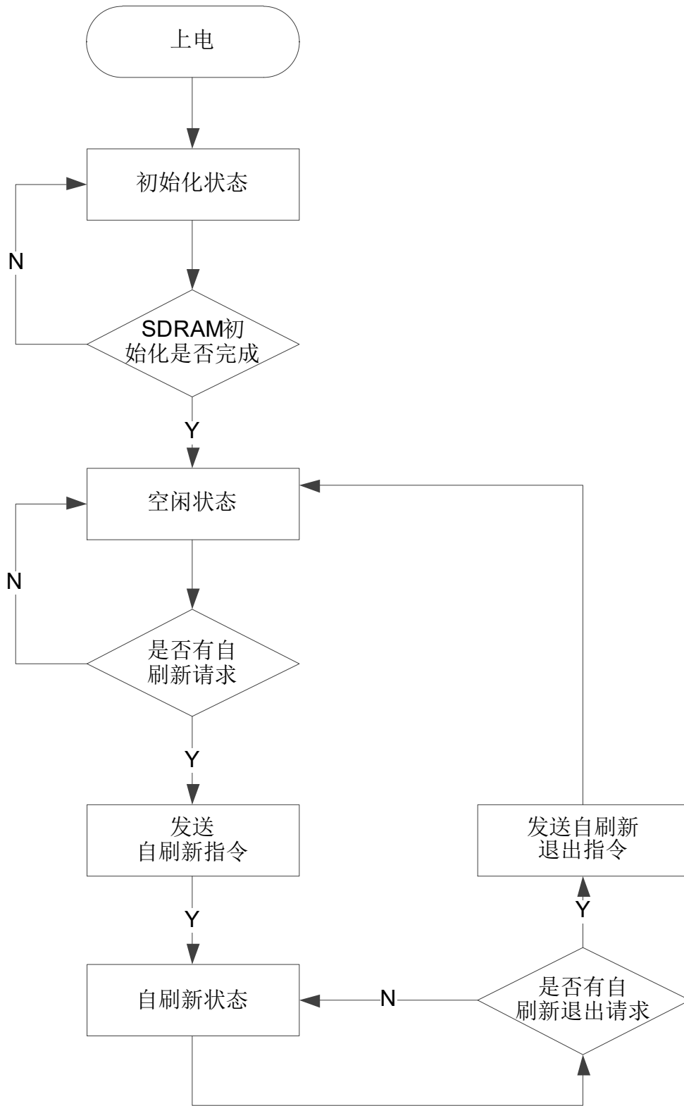
图 5-4 自刷新流程图
