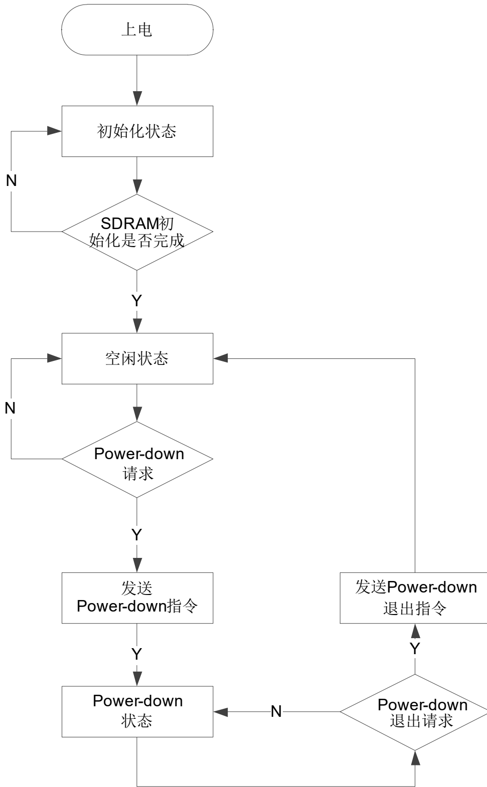
图 5-5 Power-down 流程图
