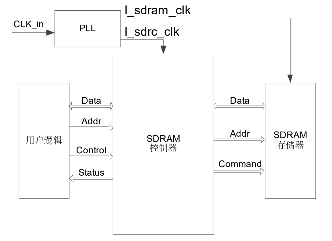
图 6-1 应用框图
