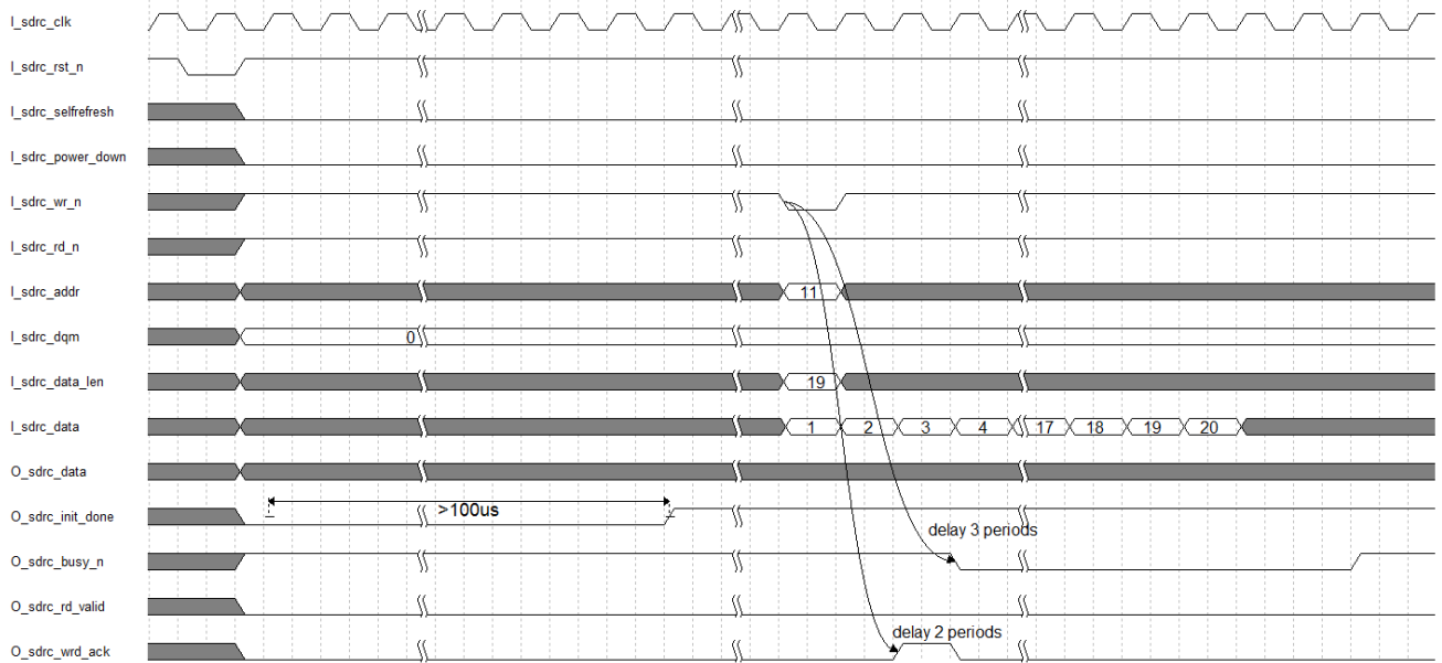
图 7-2 用户侧接口写操作
