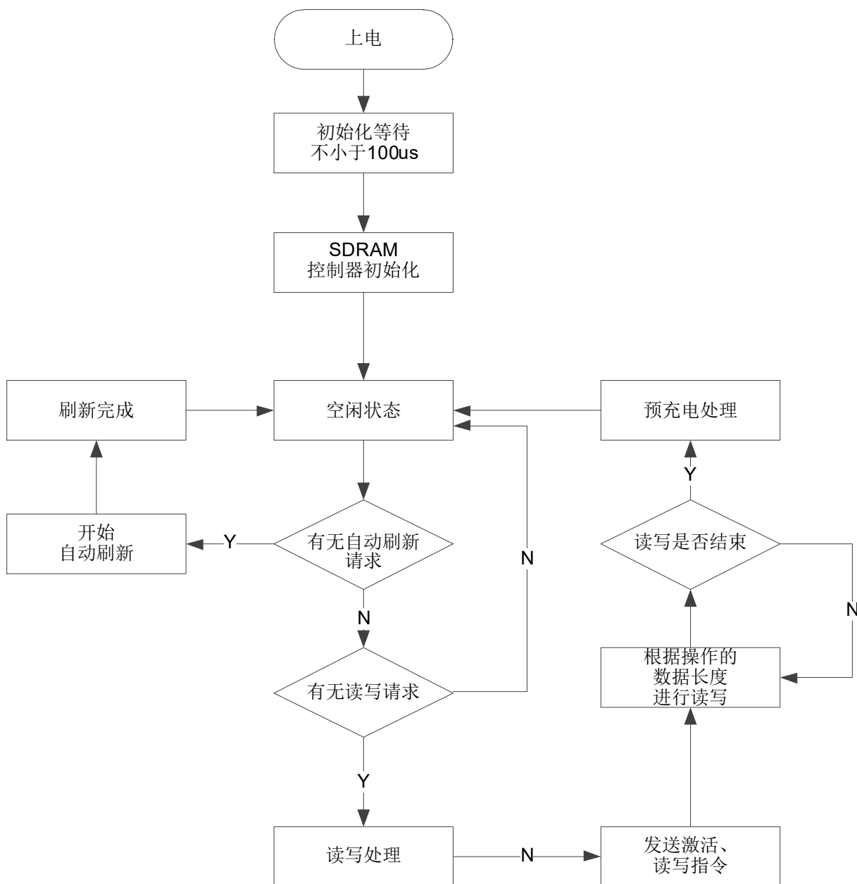
图 5-2 读写工作流程
