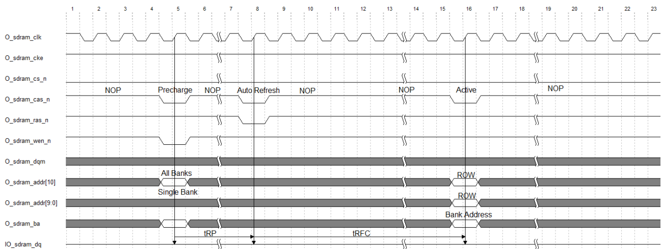
图 7-6 SDRAM 自动刷新
