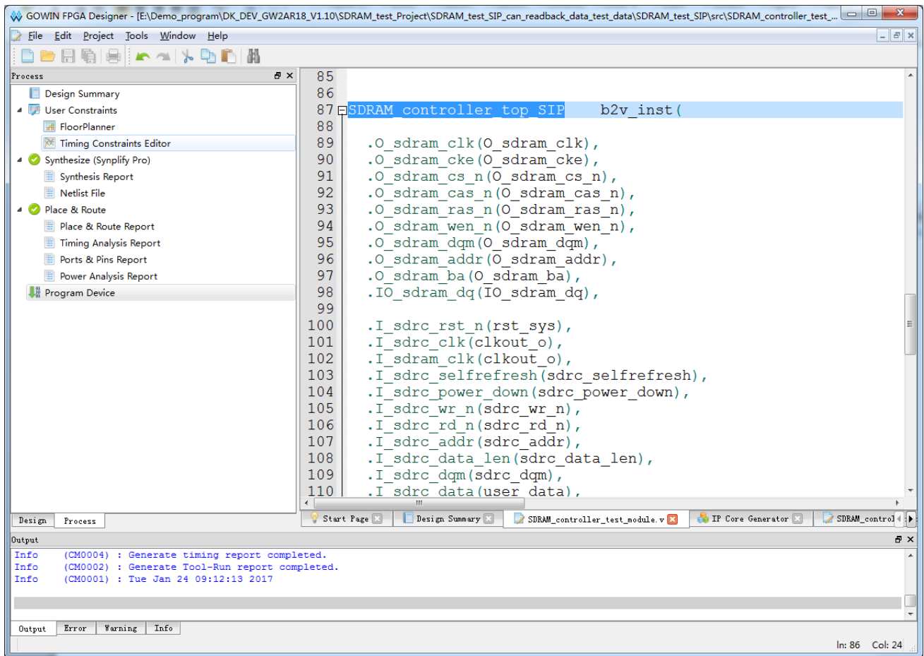
图 6-5 例化 SDRAM_controller_top_SIP
