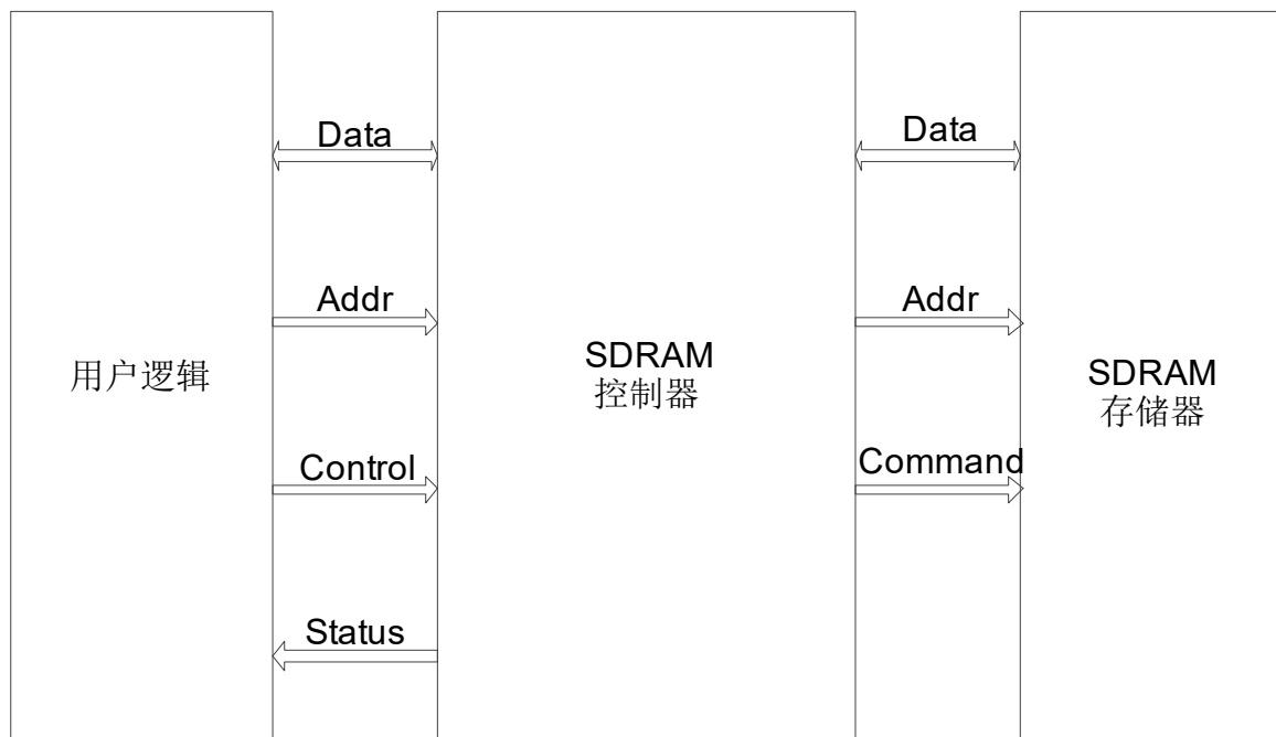
图 3-1 系统框图
