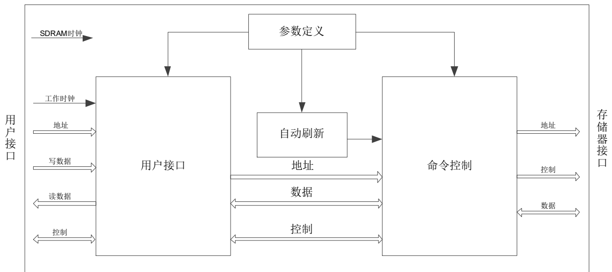
图 5-1 实现框图
