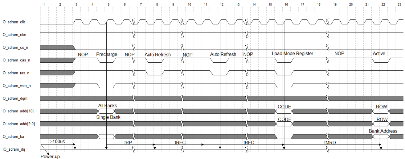
图 7-3 SDRAM 初始化
