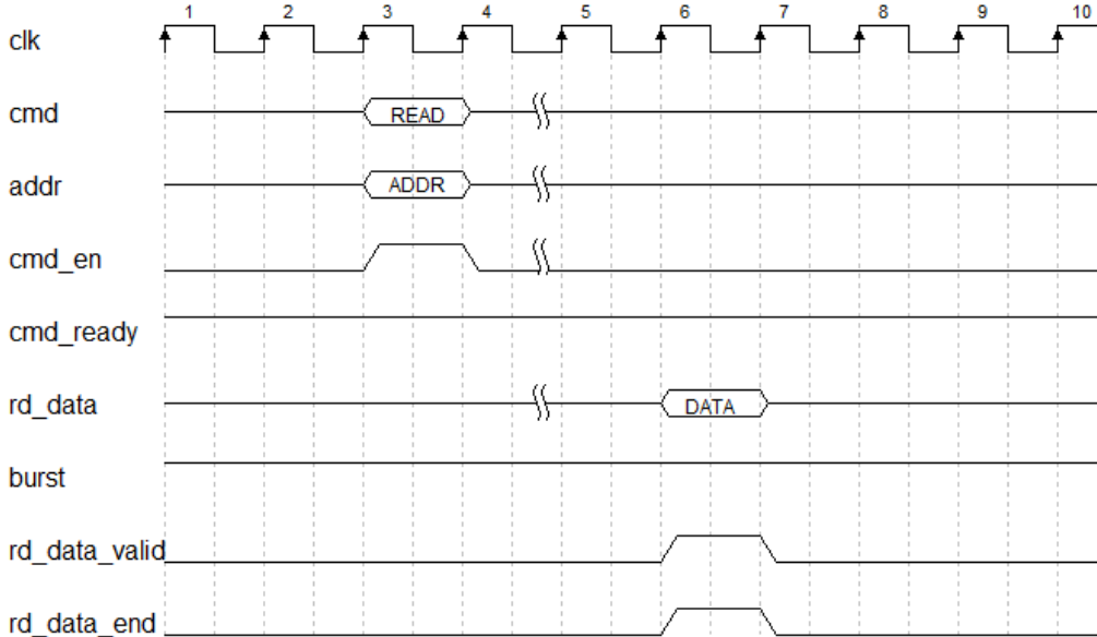
图 4-14 突发长度为 BL4 时读数据时序图
