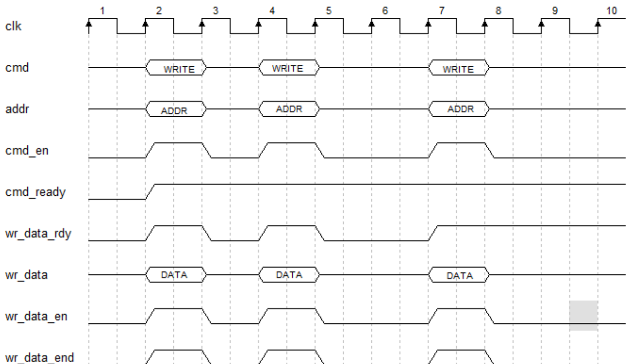
图 4-7 写数据端口时序图
