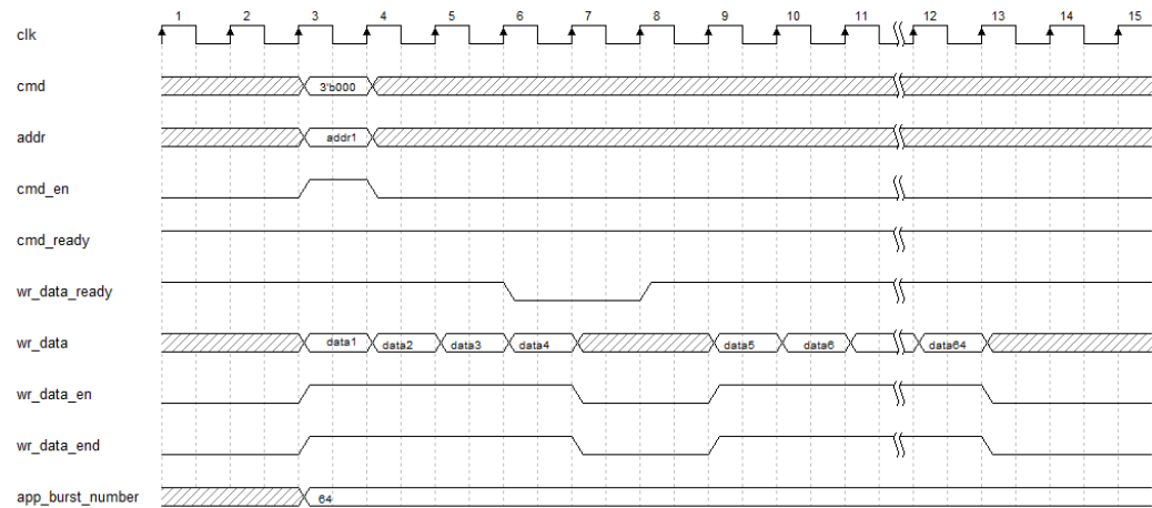
图 4-12 连续突发模式下，写数据时序图
