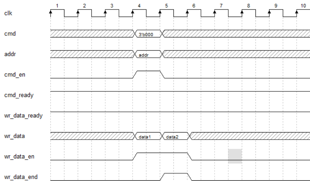
图 4-10 时钟比例 1:2, Burst_Mode=BL8, 写数据时序图
