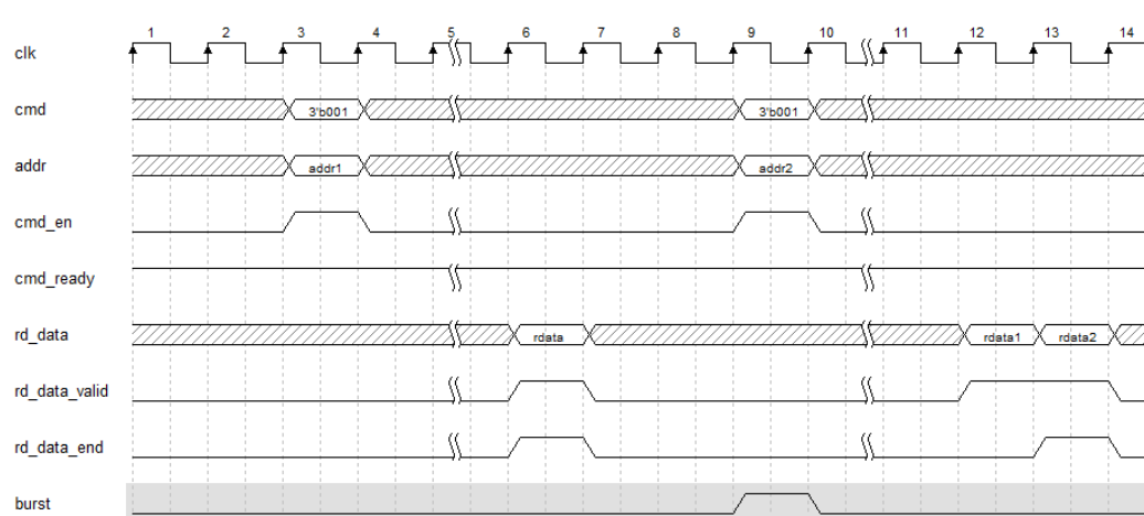
图 4-15 时钟比例 1:2, Burst_Mode=OTF, 读数据时序图
