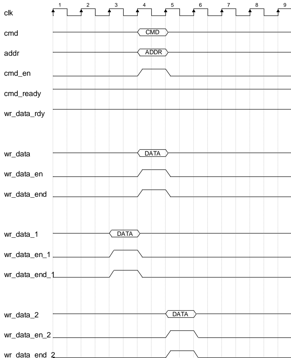
图 4-8 cmd 与数据位置关系图
