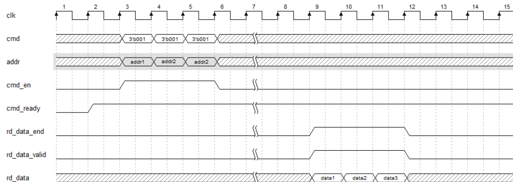
图 4-17 时钟比例 1:4，非连续突发读数据时序图
