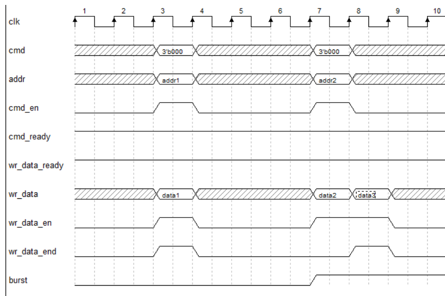
图 4-11 时钟比例 1:2, Burst_Mode=OTF, 写数据时序图
