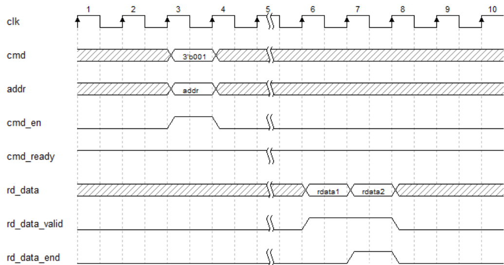
图 4-14 时钟比例 1:2, Burst_Mode=BL8, 读数据时序图
