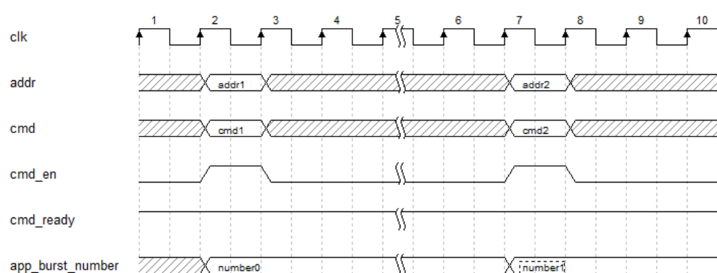
图 4-7 时钟比例 1:4，连续突发模式下命令、地址与使能信号时序图
