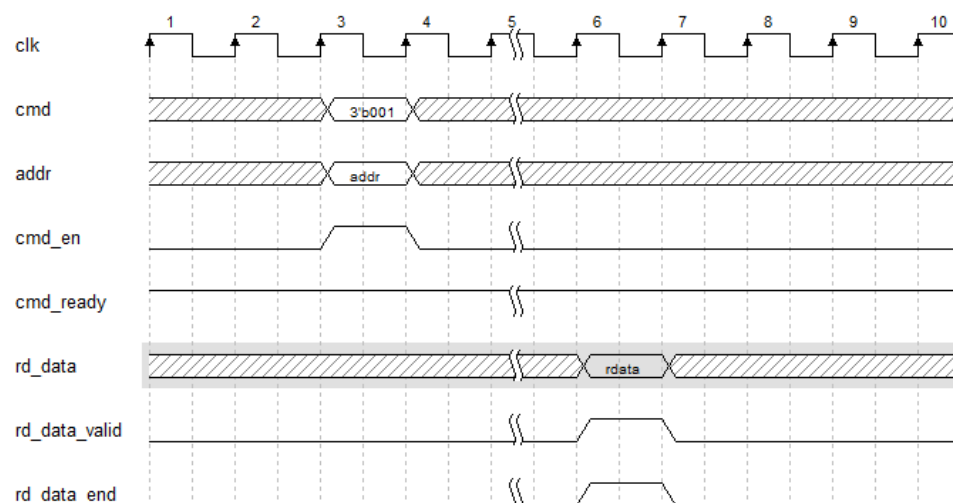
图 4-13 时钟比例 1:2，Burst_Mode=BC4，读数据时序图
