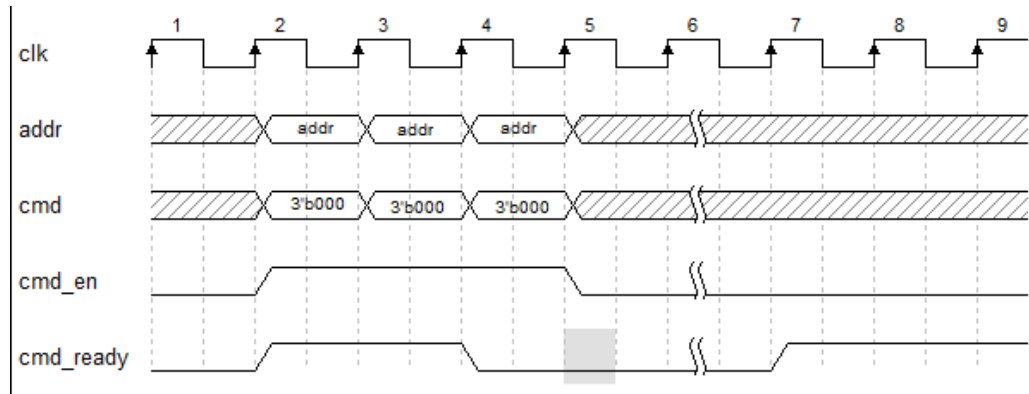
图 4-6 命令、地址与使能信号时序图-b
