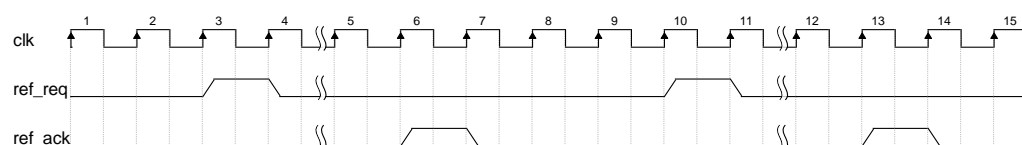
图 4-11 用户刷新时序图
