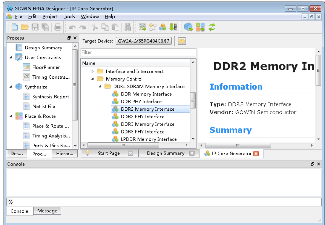
图 7-2 打开 DDR2 Memory Interface IP 核
