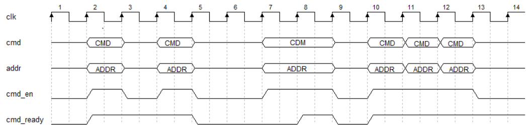
图 4-5 命令、地址与使能信号时序图
