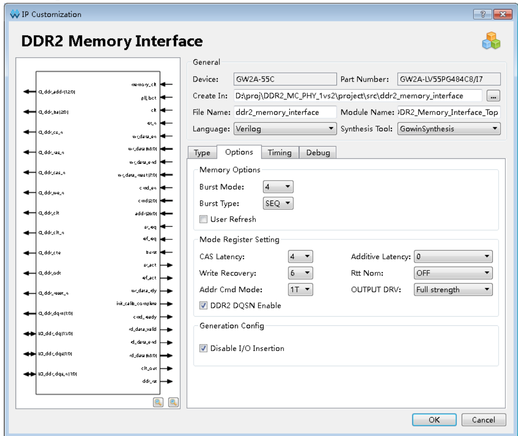
图 7-6 Options 选项卡
