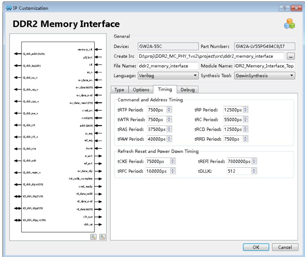
图 7-7 Timing 选项卡
