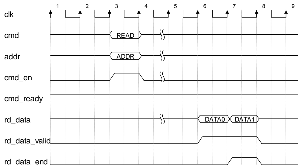
图 4-10 突发长度为 BL8 时读数据时序图
