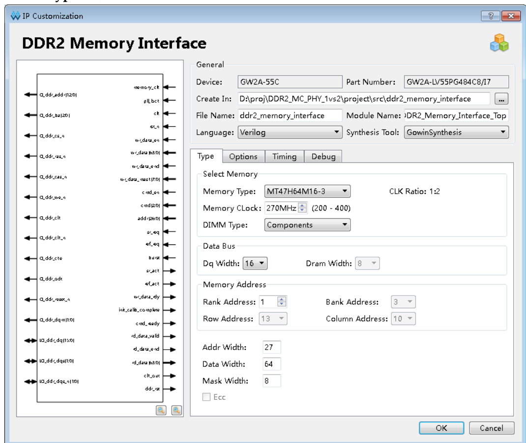
图 7-5 Type 选项卡
