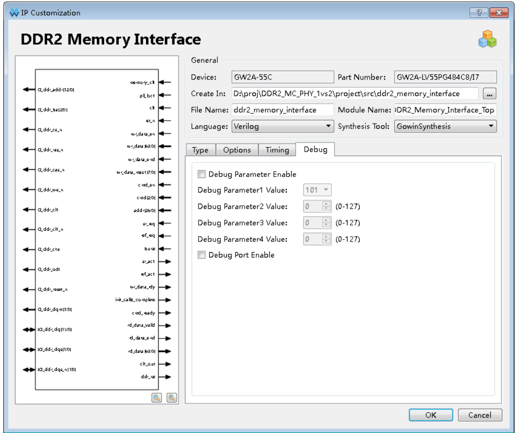
图 7-8 Debug 选项卡
