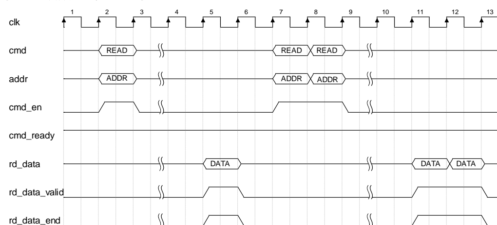
图 4-9 读数据端口时序图
