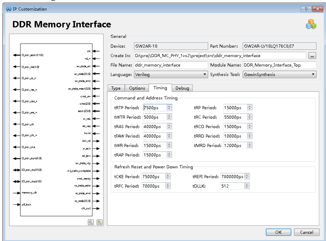
图 6-7 Timing 选项卡
