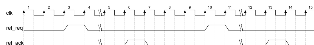
图 3-19 用户刷新时序图
