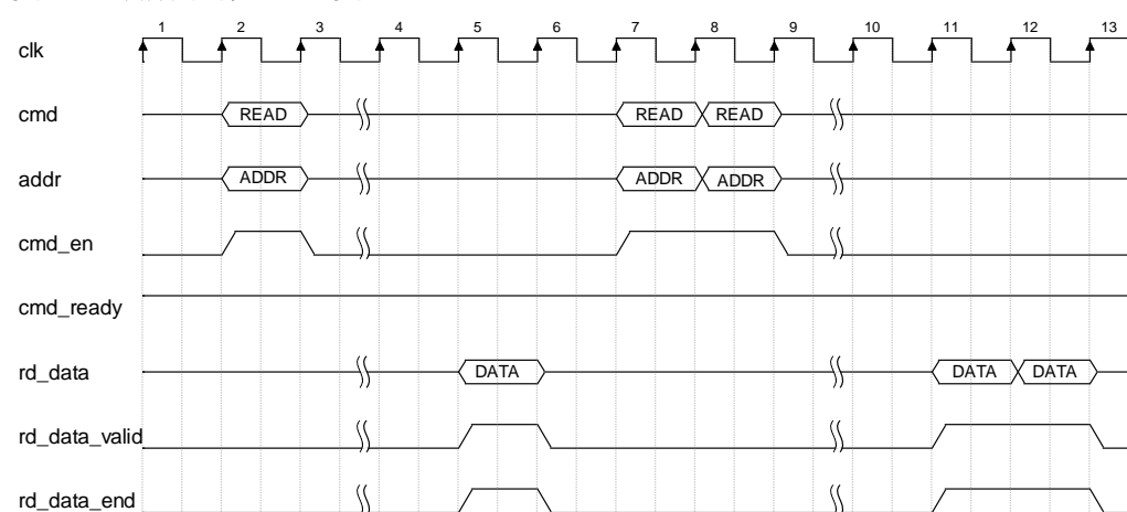
图 3-13 读数据端口时序图
