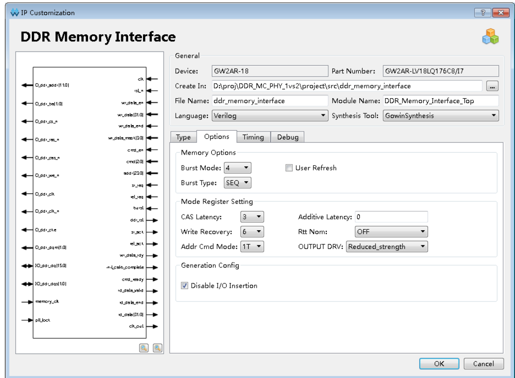
图 6-6 Options 选项卡
