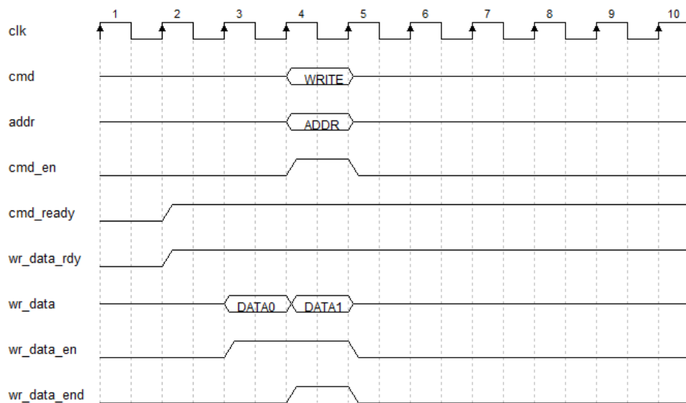
图 3-11 突发长度为 BL4 时写数据时序图
