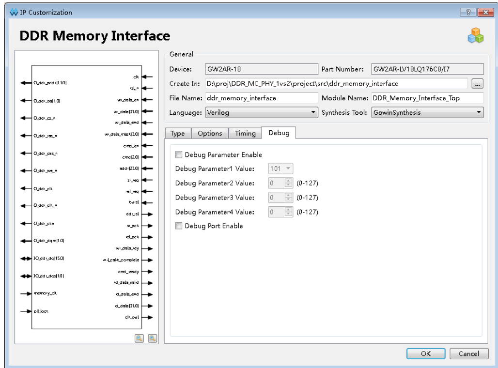
图 6-8 Debug 选项卡
