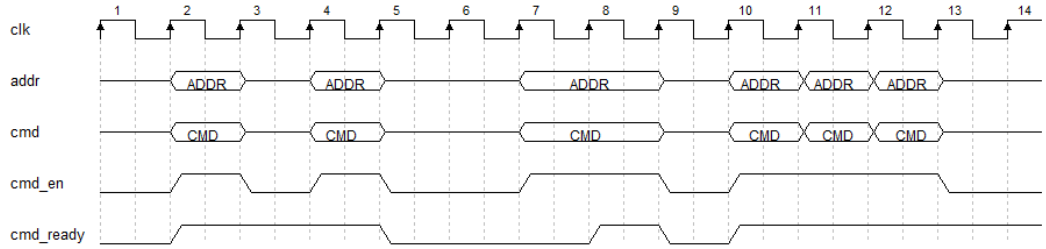
图 3-5 命令、地址与使能信号时序图
