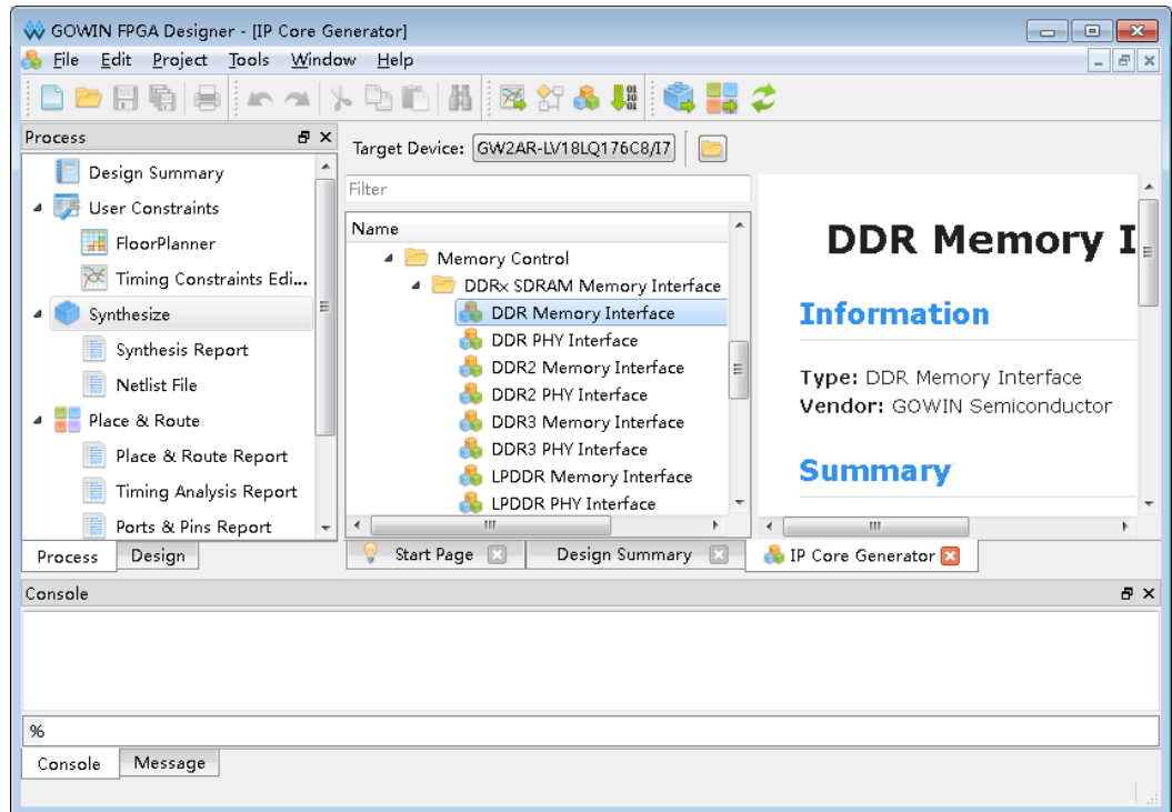
图 6-2 打开 DDR Memory Interface IP 核
