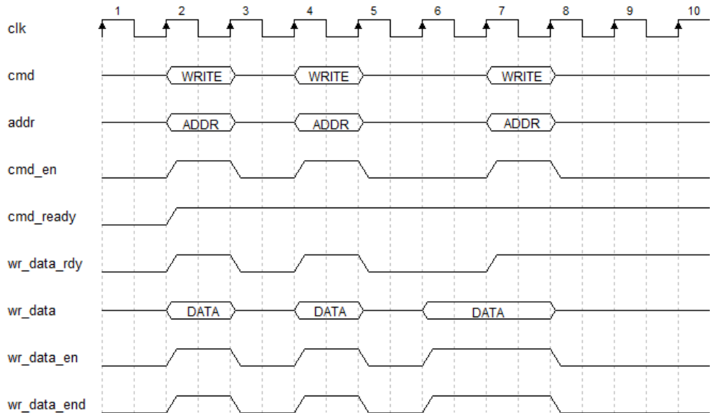
图 3-6 写数据端口时序图
