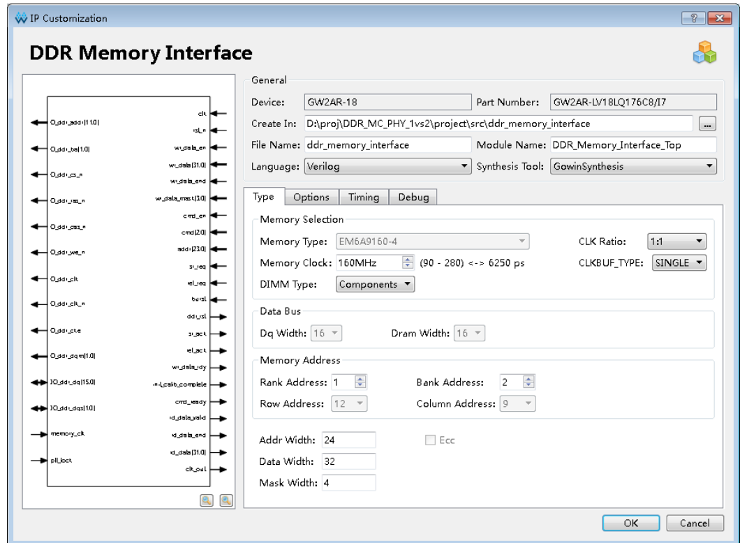
图 6-3 IP 核接口示意图
