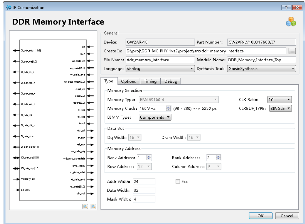
图 6-5 Type 选项卡
