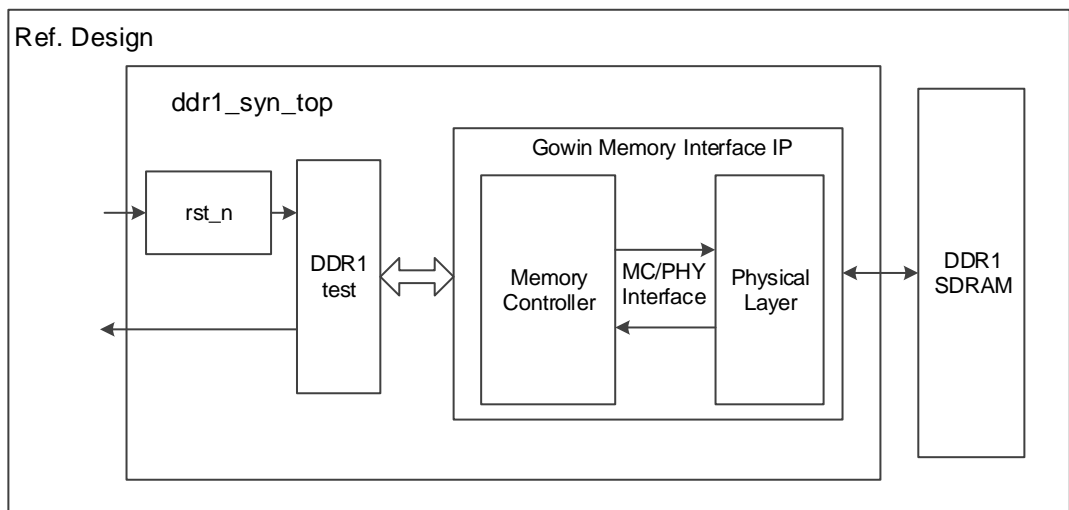
图 7-1 参考设计基本结构框图
