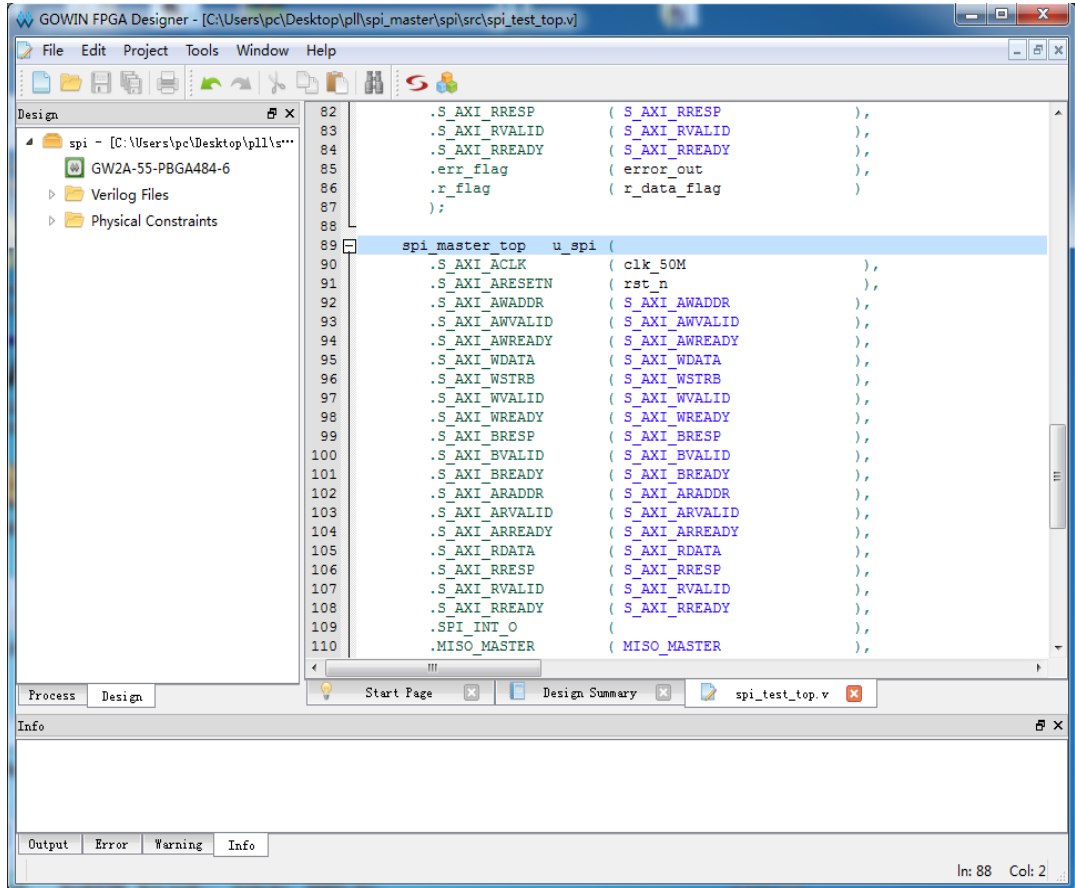
图 6-2 例化 Gowin SPI Master IP
