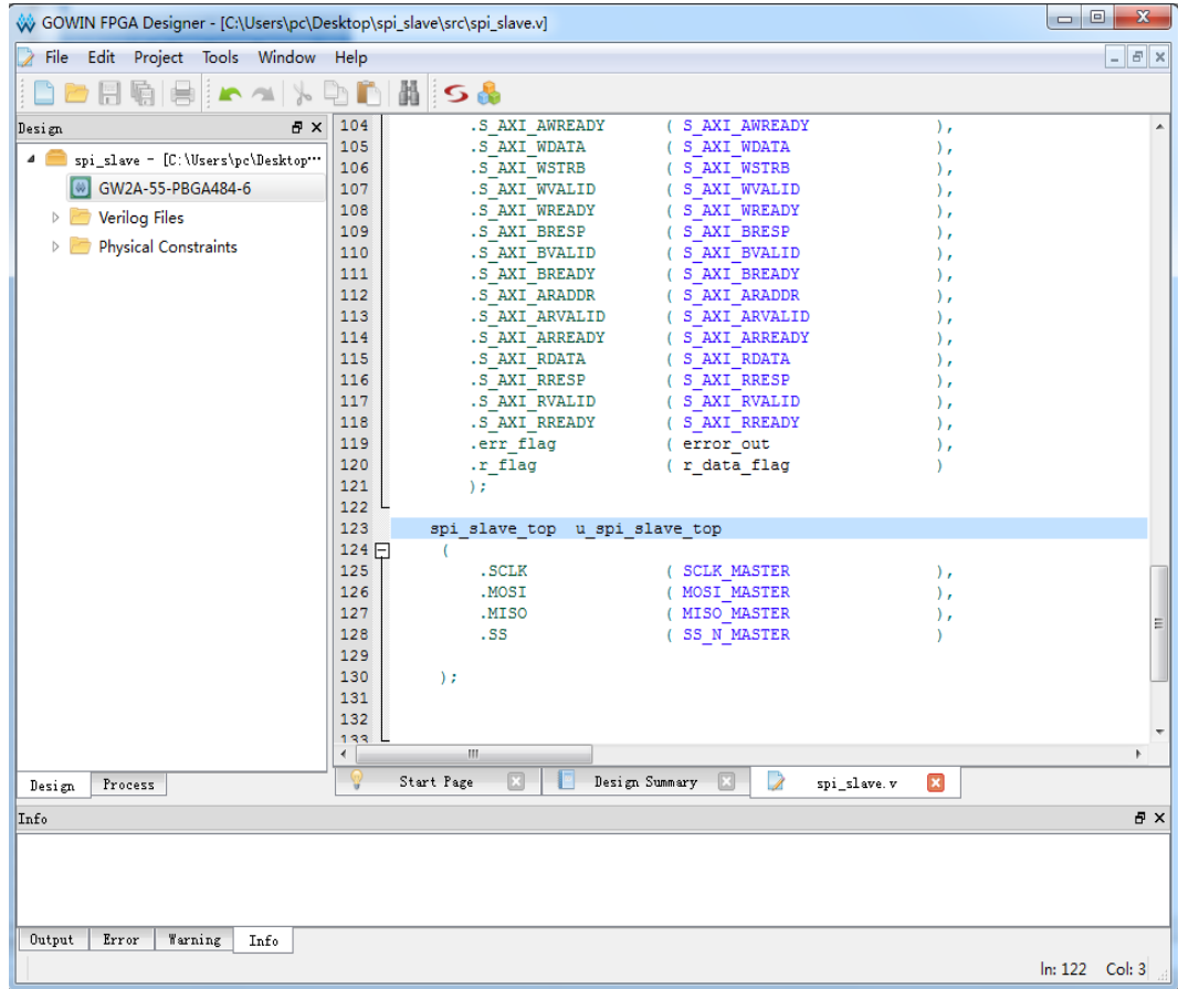
图 6-3 例化 Gowin SPI Slave IP
