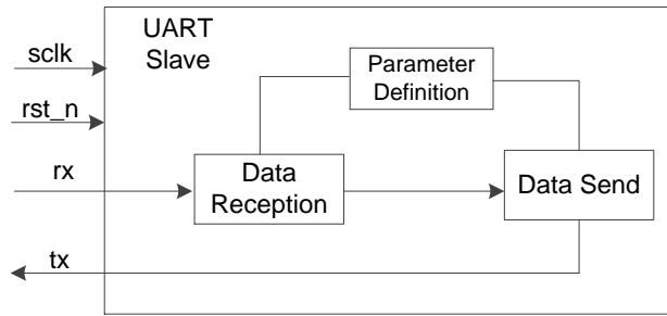
图 4-10 UART Slave 实现框图
