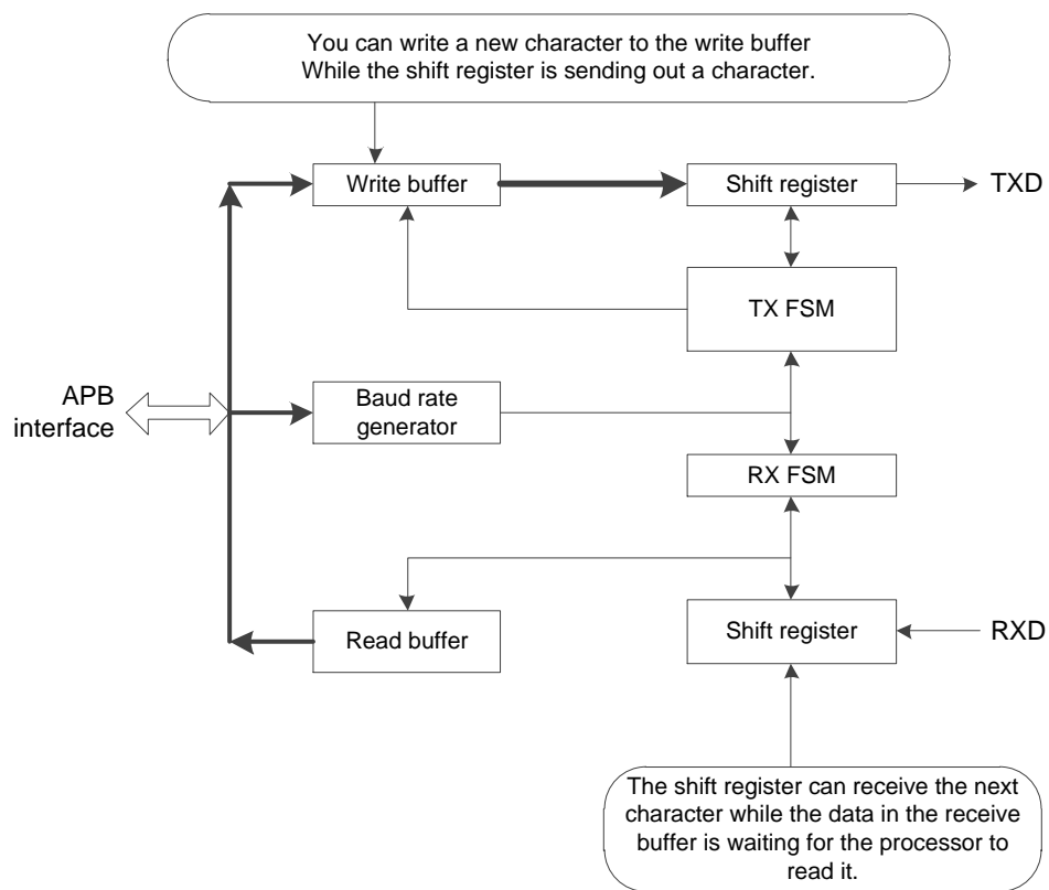
图 4-1 UART Buffering
