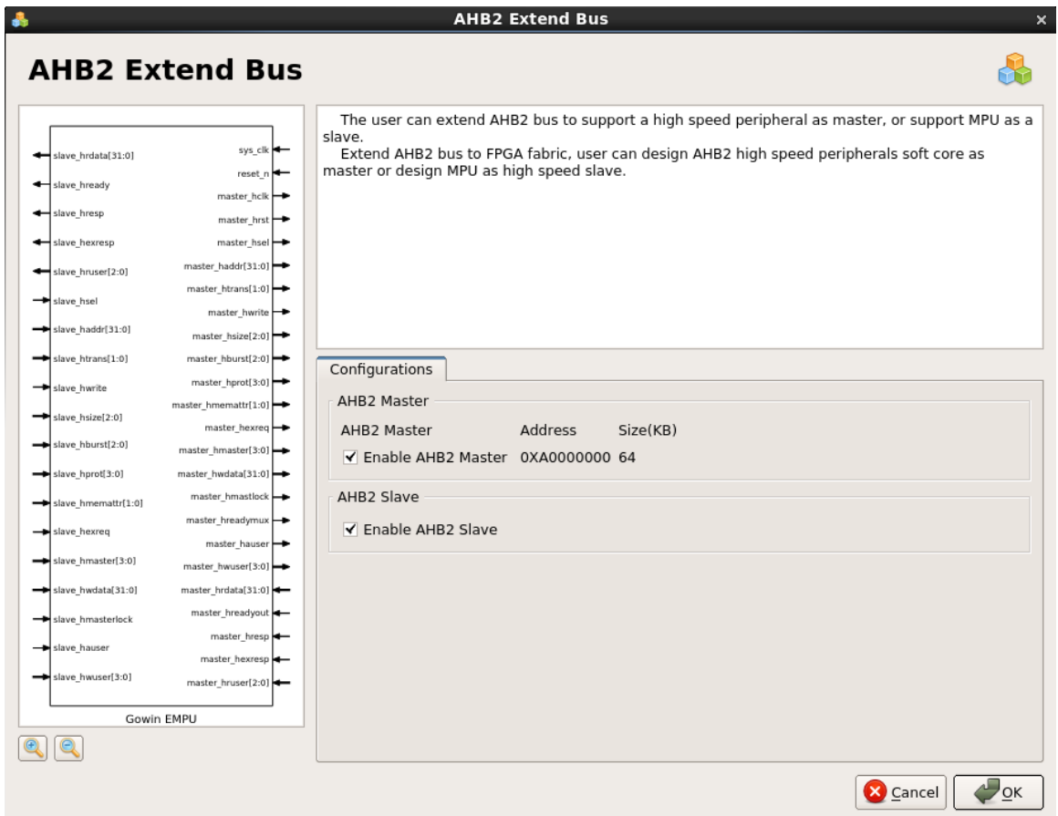
图 3-11 配置 AHB2 Extend Bus
