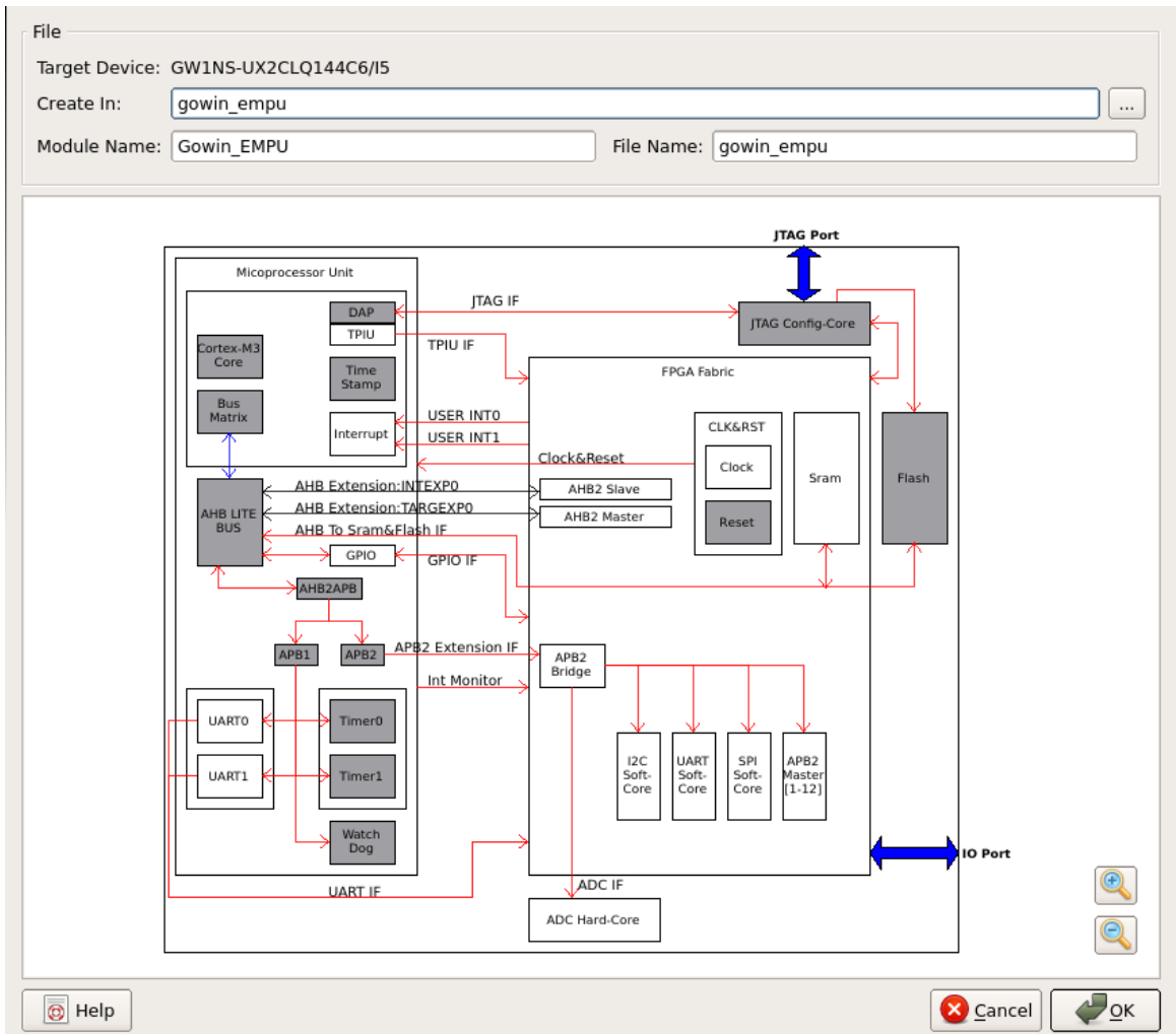
图 3-6 Gowin_EMPU (GW1NS-2C)
