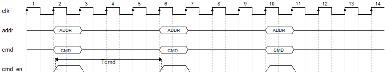
图 4-6 命令、地址与使能信号时序图
