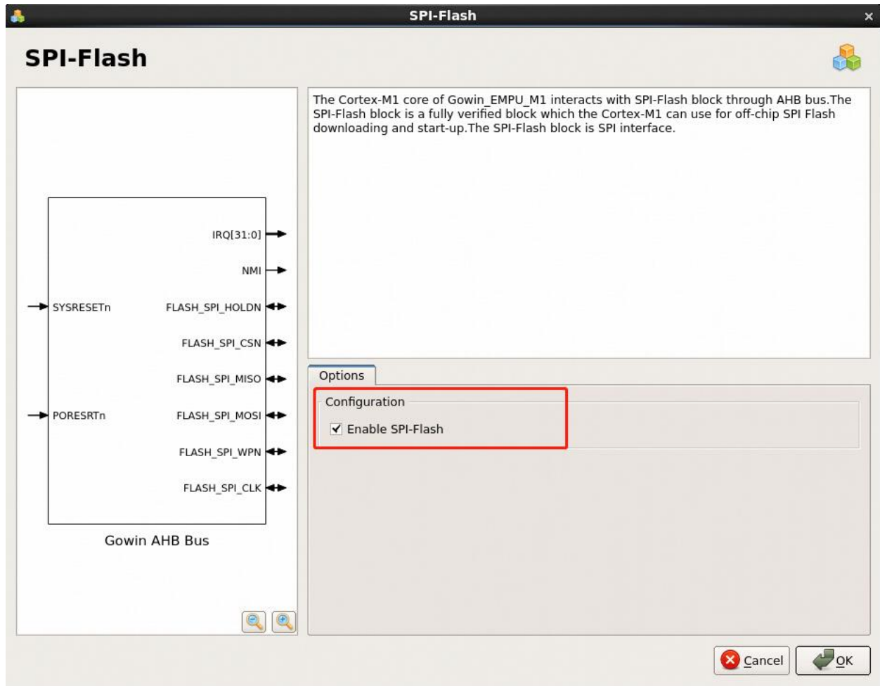
图 3-15 SPI-Flash 配置
