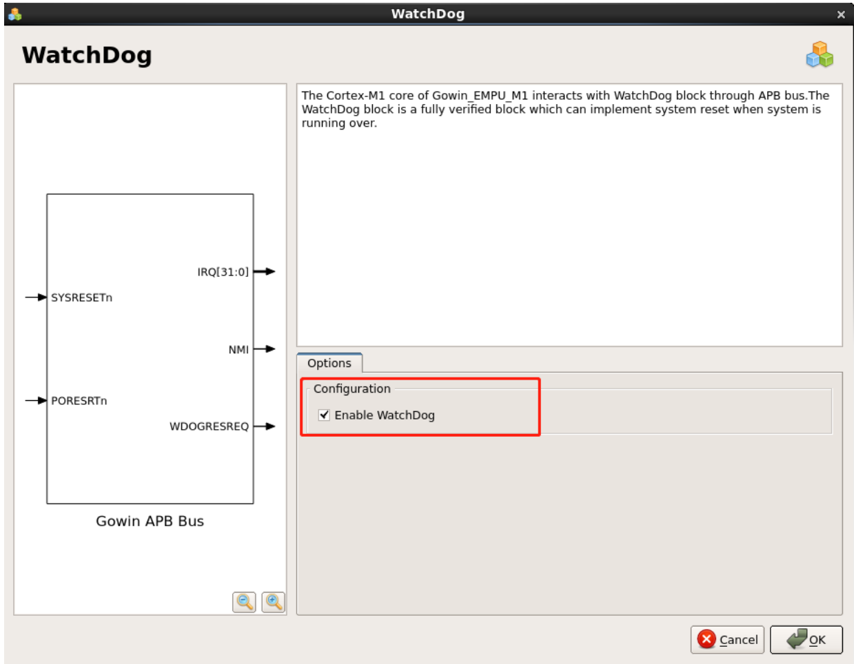
图 3-19 WatchDog 配置
