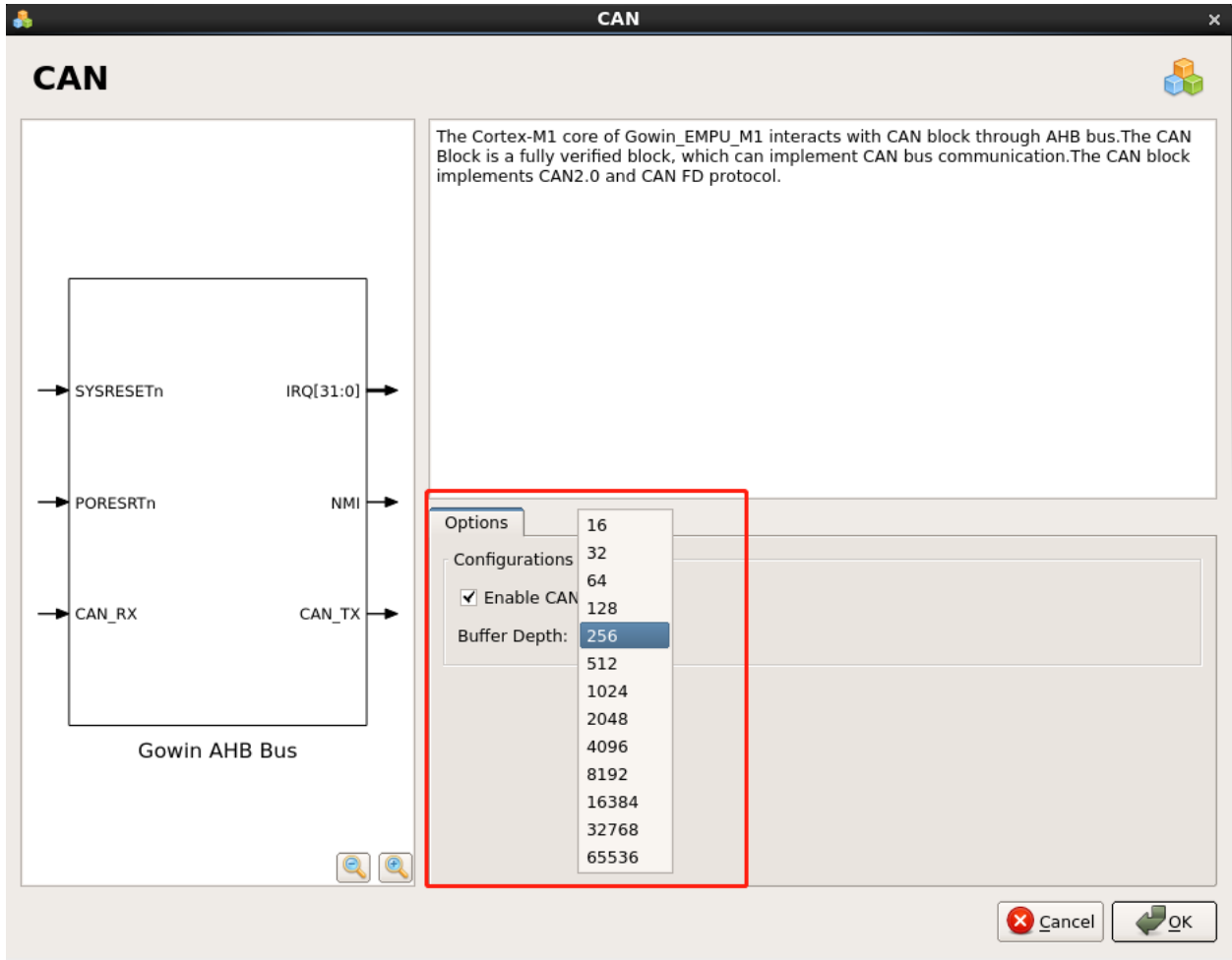
图 3-12 CAN 配置
