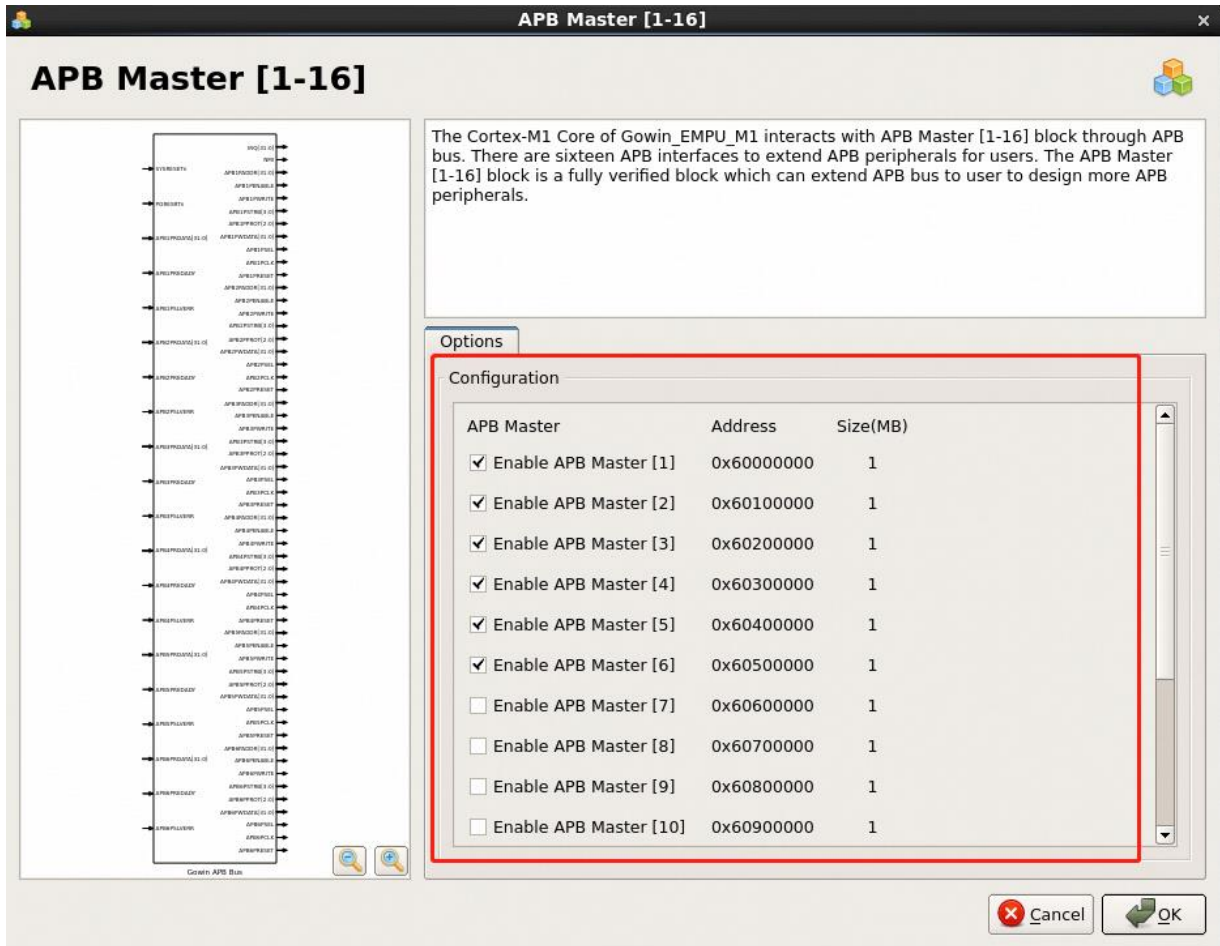
图 3-26 APB Master [1-16]配置
