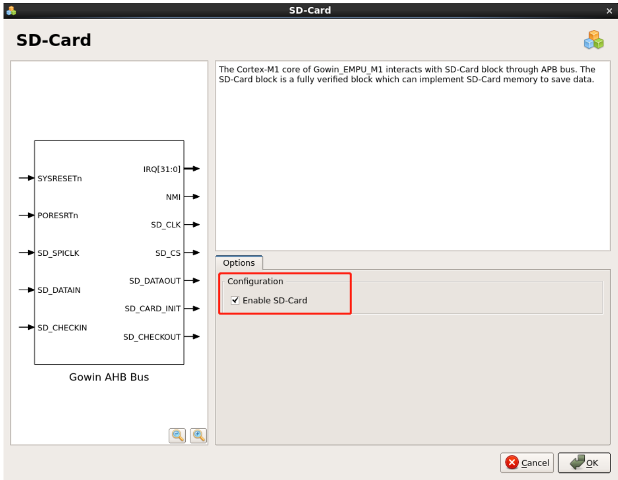
图 3-25 SD-Card 配置
