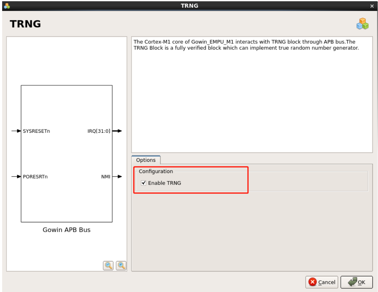
图 3-22 TRNG 配置
