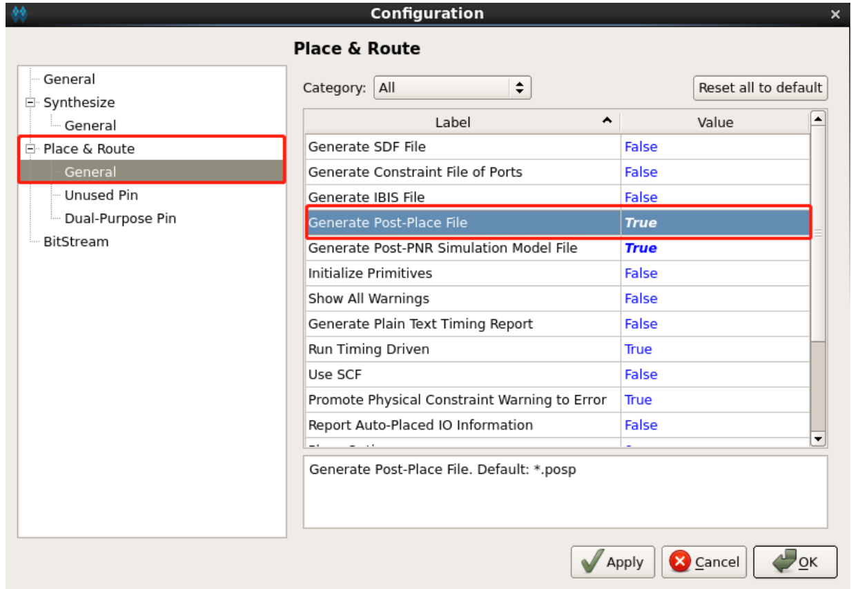
图 3-30 Post-Place File 配置
