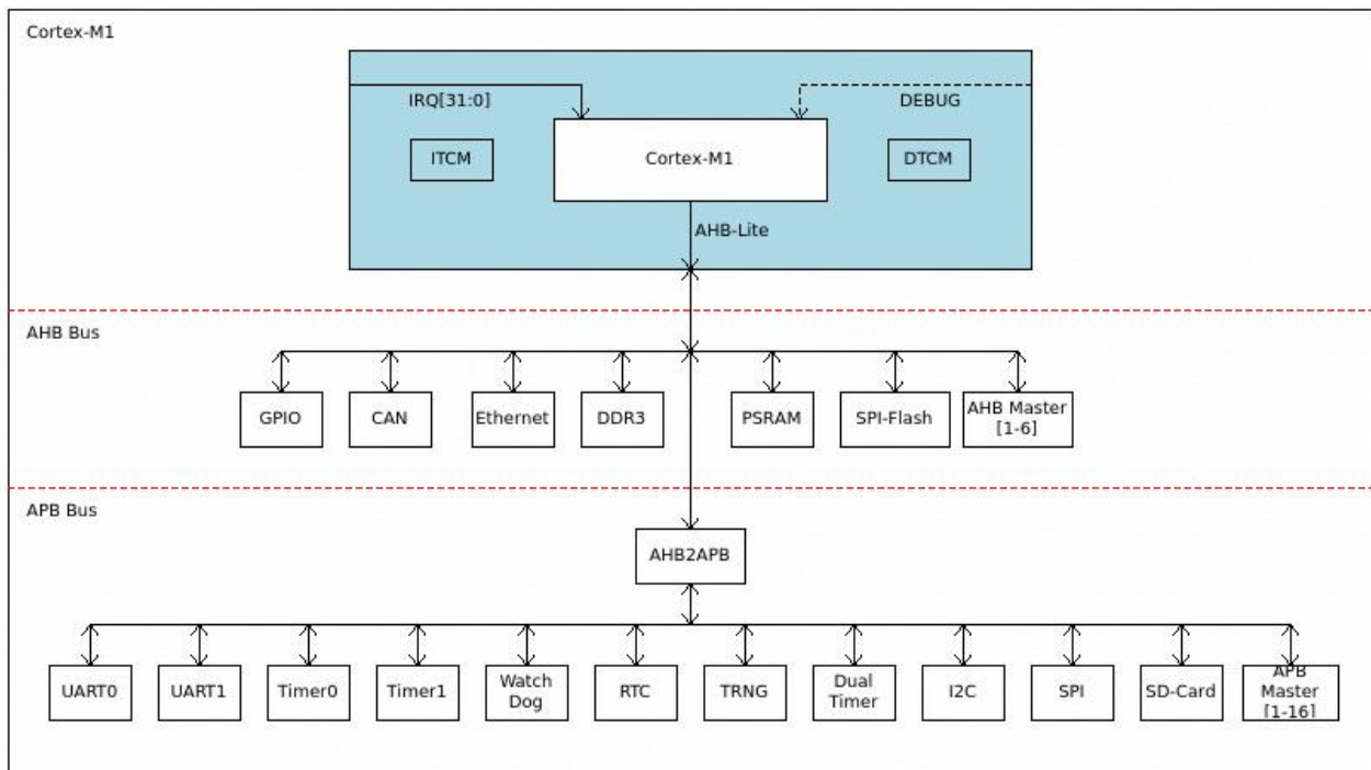
图 1-1 系统架构
