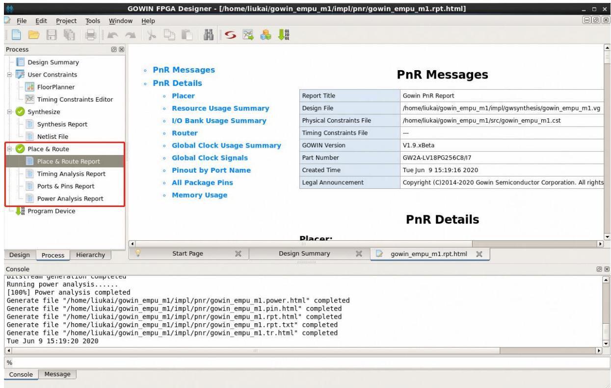
图 3-33 布局布线
