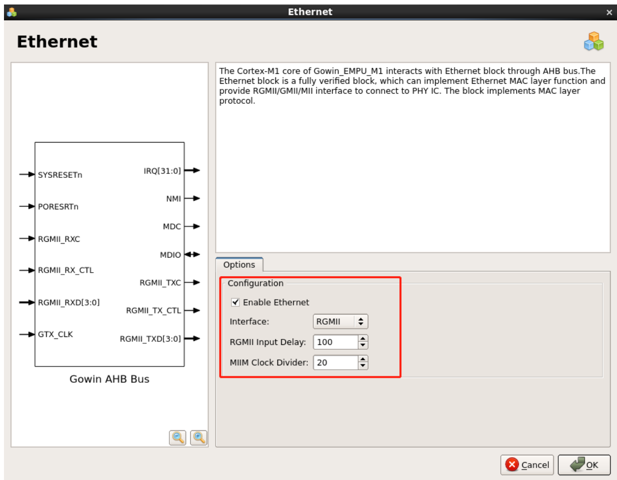
图 3-13 Ethernet 配置
