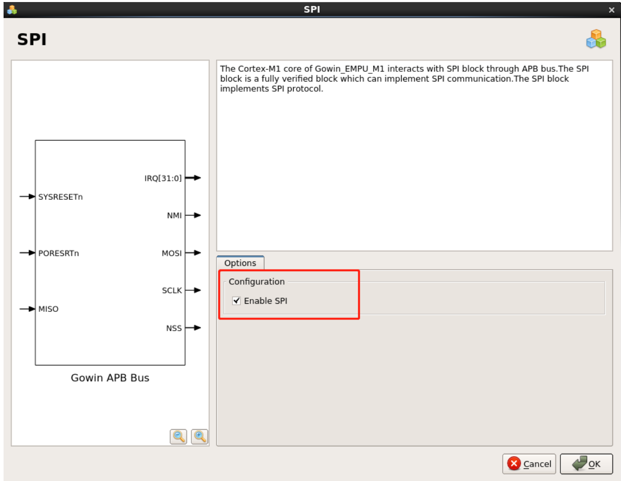
图 3-24 SPI 配置
