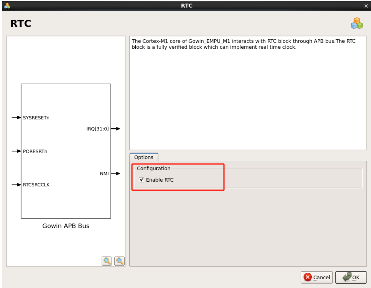
图 3-20 RTC 配置
