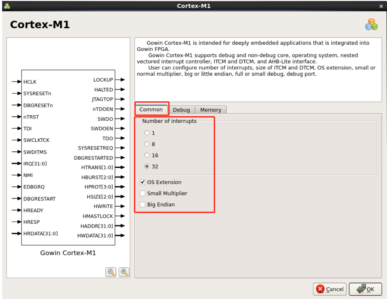
图 3-8 Cortex-M1 通用配置
