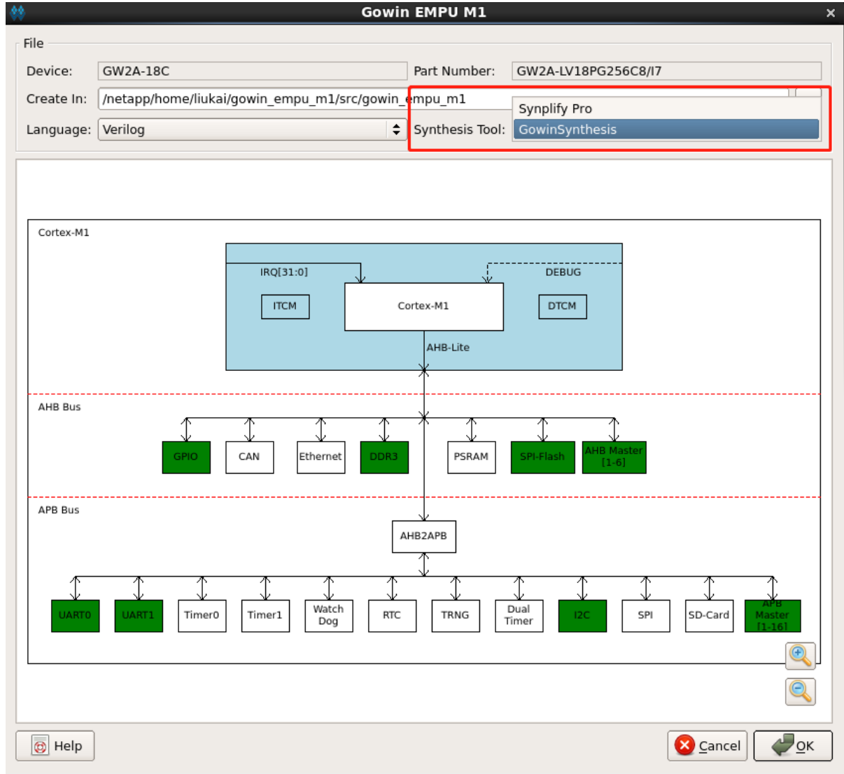
图 3-28 综合工具配置
