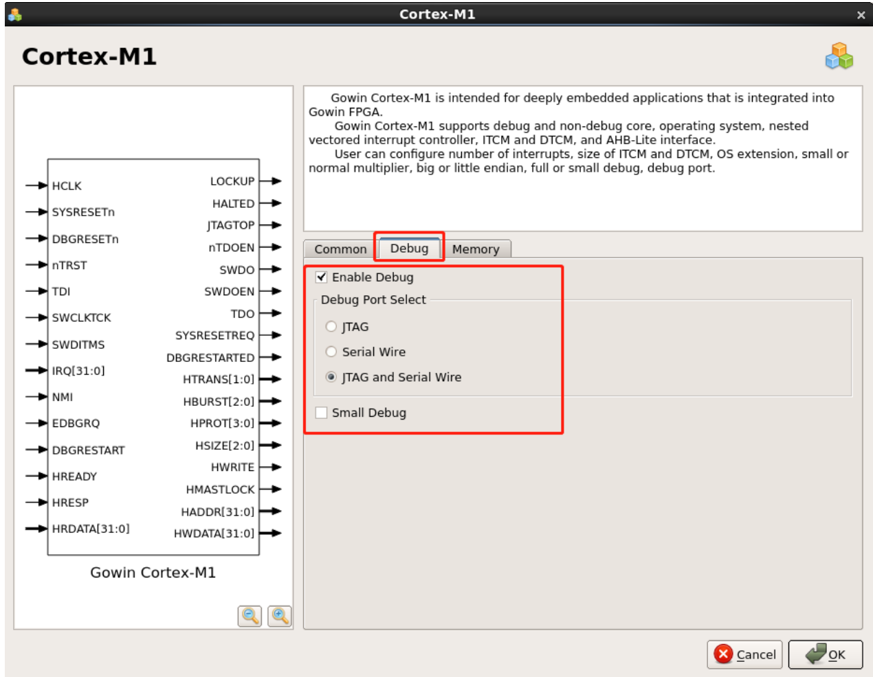
图 3-9 Cortex-M1 调试配置
