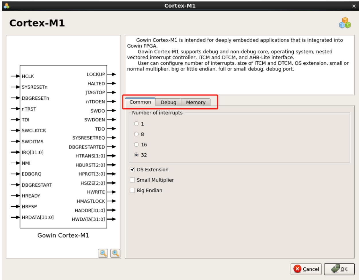
图 3-7 Cortex-M1 配置选项
