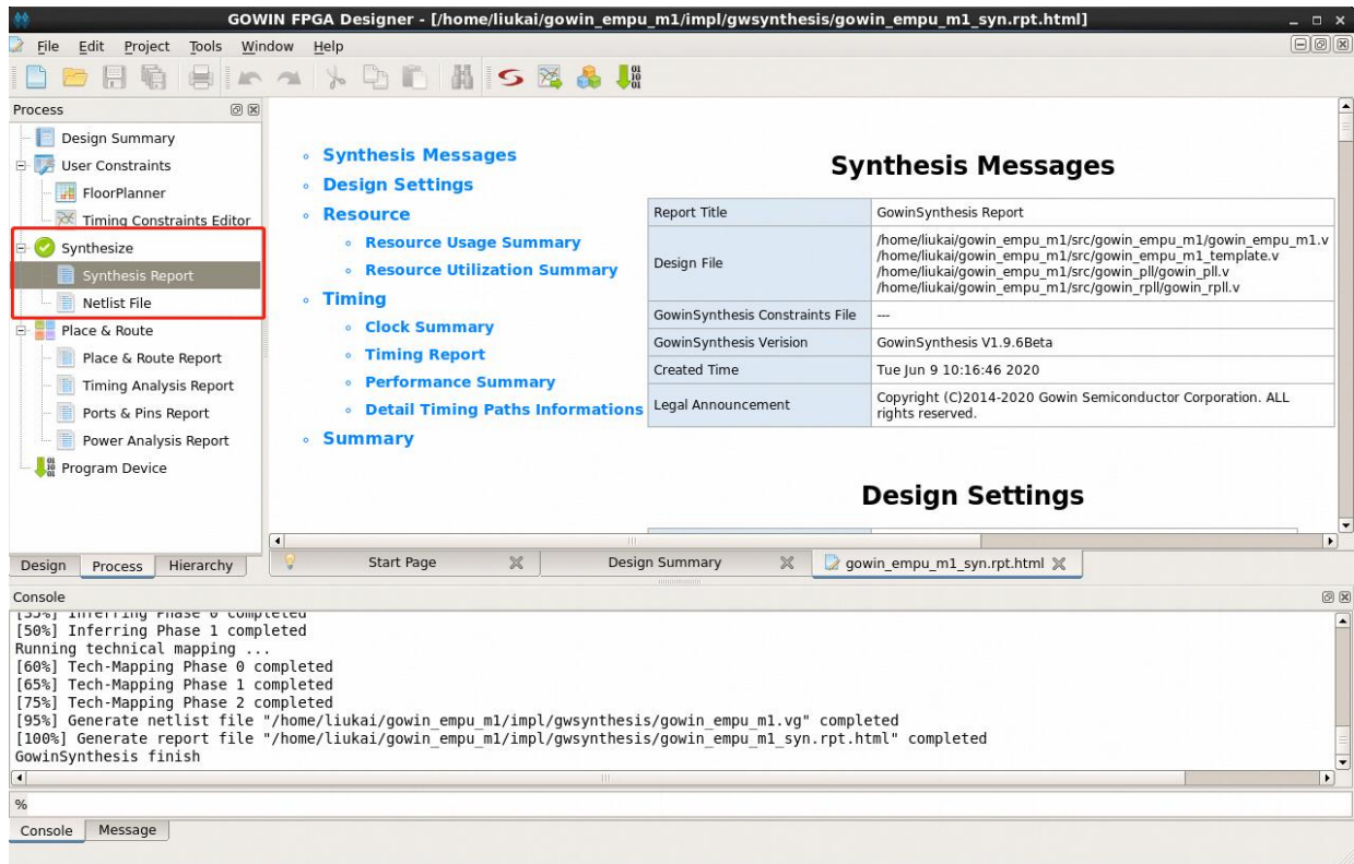
图 3-32 综合
