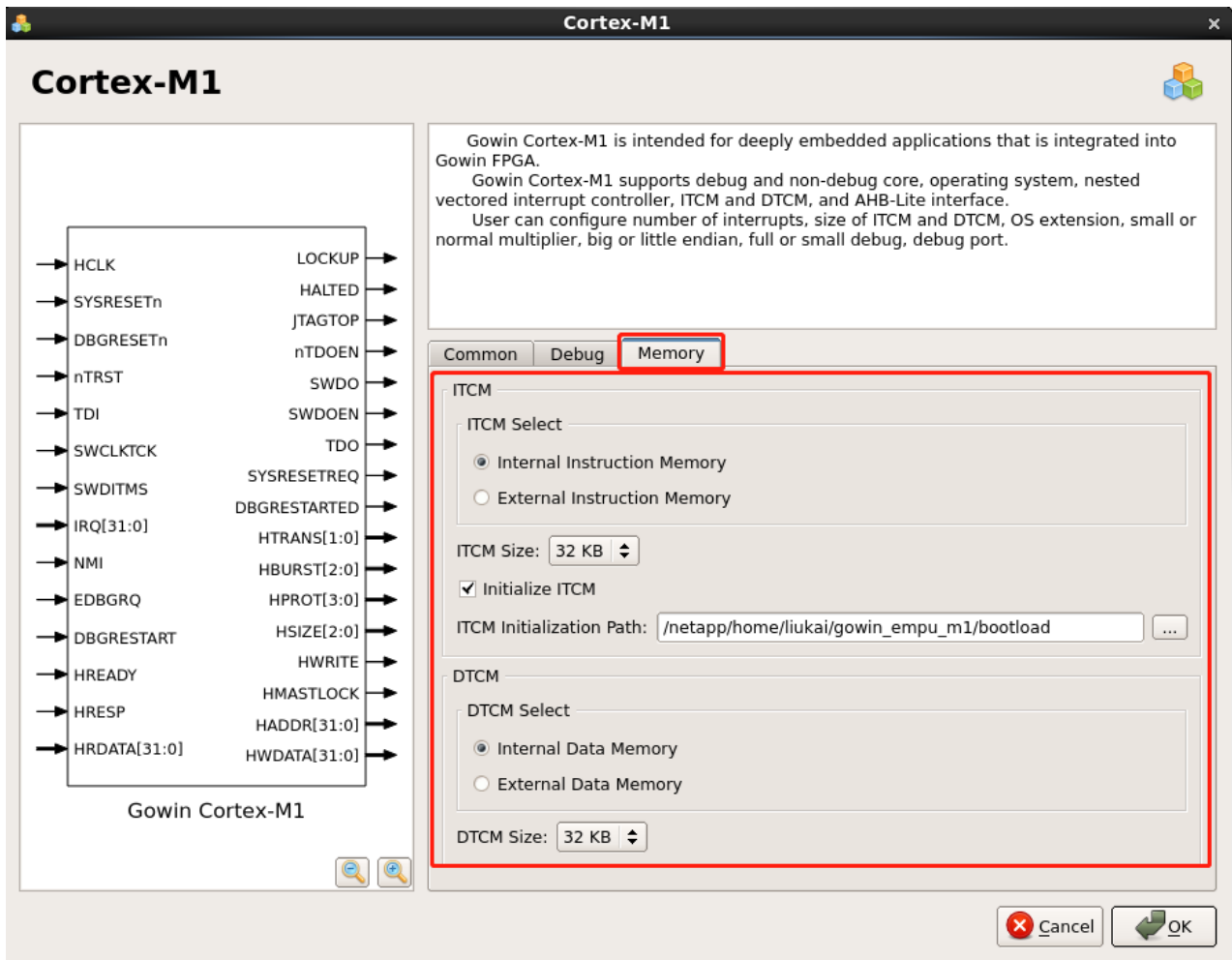
图 3-10 Cortex-M1 存储配置
