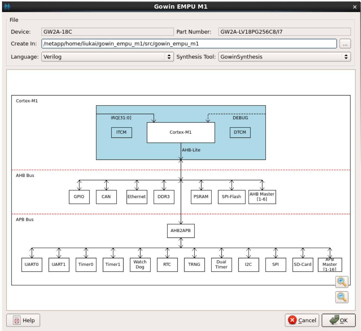
图 3-6 系统配置
