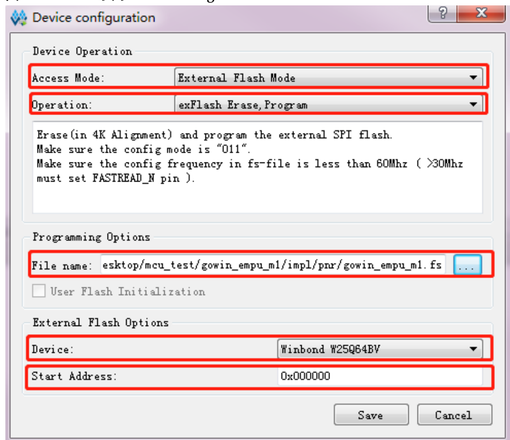
图 3-35 GW2A 系列 Device configuration
