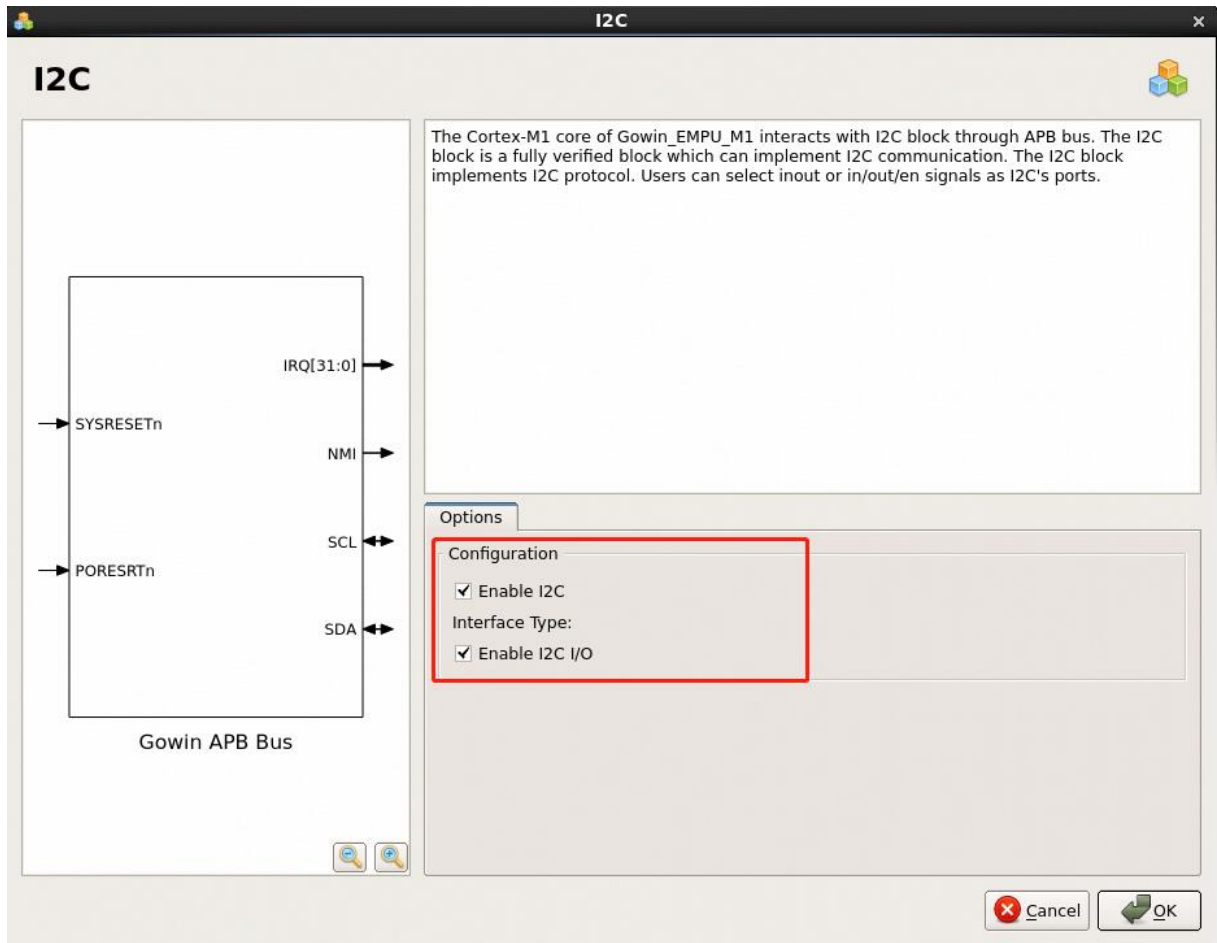
图 3-23 I 2 C 配置
