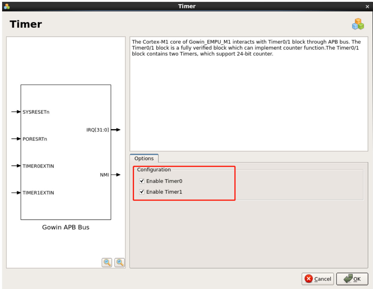
图 3-18 Timer 配置
