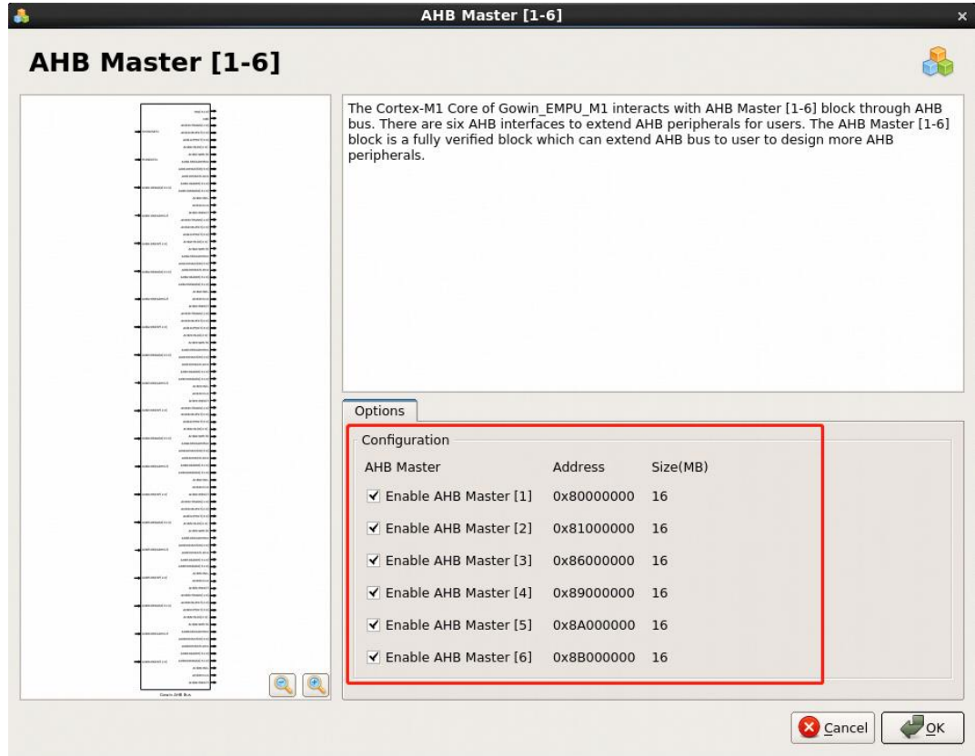
图 3-16 AHB Master [1-6]配置
