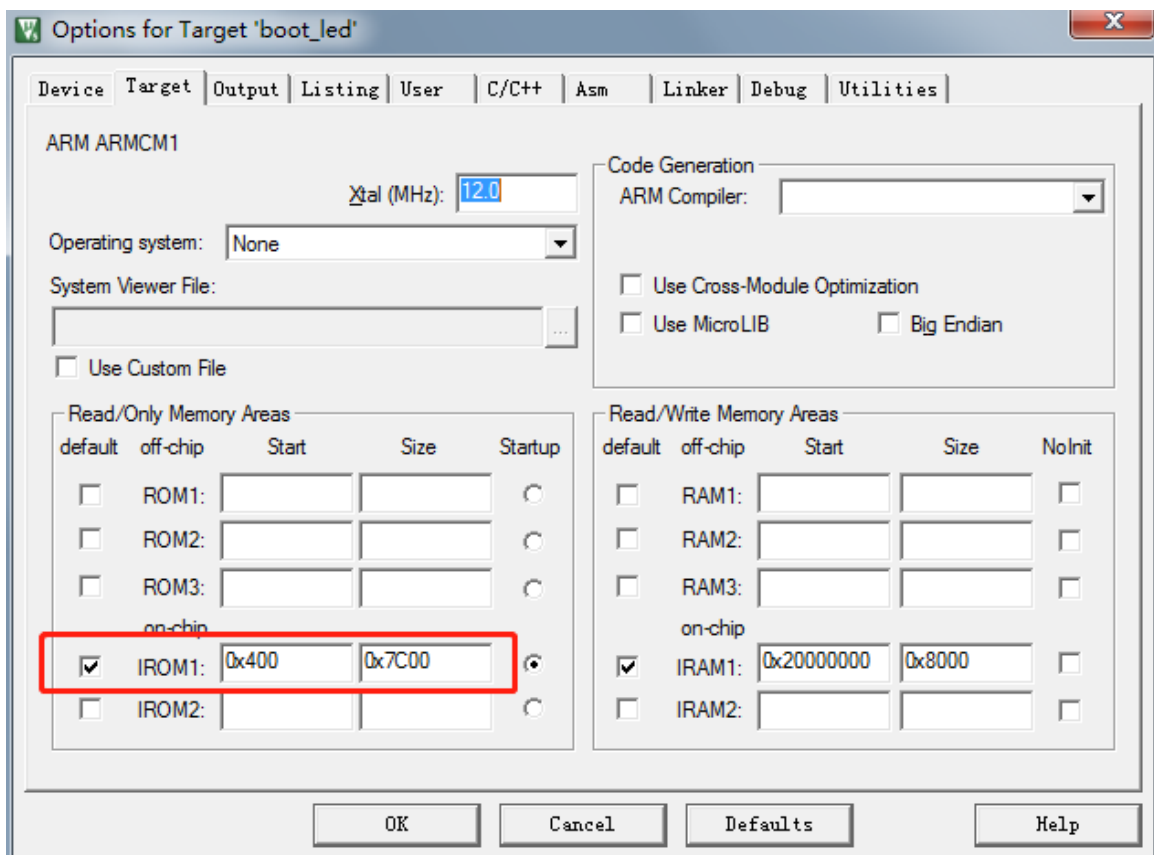
图 4-1 ROM 起始地址和容量配置
