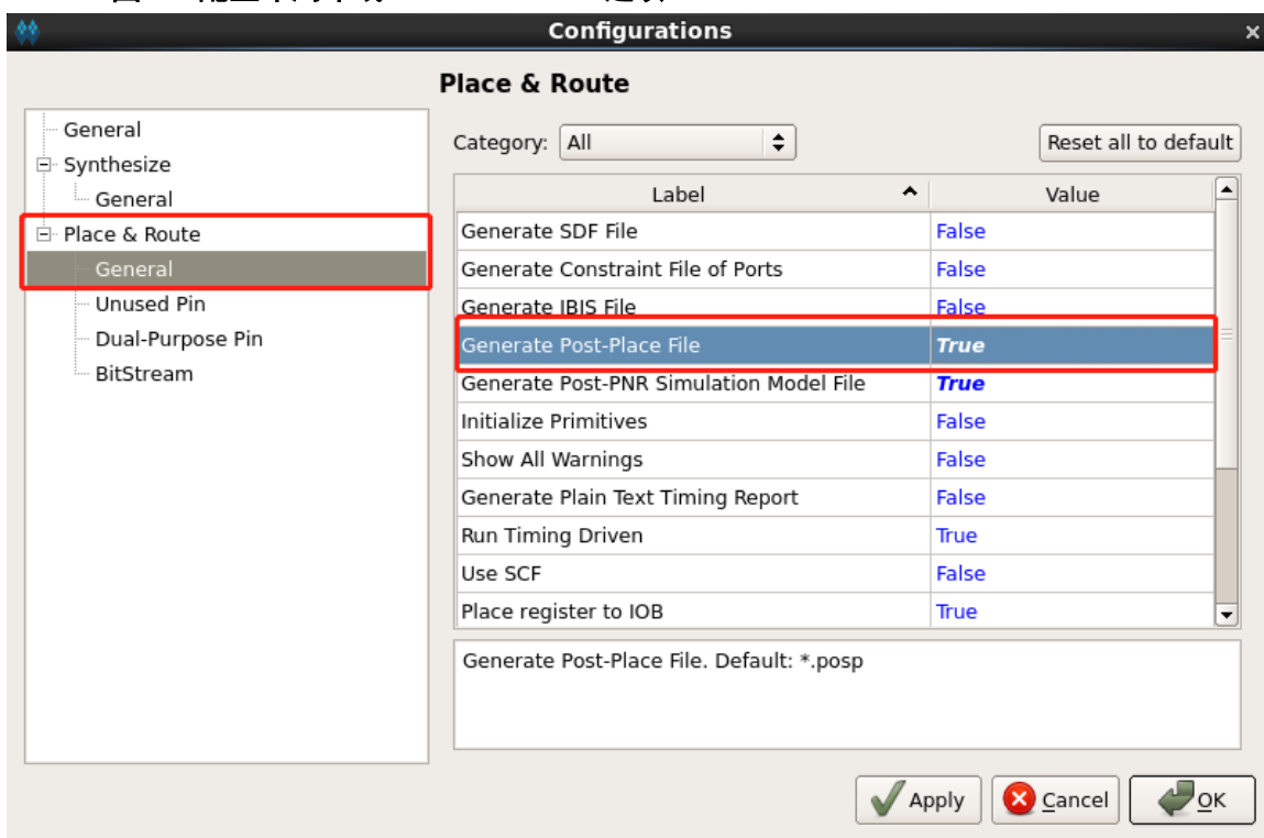
图 3-1 配置布局布线 Post-Place File 选项
